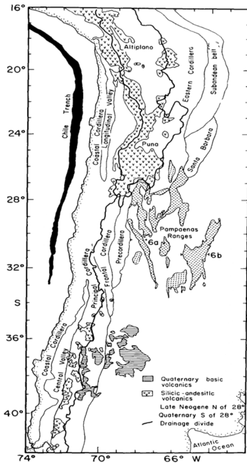
Figure II.7 : Carte des provinces tectoniques et localisation des séries volcaniques récentes des Andes centrales entre la Bolivie, le Chili et l'Argentine (latitudes 16°S et 40°S). Cette carte illustre également le partage des eaux contrôlé par les hauts plateaux de l'Altiplano-Puna (trait noir gras). La limite pacifique correspond à la ligne de crête andine de la frontière ouest des hauts plateaux, tandis que la limite Atlantique correspond à la bordure est des hauts plateaux (d'après Jordan et al., 1983)
