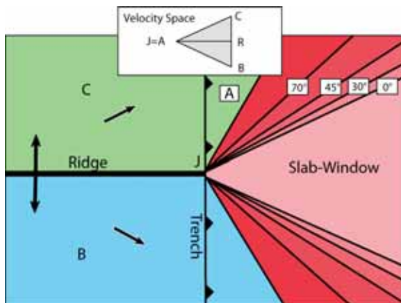
Figure I.5: Effets de l'angle de subduction sur la géométrie en surface de la fenêtre. Projection en surface des bordures de la fenêtre pour des angles de 0 à 70°. Plus l'angle est important, plus la géométrie de la fenêtre est modifiée (Thorkelson, 1996).
