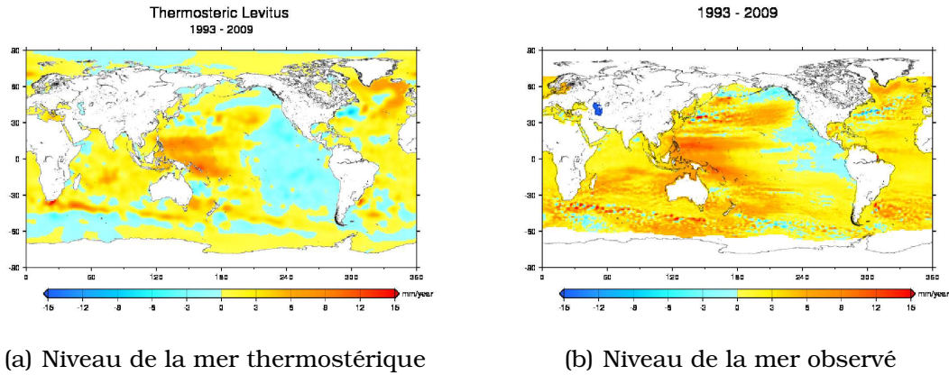
FIG. 5.3 – Cartographie régionale du niveau de la mer (a) thermostérique (jusqu'à 700m, Levitus et al. [2009]) et (b) observé par altimétrie spatiale entre 1993 et 2009
