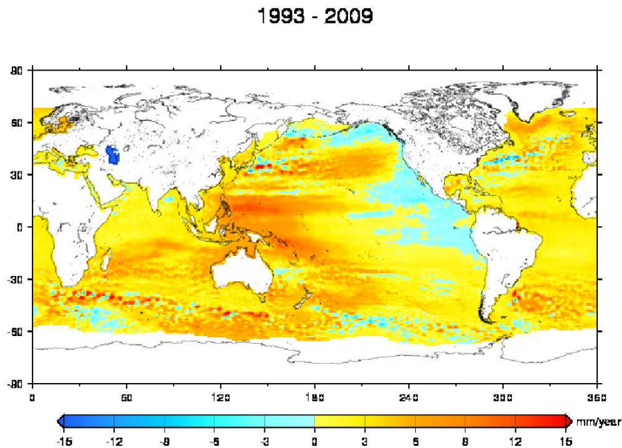
FIG. 5.1 – Distribution géographique des taux de variation du niveau de la mer entre janvier 1993 et novembre 2009 (source CLS-LEGOS).
