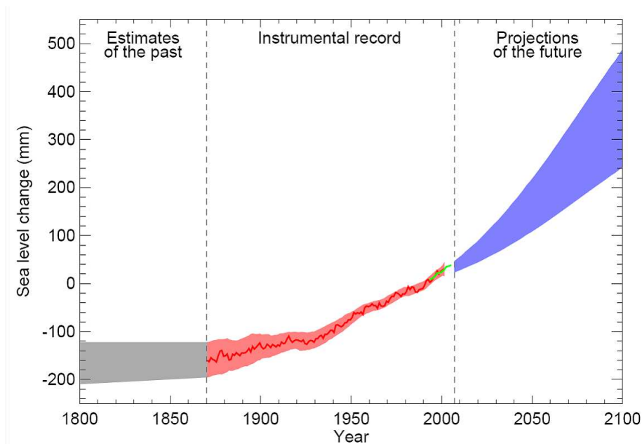
FIG. 2.9 – Evolution du niveau moyen global de la mer entre 1800 et 2100 (IPCC, 2007). La courbe grise représente les estimations faites à partir des études géologiques. La courbe rouge représente le niveau de la mer observé par les marégraphes ( Church et al. [2004]). La courbe verte représente le niveau moyen global observé par altimétrie spatiale. Enfin, l'enveloppe bleue représente les estimations basées sur les modèles numériques climatiques de l'IPCC (2007).
