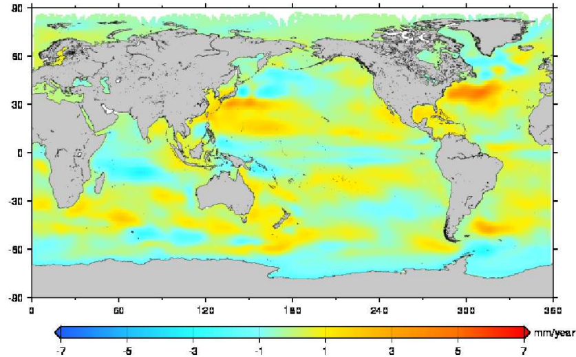
FIG. 5.7 – Cartographie des taux de variation du niveau de la mer entre 1960 et 2003 basée sur les données du modèle numérique OPA/NEMO.
