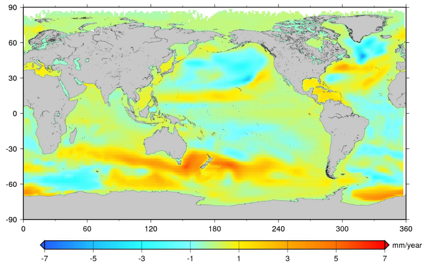
FIG. 5.14 – Cartographie des tendances du niveau de la mer thermostérique (tendance uniforme retirée) entre 1950 et 2000 basée sur les données du modèle couplé CNRM-CM3 (Salas-Melia et al. [2005]) de la simulation du XX ème siècle.
