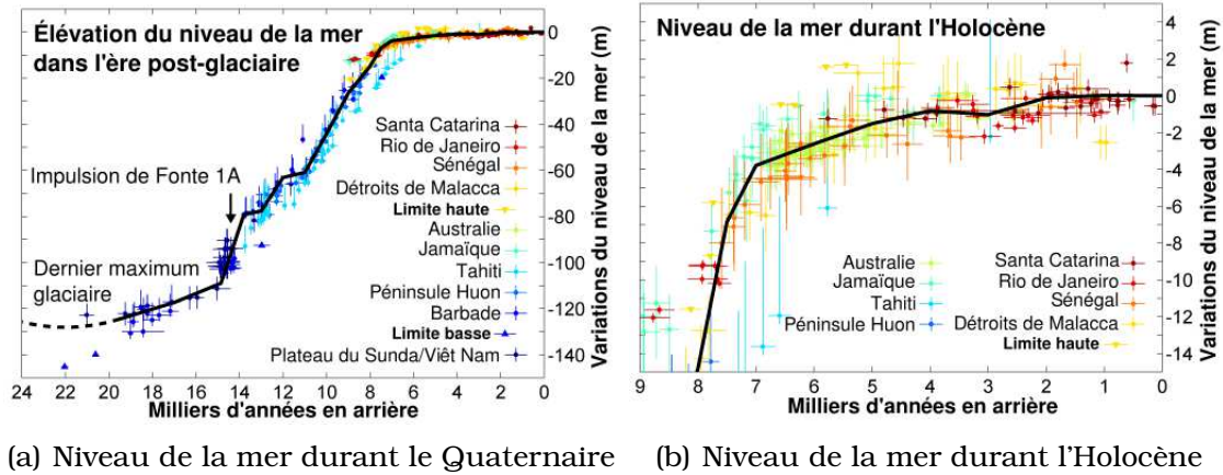
FIG. 2.3 – Estimations des variations du niveau de la mer durant le Quaternaire et l'Holocène basées sur des études sédimentaires ( Fleming et al. [1998]; Milne et al. [2005])
