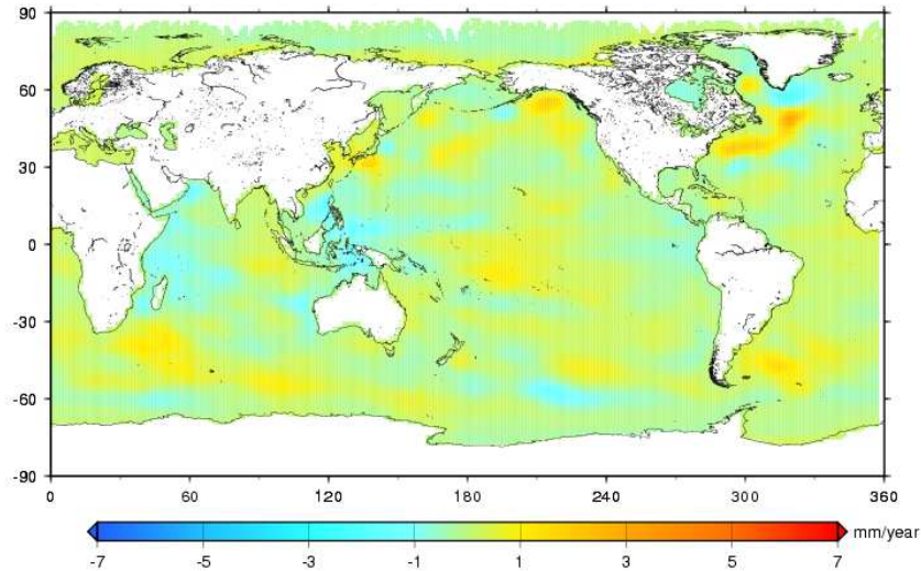
FIG. 5.9 – Cartographie des taux de variation du niveau de la mer reconstruit entre 1950 et 2003 en retirant l'EOF0 lors du calcul de reconstruction.
