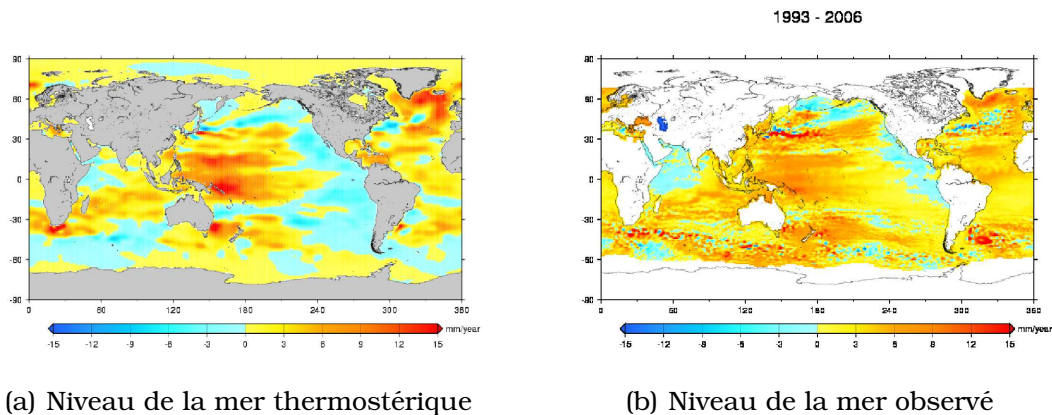
FIG. 5.4 – Cartographie régionale du niveau de la mer (a) thermostérique (jusqu'à 700m, Ishii and Kimoto [2009]) et (b) observé par altimétrie spatiale entre 1993 et 2006.
