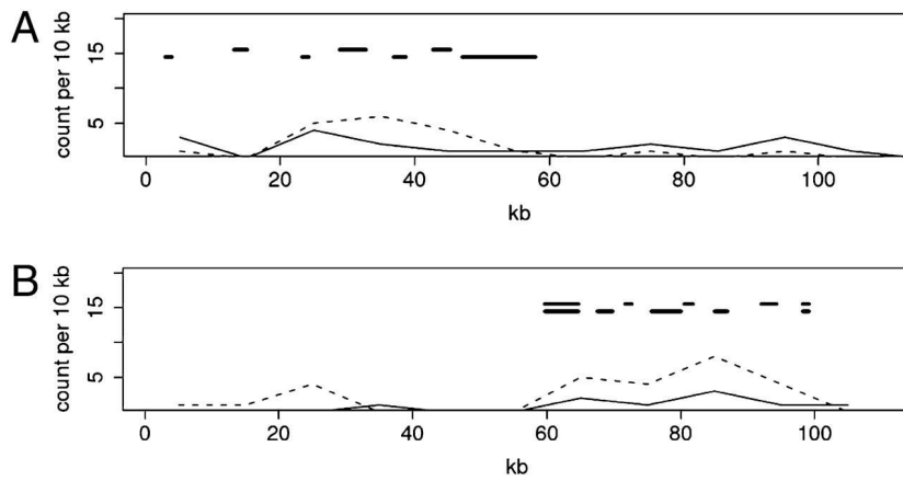
FIG. 6: Corrélation entre les points de rupture de synténie et la densité en ET chez des Lépidoptères. A. region CYP4M de S. frugiperda . B. région EcR de H. armigera . Les lignes pointillées correspondent à la densité en ET, les lignes pleines fines à la densité en gènes, et les lignes pleines épaisses aux points de rupture de synténie. (Tiré de d'Alençon et coll. 2010. )
