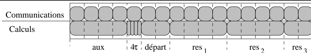
FIG. 6.9 - L'ordonnancement
