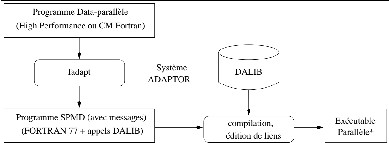
FIG. 4.3 - Aperçu d'ADAPTOR
