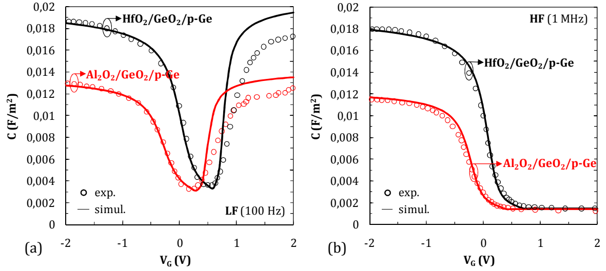
Figure 2.12 : Caractéristiques C - V expérimentales (ronds) [Delabie] et simulées [Moreau3] (Poisson-Schrödinger) de deux capacités HfO_2/GeO_2/p-Ge (noir) et Al_2O_3/GeO_2/p-Ge (rouge) (a) à basse fréquence (100 Hz) et (b) à haute fréquence (1 MHz) (où les paramètres de simulation sont: T_{HfO_2} = T_{Al_2O_3} = 4.0 nm, T_{GeO_2} = 1.4 nm, N_A = 1 \times 10^{17} cm^{-3} ).
