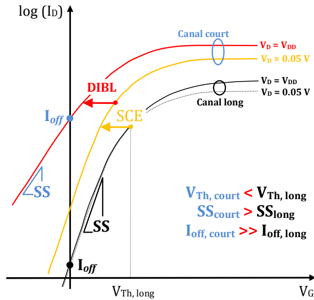
Figure 1.4 : Caractéristiques I_D(V_G) schématisques de transistors MOSFET à canal long et canal court sous faible et forte polarisation de drain. La figure met en évidence la dégradation des paramètres sous le seuil due aux effets de canal court SCE et DIBL.
