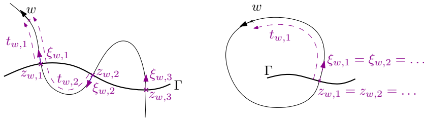
FIGURE 6.5 – Les conditions initiales (z_{w,k}, \xi_{w,k}) \in N_E\Gamma_0 qui atteignent w en temps t_{w,k} positif.
