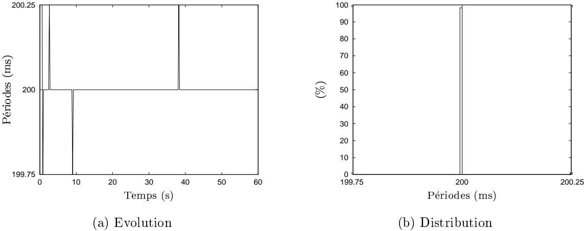
Figure 3.31 – Simulation : évolution des périodes en sortie d'un régulateur (cas Béziens)
