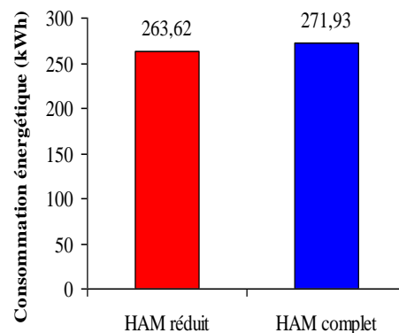
Figure 4.7b : Consommations énergétiques.
