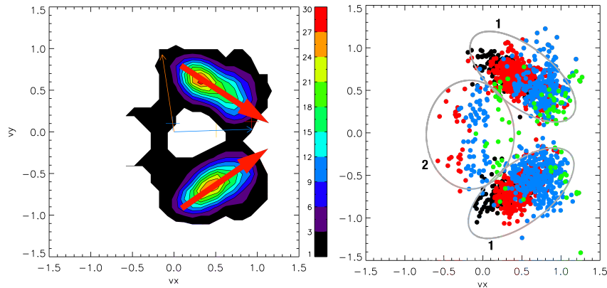
FIGURE 2.19: A gauche, la distribution \mathbf{e} mesurée au centre du jet (déjà représentée sur la figure 2.14). Les flèches rouges représentent le transfert de v_y vers v_x qu'une particule fait lorsqu'elle subit les rebonds sur la séparatrice. A droite, les particules de cette même distribution, colorées en fonction du nombre de rebonds effectués : noir - 0 rebond, rouge - 1 rebond, bleu - 2 rebonds, vert - 3 rebonds. Les cercles gris numérotés 1 encerclent les particules faisant en effet ce mouvement. Le cercle numéroté 2 entoure les particules minoritaires ayant une dynamique différente.
