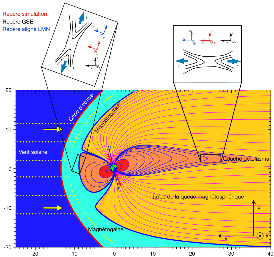
FIGURE 1: Magnétosphère terrestre représentée dans le plan méridien GSE (x, z) . Un schéma de reconnexion est placé à la magnétopause et un autre dans la queue. Pour chaque emplacement, les repères GSE, simulation et local LMN sont représentés.
