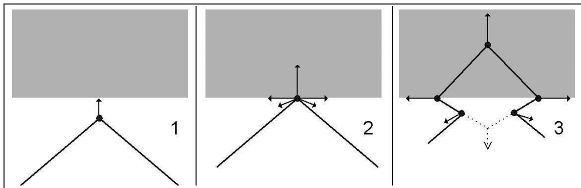
FIG. 4.11: Décomposition selon le principe de Huygens avec un agent entrant en collision avec un milieu plus rapide, (1) avant la collision, (2) l'agent se décompose en cinq, (3) après la décomposition.
