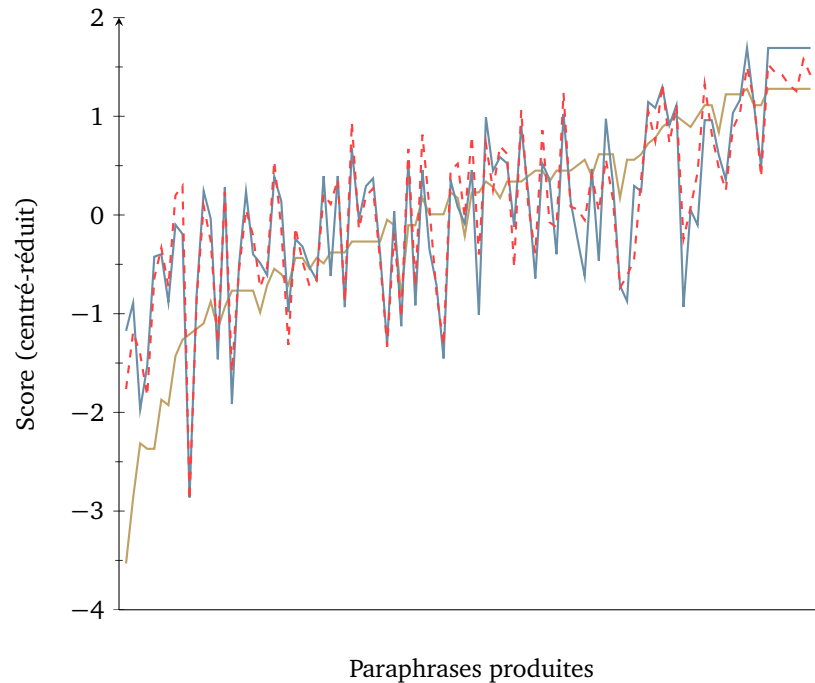
FIGURE 4.5: Comparaison entre les paraphrases et les phrases sources du jeu TEST 2. En beige, l'opposé de la distance d'édition ; la mesure BLEU en bleu ; la mesure NIST en rouge. Les trois mesures suivent la même tendance.
