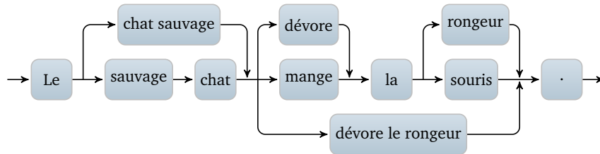
(c) Treillis de production
