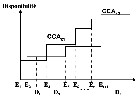
FIGURE 3.14 – Discretisation du temps par événements, cas général
