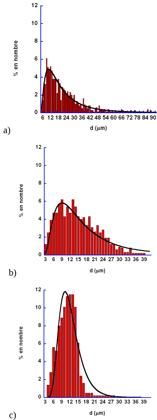
Figure 42 : Distributions en nombre de la taille des gouttes aux temps d'émulsification de l'ETC 91 t = a) 300 ; b) 780 ; c) 2400 s pour une vitesse de rotation du gros barreau \Omega = 90 rpm. Les modèles (courbes noires) sont des lois de distribution log-normale.
