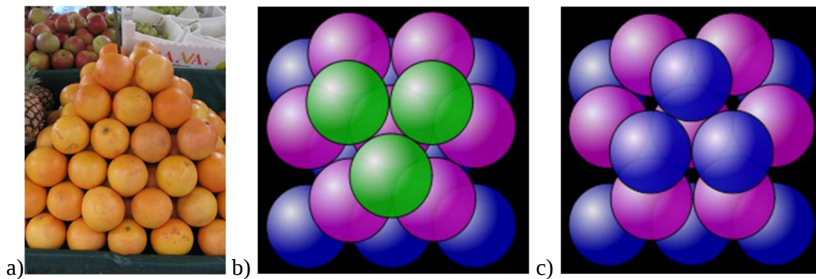
Figure 3 : a) Exemple d'empilement compact utilisé « intuitivement » au quotidien. b) Empilement compact de type cubique face centré (ABC). c) Empilement compact de type hexagonal compact (ABA).
