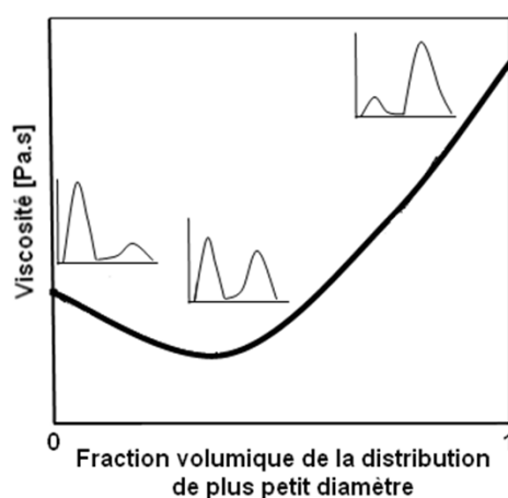
Figure 17 : Représentation de l'évolution de la viscosité d'une ETC bimodale (mesurée à un gradient de vitesse donné) en fonction de la fraction volumique de chacune des distributions [81].
