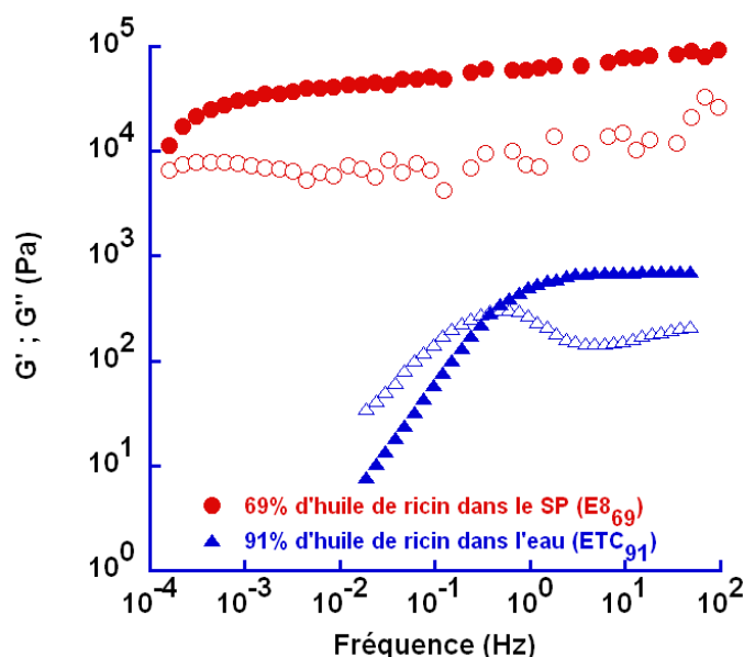
Figure 84 : Evolution des modules visqueux G'' (symboles vides) et élastique (symbole pleins) en fonction de la fréquence pour l'émulsion concentrée E8 69 contenant 69% de phase dispersée (ronds) et pour l'ETC contenant 91% de phase dispersée (triangles). Les valeurs des contraintes, prises dans le domaine linéaire de chaque émulsion, étant de 40 Pa et 5 Pa respectivement
