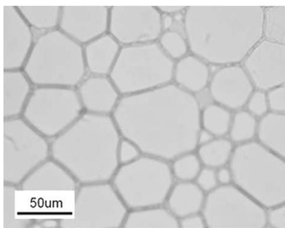
Figure 2 : Photographie au microscope d'une émulsion très concentrée (ETC) contenant 80% de n-nonane dans l'eau [24].
