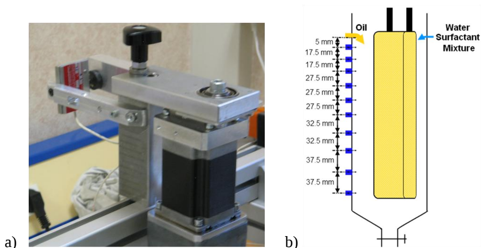
Figure 63 : a) Photographie du moteur entraînant le gros barreau auquel est lié le capteur de force. b) Schéma représentatif d'une vue transversale du MDB-Cont. Mise en évidence des vannes de prélèvement latérales.
