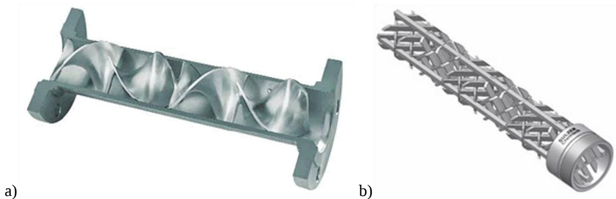
Figure 25 : Exemples de géométrie de mélangeurs statiques : a) de type hélicoïdal ; b) de type grillage.
