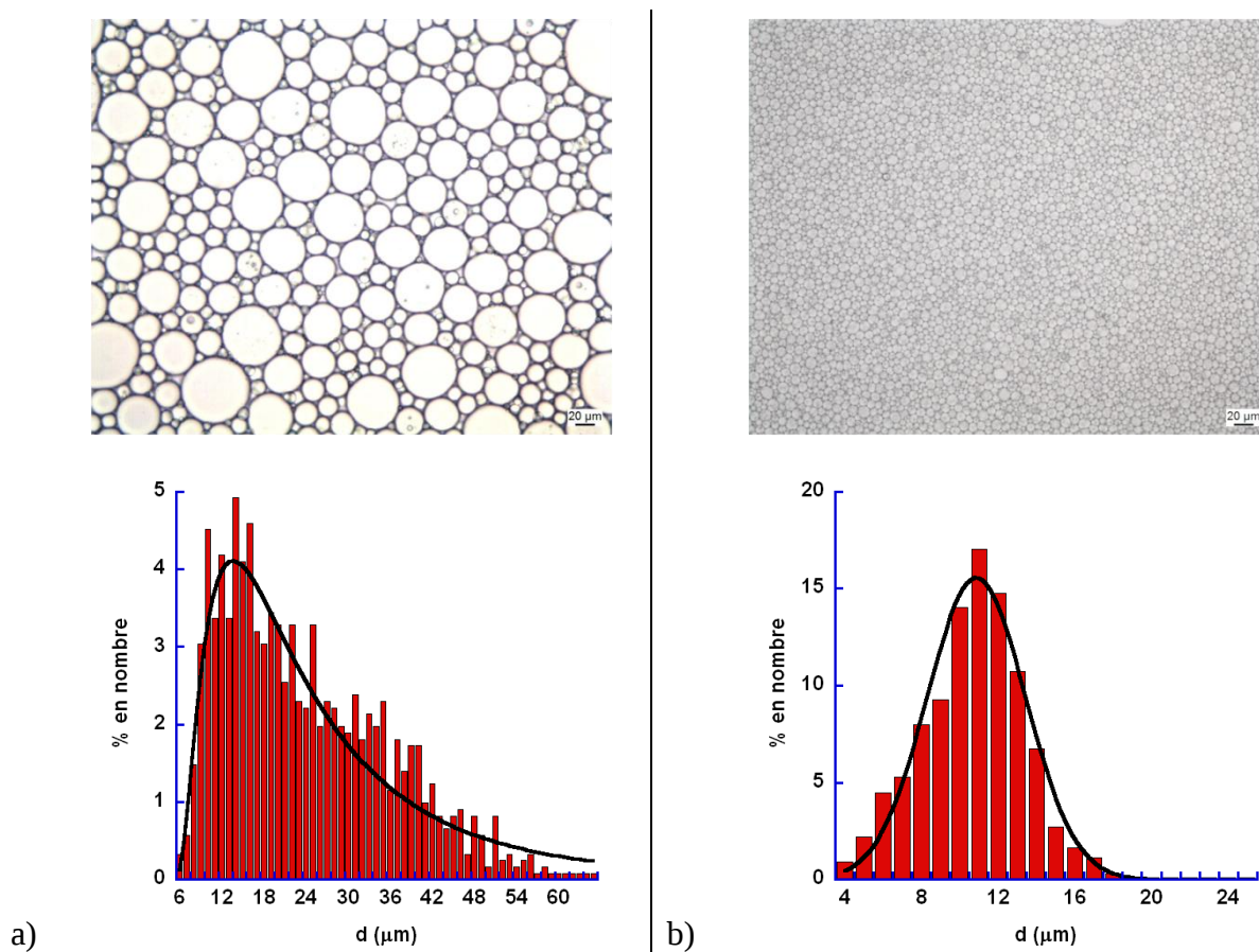
Figure 40 : Photographies prises au microscope optique et distributions en nombre de la taille des gouttes pour les émulsions réalisées a) pour l'ETC 85 et b) l'ETC 91 . Les modèles (courbes noires) sont des lois de distribution a) log-normale et b) gaussienne (normale).
