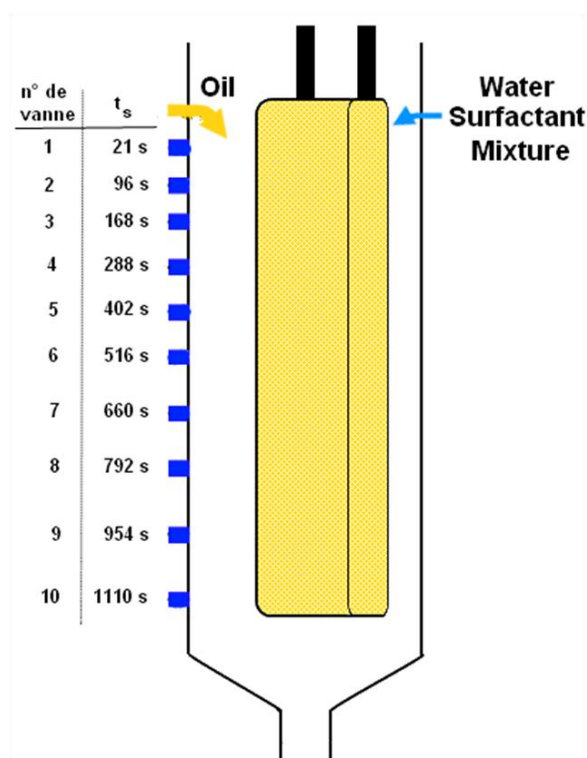
Figure 66 : Correspondance entre les vannes de prélèvement et les temps de séjour moyens des fluides dans le MDB-Cont.
