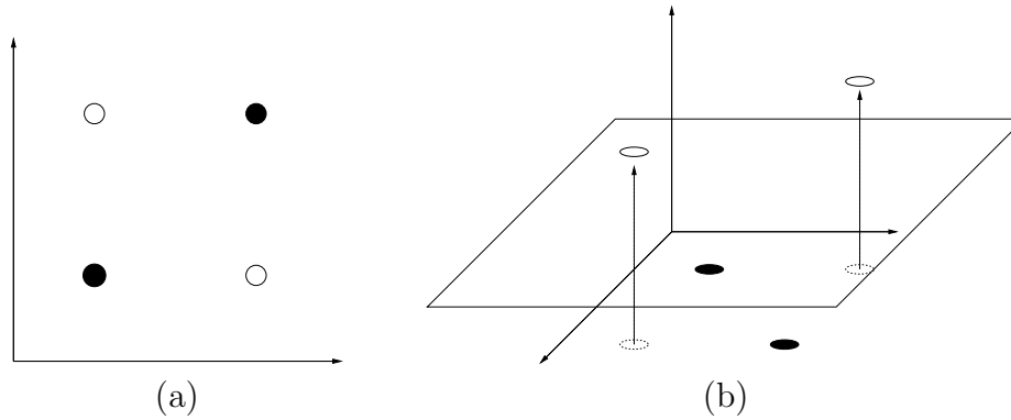
FIG. 3.1 – Dimension et pouvoir discriminant des classifieurs. Dans le cas à deux dimensions (a), il est impossible de séparer les points noirs et blancs à l’aide d’un hyperplan, alors que dans le cas à trois dimensions (b), cela devient possible.
