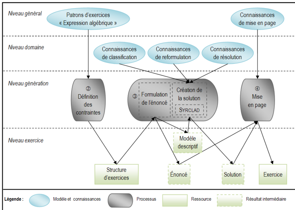
Figure A-51 : Architecture du générateur « Expression algébrique ».
