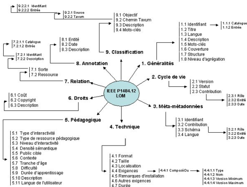
Figure 2-3 : Métadonnées du LOM [De la Passardièrre et al. 2004].
