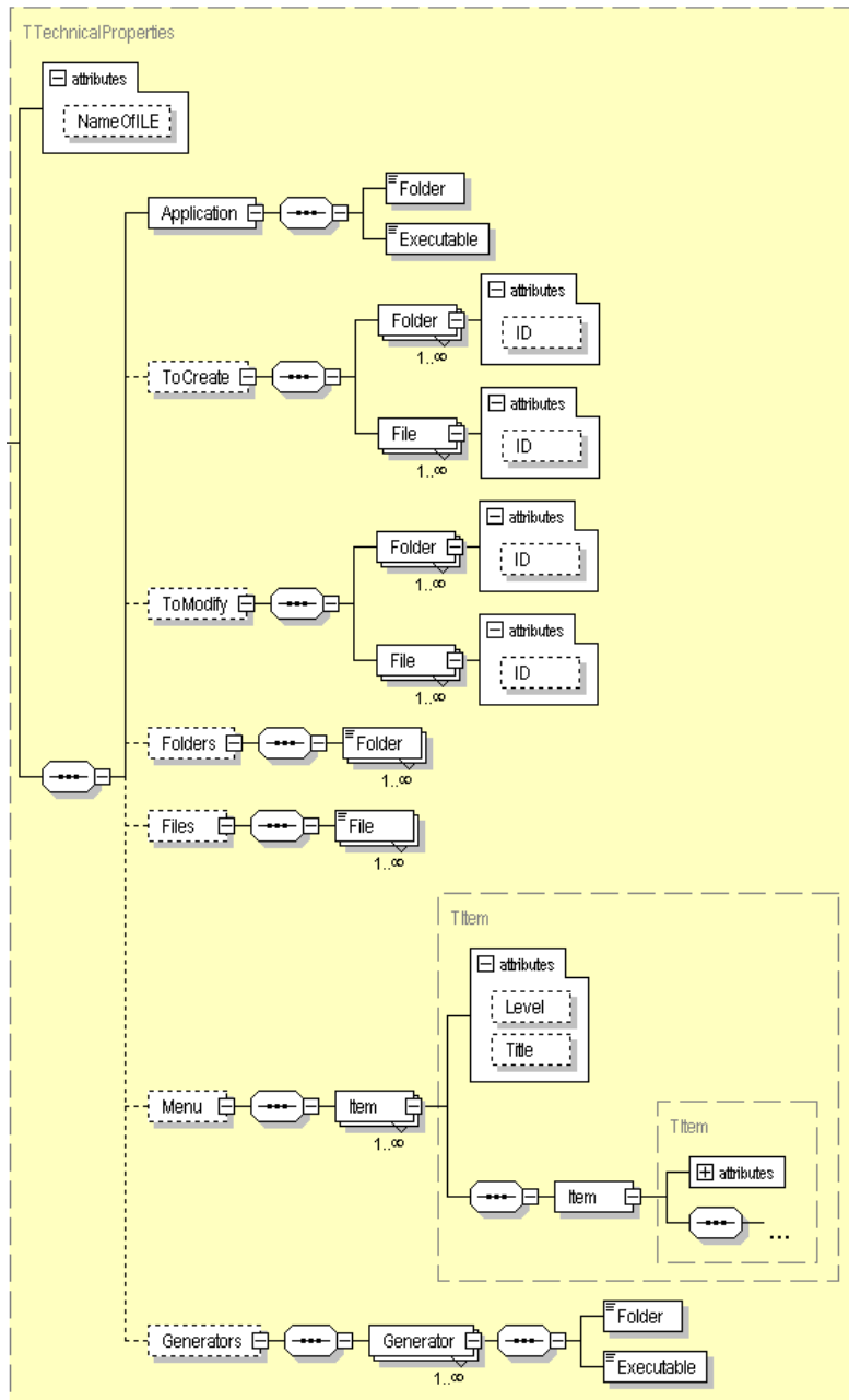
Figure 6-52 : Modèle des propriétés techniques du méta-modèle AKEPI.
