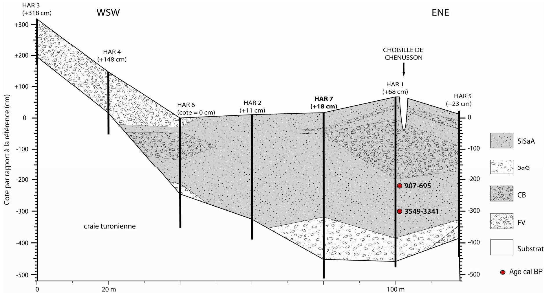
Figure 2.16 : transect lithologique sur le site HAR
