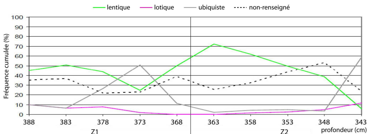
Figure 4.11 : pourcentages de répartition des Chironomidés selon leur préférence écologique dans le forage CHA9 (modifié d'après Dellile et Augé, 2009)
