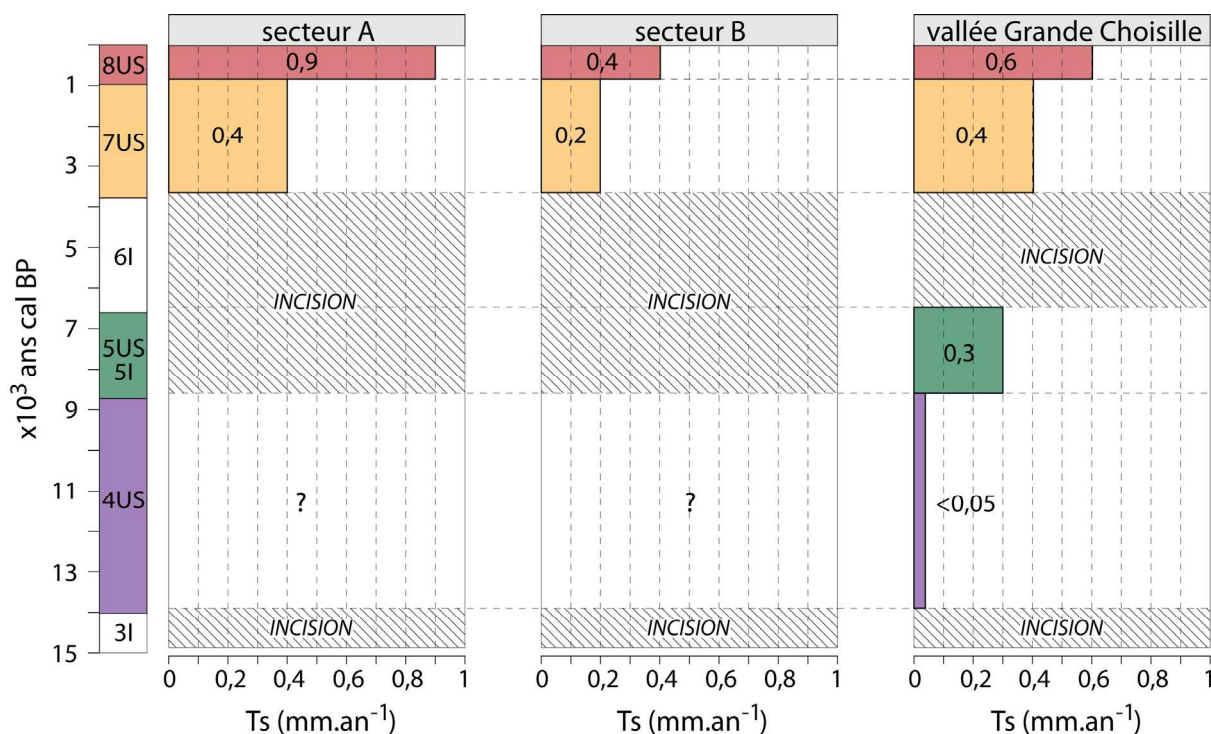
Figure 7.13 : valeurs des taux de sédimentation moyens ( T_s en \text{mm.an}^{-1} ) dans les secteurs A et B et dans la vallée principale de la Grande Choisille (incluant les secteurs C et D)
