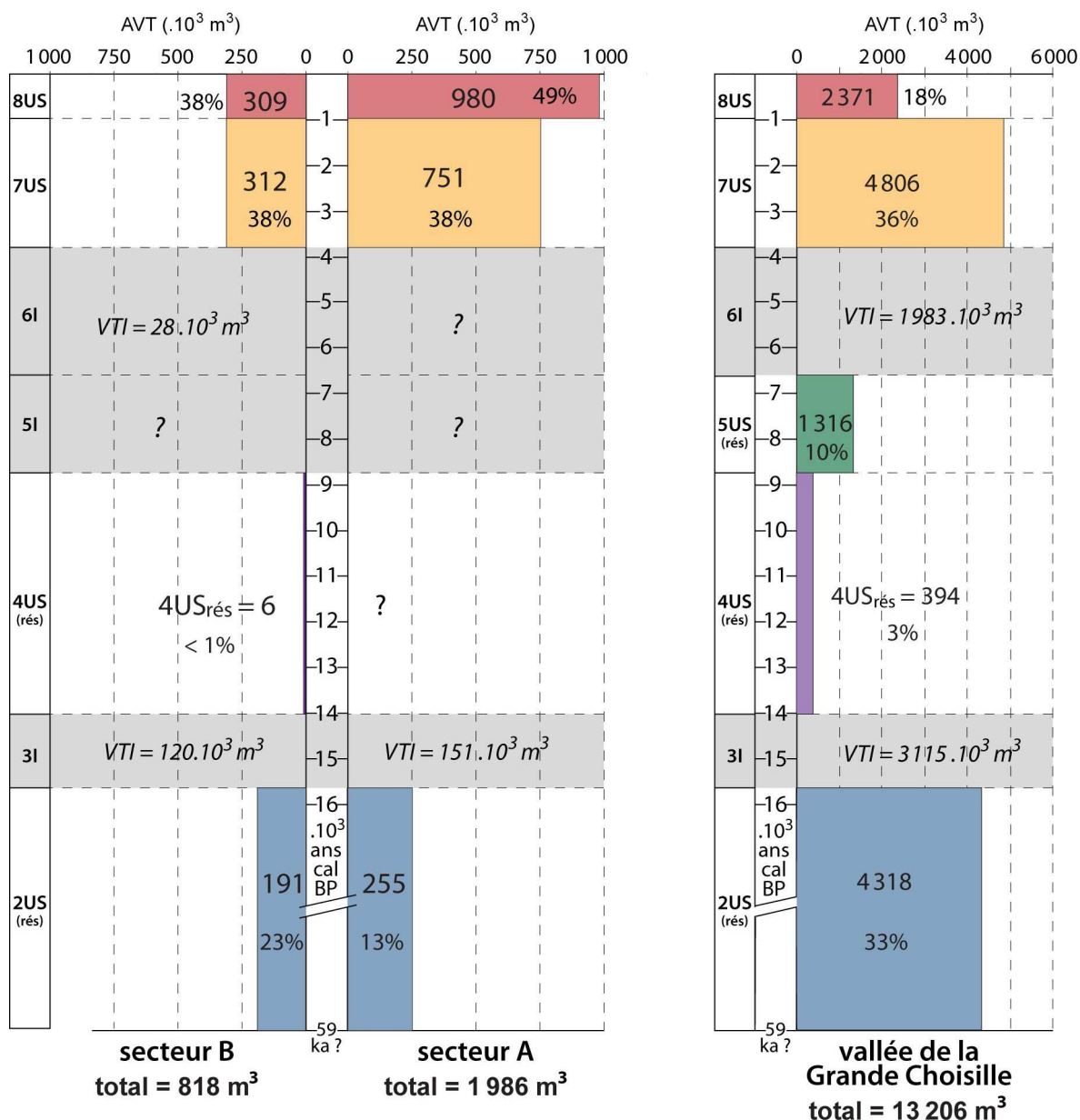
Figure 7.12 : valeurs d'accumulation volumique totale (AVT en \cdot 10^3 m^3 ) et de volume total incisé (VTI en \cdot 10^3 m^3 ) pour chaque phase dans les secteurs A et B et dans la vallée de la Grande Choisille (incluant C et D)
