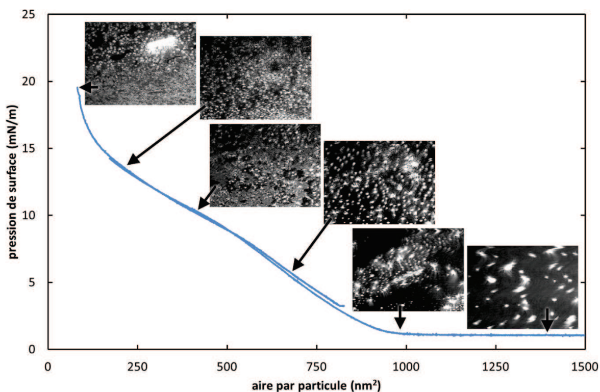
Figure 34 : Isotherme de Langmuir et photos BAM, nanoparticules moyennement hydrophobes (6.7 molécules de TMES/nm 2 ).
