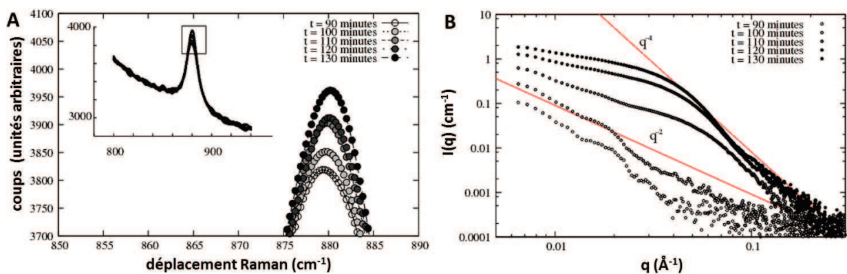
Figure 13 : Cinétique de la réaction entre 90 et 130 minutes (T=70°C), A : évolution du pic Raman à 880cm -1 , B : courbes de diffusion de la phase aqueuse.
