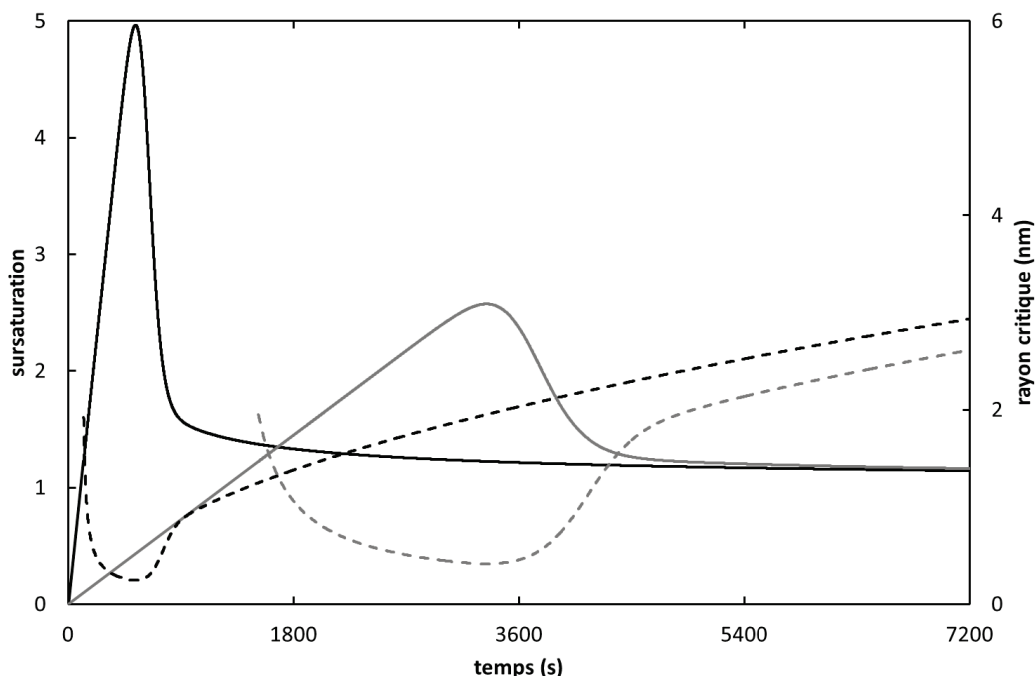
Figure 23 : Evolution de la sursaturation (lignes) et du rayon critique (pointillés) donnés par la simulation, en fonction de la vitesse d'agitation. Gris : 250rpm, noir : 1000rpm.
