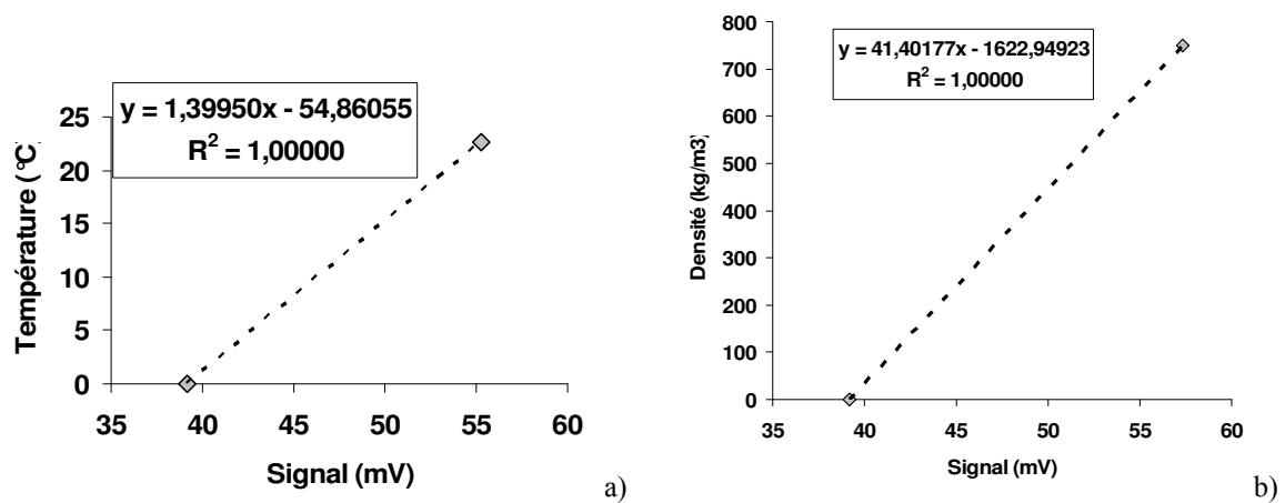
Figure 163. Droite d'étalonnage de la sortie : a) de température de tubulure du débitmètre Coriolis (Résistance aux bornes de 9,8 Ω); b) de masse volumique du débitmètre (Résistance aux bornes de 9,8 Ω).
