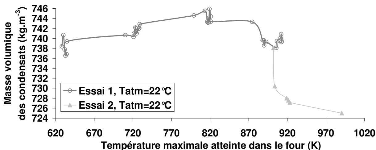
Figure 101. Evolution de la masse volumique des condensats au cours de la pyrolyse (60 bars, 0,05 g.s -1 ).
