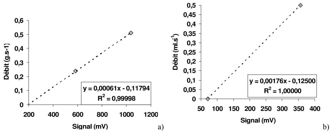
Figure 162. Droite d'étalonnage de la sortie : a) de débit massique du débitmètre Coriolis (Résistance aux bornes de 49,8 Ω); b) de débit volumique du débitmètre Coriolis (Résistance aux bornes de 18 Ω).
