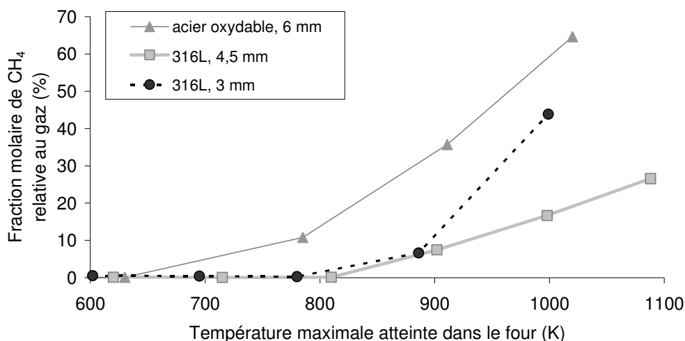
Figure 88. Effet catalytique et du diamètre interne du canal sur la formation de \text{CH}_4 (10 bars et 0,05 \text{ g.s}^{-1} ).
