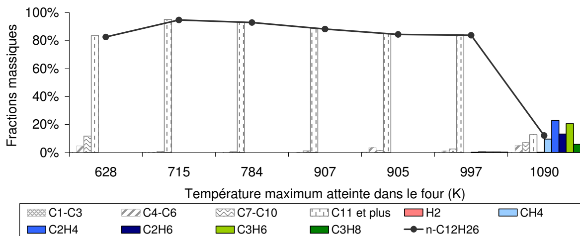
Figure 209. Distribution des produits de pyrolyse en fonction de la température maximum atteinte (produits liquides en noir & blanc; ceux gazeux en couleurs). Essais à 15 bars, 0,1 g.s -1 , réacteur de 3 mm.
