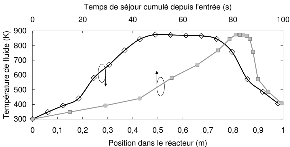
Figure 76. Température du fluide le long du réacteur chimique en fonction de la position et du temps de séjour écoulé depuis l'entrée (débit de 0,05 \text{ g.s}^{-1} ).
