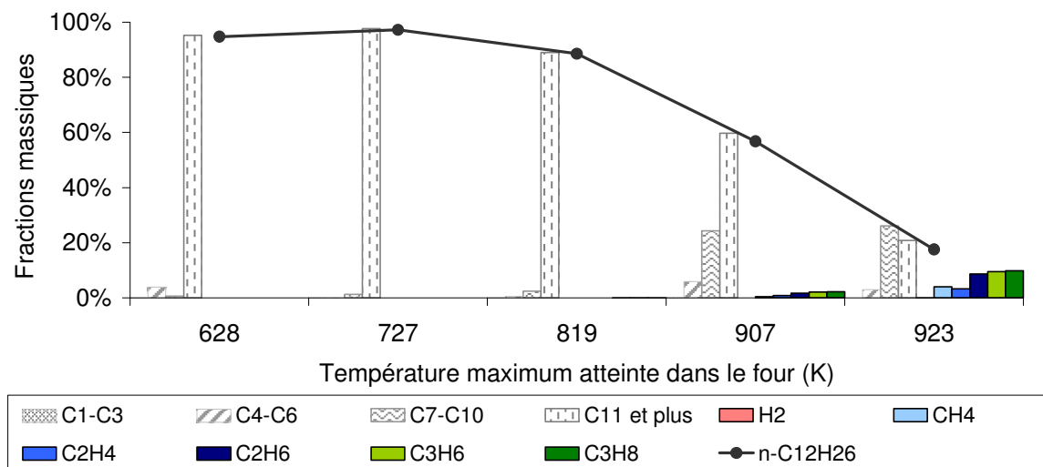
Figure 208. Distribution des produits de pyrolyse en fonction de la température maximum atteinte (produits liquides en noir & blanc; ceux gazeux en couleurs). Essais à 60 bars, 0,05 g.s -1 , réacteur de 3 mm.
