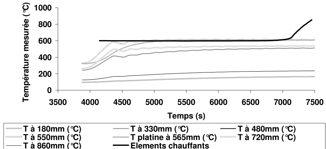
Figure 167. Variation temporelle à différentes positions de température de rayonnement du tube de travail pour une consigne programmée à 3800s à 600°C.
