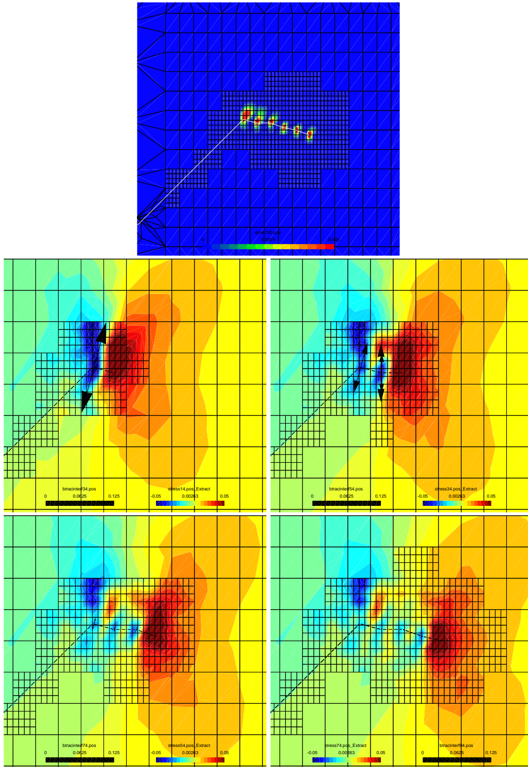
FIG. 4.34: Déformation plastique cumulée finale et efforts d'interface à F = F_{min} après la i^{ème} propagation superposé avec la composante \sigma_{yy} du tenseur des contraintes avant la i^{ème} propagation (i allant de 1 à 4).
