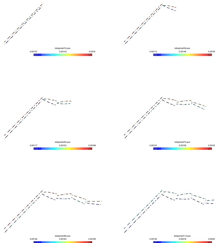
FIG. 4.33: Configurations déformées amplifiées de l'interface aux efforts minimums
