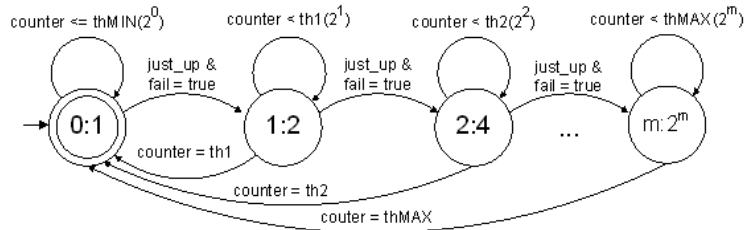
Figure 7: Mécanisme de backoff dans Q-DRAM.
