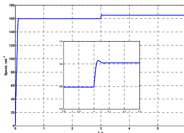
Figure 4.12. Variation de la vitesse de rotation avec un zoom sur le processus transitoire
