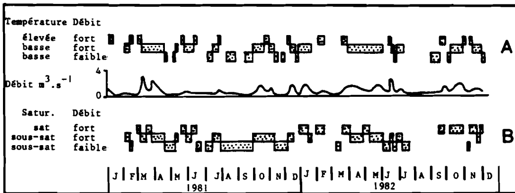
Fig. 41 : PONT DE GYS : DEBIT, TEMPERATURE ET SATURATION
