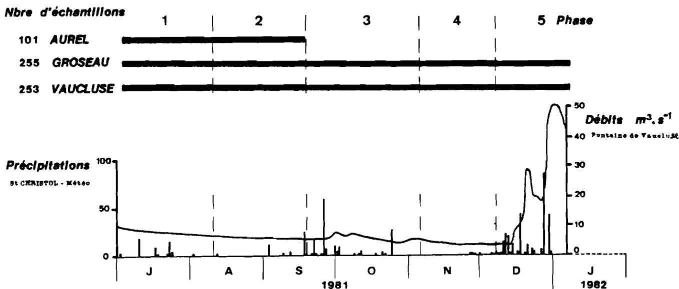
Fig. 13 : VAUCLUSE : ECHANTILLONNAGE DE TROIS SOURCES
