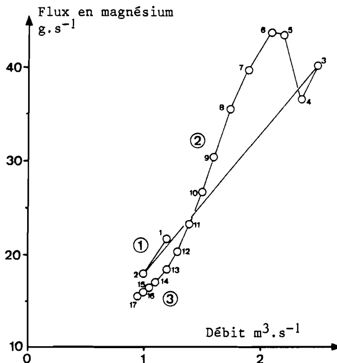
Fig. 152 : RELATION FLUX EN MAGNESIUM-DEBIT. SOURCE DU LEZ, CRUE DE JUIN 1973
