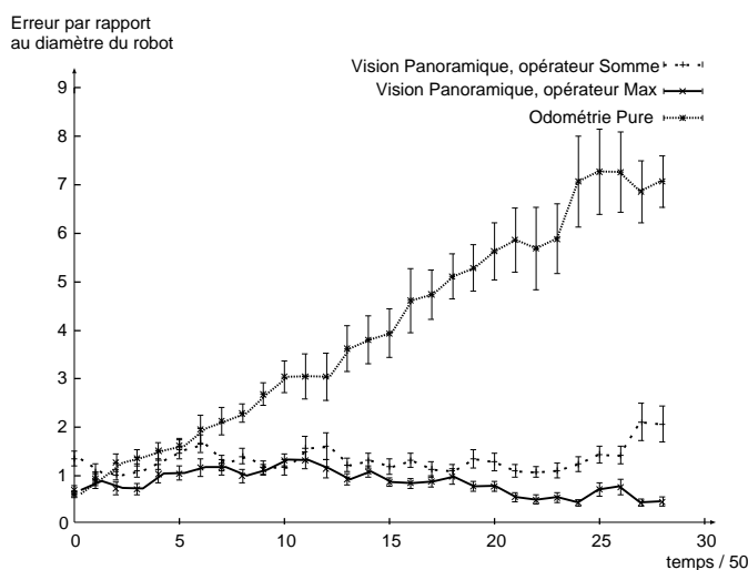
FIG. 6.8: Évolution de l'erreur de l'estimation de la position au cours de la cartographie de l'environnement de la figure 6.6 en utilisant l'opérateur somme et l'opérateur max. L'évolution de l'erreur de l'odométrie est donnée pour comparaison. Ces valeurs sont les moyennes sur dix expériences. Chaque unité de l'axe des abscisses correspond à cinquante pas de temps.
