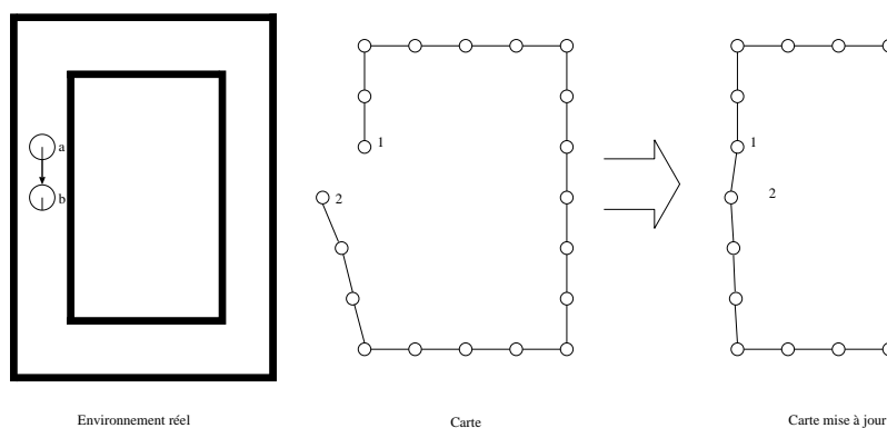
FIG. 5.12: Exemple de cas dans lequel les données idiothétiques doivent être intégrées à la carte. Le robot se déplace ici de la position a à la position b. L'estimation de cette position reste correcte et passe du nœud 1 au nœud 2. Dans ce cas, la position relative des nœuds 1 et 2 et le déplacement mesuré par l'odométrie sont différents à cause d'erreurs de la carte. Ajouter les données idiothétiques relevées entre les nœuds 1 et 2 permet donc d'améliorer la carte. Le seuil empêchant ce type de mises à jour doit donc être choisi pour permettre de tels phénomènes.
