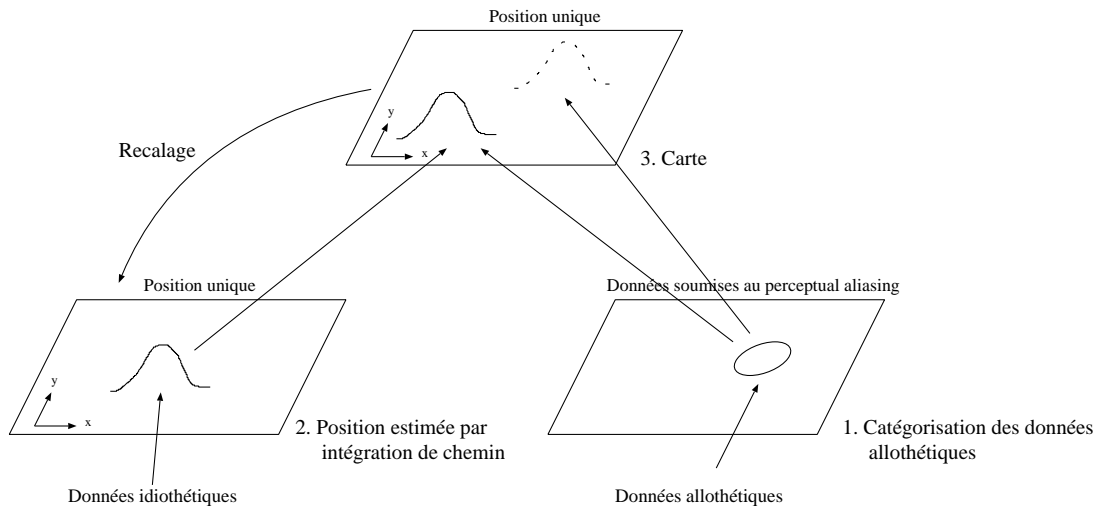
FIG. 7.1: Structure fonctionnelle du modèle d'Arléo et Gerstner (voir le texte pour les explications).
