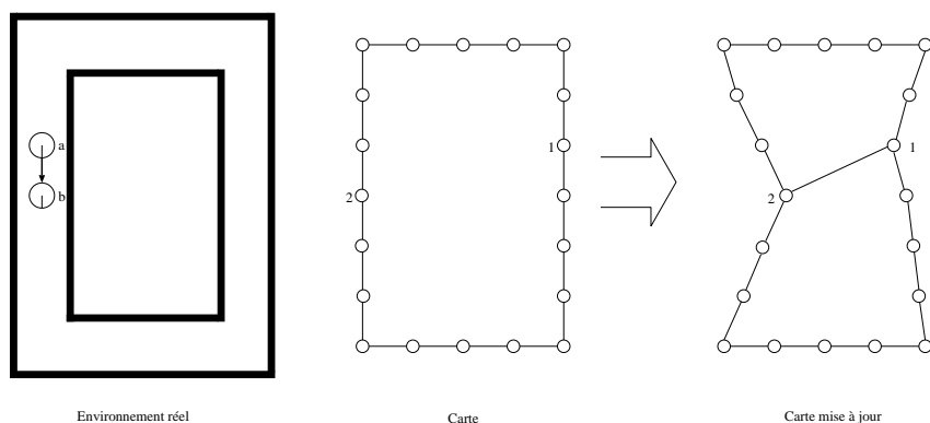
FIG. 5.11: Exemple de cas dans lequel les données idiothétiques ne doivent pas être intégrées à la carte. Le robot se déplace ici de la position a à la position b. L'estimation de cette position, qui était initialement fautive, passe du nœud 1 au nœud 2. Ajouter une connexion et les données idiothétiques relevées entre les nœuds 1 et 2 dans ce cas conduit à une carte à la topologie erronée. Pour limiter ce phénomène, l'ajout de connexion n'est réalisé que si la position relative des nœuds 1 et 2 et le déplacement mesuré par l'odométrie sont suffisamment proches.
