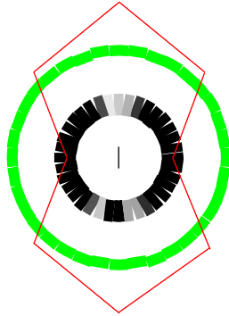
FIG. 6.12: Représentation des données mémorisées dans un nœud de la zone entourant le point A (cf. figure 6.6). La ligne brisée joint les points détectés au moyen des sonars. Nous pouvons constater l'effet des réflexions des sonars dont l'angle d'incidence sur les murs est de 45 degrés. Ces réflexions conduisent à une surestimation de la distance des obstacles. Le cercle intérieur montre le niveau de gris de l'environnement pour toutes les directions réparties autour du robot. L'épaisseur du cercle extérieur indique le nombre de perceptions effectuées dans chaque direction. Ici, cette épaisseur est constante car une caméra panoramique est utilisée.
