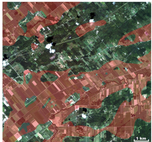
FIGURE 3 Dépôts géomorphologiques de la zone étudiée : Les zones recouvertes par des dépôts marins ont été surlignées en rouge ; les zones recouvertes par des dépôts morainiques n'ont pas été modifiées.
