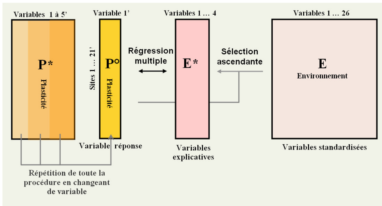
FIGURE 8 Schéma de la procédure suivie pour analyser les relations entre variables plastiques et variables environnementales : une sélection progressive des variables ascendante en régression multiple est appliquée sur la matrice environnementale ; La matrice [E*] regroupe les variables ainsi sélectionnées ; une régression multiple est réalisée en utilisant la matrice [E*] comme matrice explicative et chacune des variables plastiques identifiées précédemment comme ayant un impact sur la prolifération des populations comme variable réponse ; l'apostrophe est utilisée après les nombres de variables, nombre de site ou numéro d'espèce quand ceux-ci varient d'une espèce à l'autre : la valeur donnée est alors uniquement fournie à titre d'exemple.
