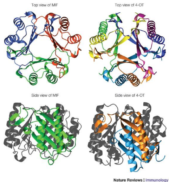
Figure 23. Structure de la protéine MIF. Comparaison des structures tertiaires de MIF et de la 4-OT bactérienne. D'après (Calandra and Roger, 2003).
