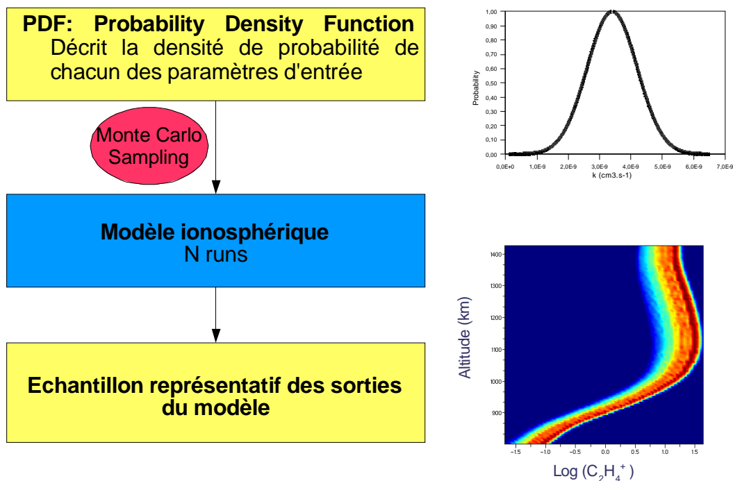
Figure 8: Principe de la propagation d'incertitude par tirages Monte Carlo.
