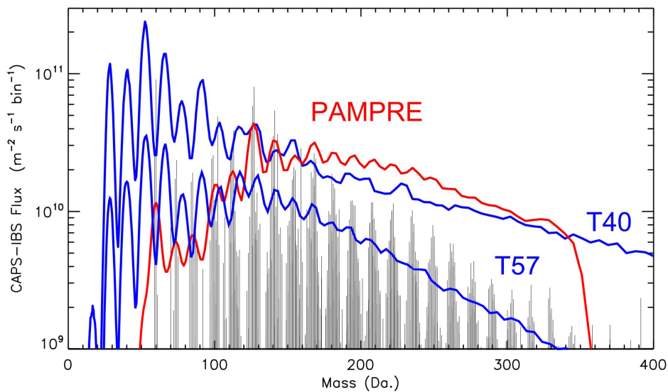
Figure 15: (Bleu) Spectres de masse mesuré par CAPS-IBS lors des survols T40 et T57 de Cassini à 1015km d'altitude. (Noir) Spectre de masse des tholins de PAMPRE à haute résolution (Pernot et al., 2010). (Rouge) Spectre de masse des tholins, avec une résolution dégradée, identique à celle de CAPS-IBS.
