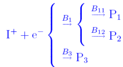
Figure 24 : Exemple de la fragmentation d'un ion par recombinaison dissociative avec un électron.
