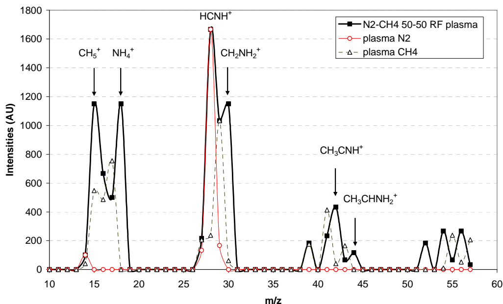
Figure 17 : Spectres de masse des ions mesurés dans un plasma RF d'azote pur, de méthane pur et d'un mélange 50-50 d'azote-méthane (Carrasco et al., 2011)
