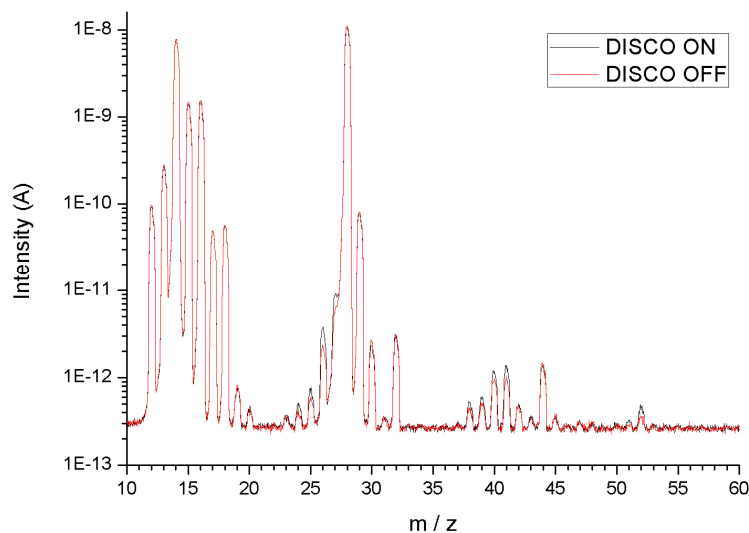
Figure 23 : Effet d'environ 1 h d'irradiation DISCO sur un mélange N 2 -CH 4 90-10%.
