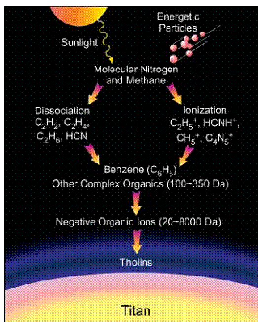
Figure 7 : Processus de formation des aérosols dans la haute atmosphère de Titan (Waite Jr. et al., 2007)
