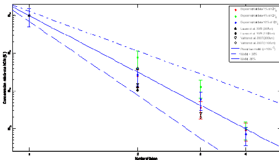
Figure 16 : concentration relative des nitriles en fonction du nombre de carbones dans les molécules. Les points rouge, vert et bleu représentent les points expérimentaux de différentes expériences menées sur PAMPRE. Les courbes bleues représentent la modélisation en loi de puissance de ces points expérimentaux. Les autres symboles (noirs et blancs) représentent les données d'observations de Cassini tirées d'observations CIRS à 300 km et INMS à 1100 km (Vuitton et al., 2007), ainsi que du modèle de Lavvas et al., 2008.
