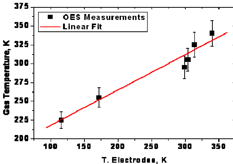
Figure 19 : Evolution de la température du gaz neutre en fonction des parois de la cavité plasma, refroidies par une circulation d'azote liquide.
