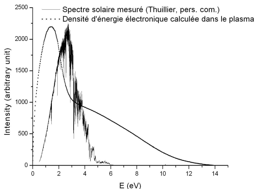
Figure 20 : EEDF du plasma DC d'azote-méthane de Bernard, 2004, compare au spectre solaire : courbe pleine : spectre solaire ; courbes pointillée : EEDF du plasma DC.
