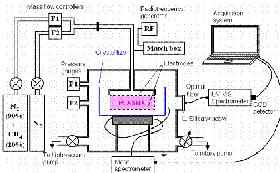
Figure 12 : Schéma de l'expérience PAMPRE.
