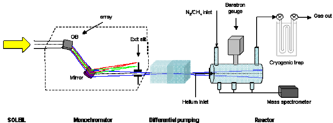
Figure 21 : Schéma du réacteur APSIS pour la ligne de lumière DISCO du synchrotron SOLEIL.
