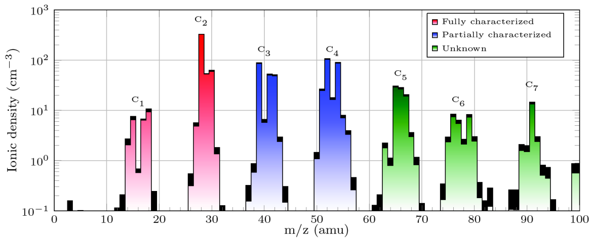
Figure 26 :Spectre de masse des ions mesuré par l'instrument INMS au cours du survol diurne T19 à 1100 km d'altitude. La couleur des blocs indique l'état des connaissances sur les produits neutres issus des recombinaisons dissociatives des ions identifiés.
