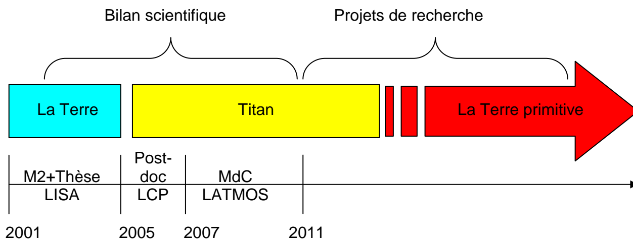
Figure 2: schéma de mon parcours et de mon projet de recherche.
