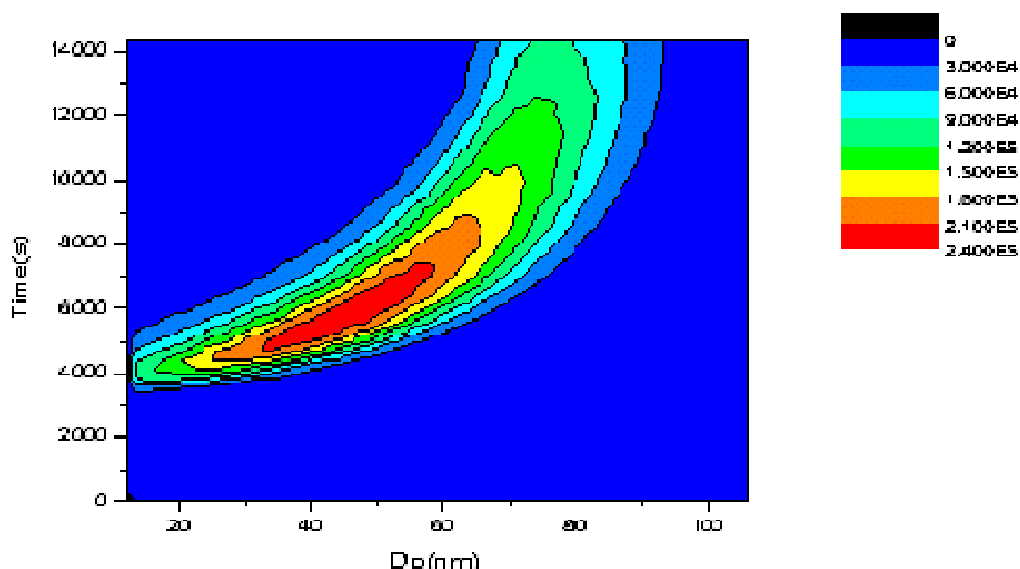
Figure 5 : Production d'aérosols organiques au cours de la réaction de photo-oxydation du MBO: nombre de particules produites par unité de volume ( \text{cm}^{-3} ) en fonction des classes de diamètre (nm) et du temps (s).
