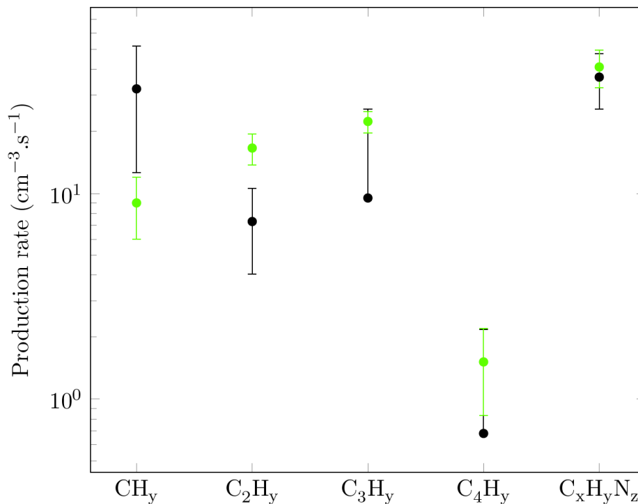
Figure 27 : Comparaison des vitesses de production de neutres à 1100 km. (Noir) Vitesse de production par le modèle photochimique ; (vert) vitesse de production par les recombinaisons dissociatives avec les densités ioniques mesurées par INMS au cours du survol T19 à 1100 km d'altitude.
