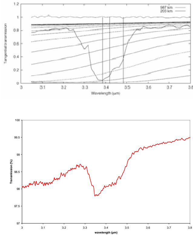
Figure 14 : (Bas) bande d'absorption infra-rouge à 3.4 μm d'un tholin de PAMPRE; (Haut) Même absorption mesurée par transmission tangentielle des aerosols de Titan par l'instrument VIMS de Cassini (Rannou et al., 2010).
