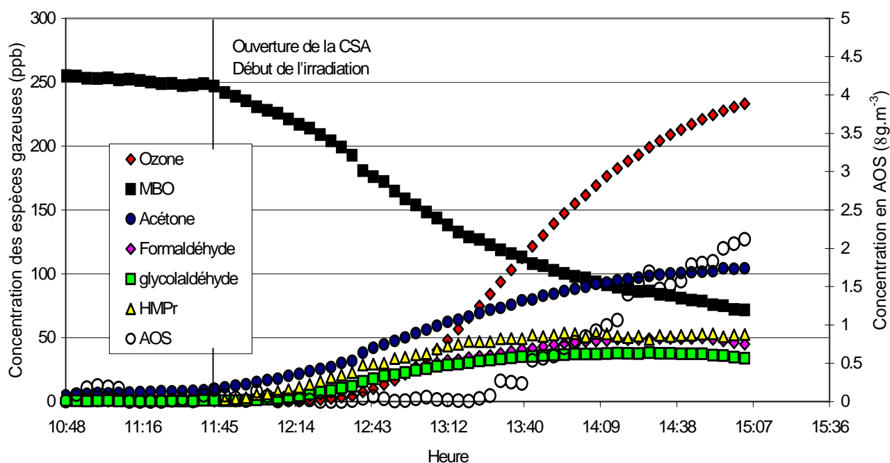
Figure 4 : Expérience de photo-oxydation réaliste du MBO (EUPHORE 19/05/03).
