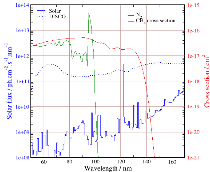
Figure 22 : Comparaison des spectres en énergie de DISCO et du Soleil.
