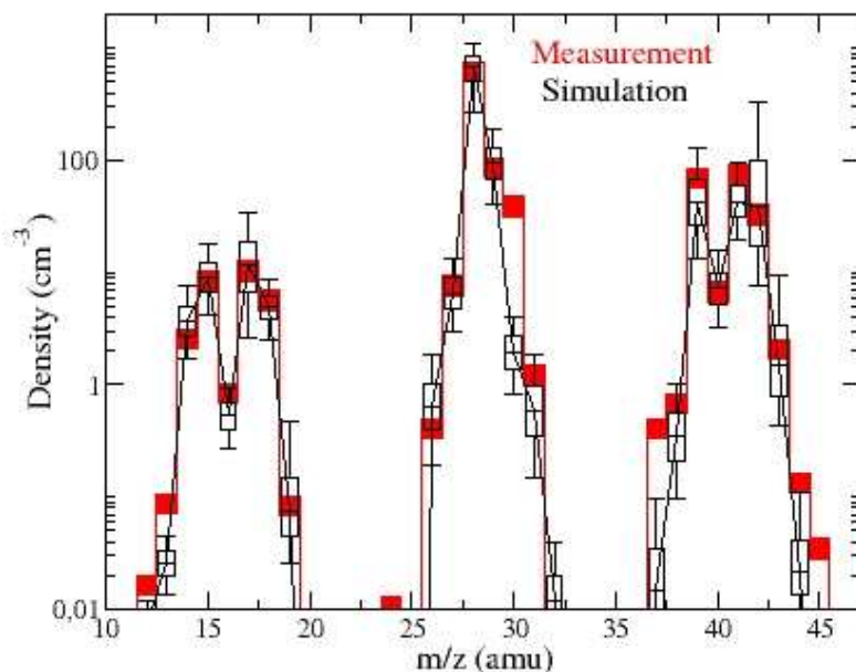
Figure 9 : Comparaison des spectres de masse des ions (rouge) mesuré par l'instrument INMS à 1200km lors du vol T5 ; (noir) simulé dans Carrasco et al., 2008b.
