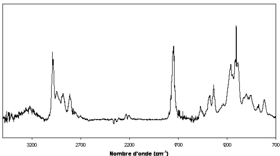
Figure 6: Spectre de référence de HMP r – 4,9 \times 10^{13} molécule. \text{cm}^{-3} – L = 156 m – R = 0,7 \text{cm}^{-1}
