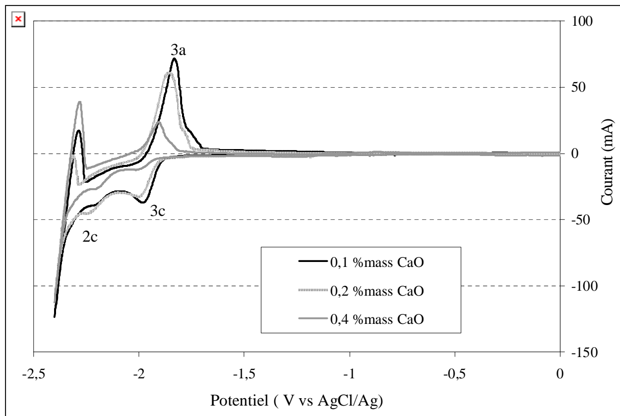
Figure 3-11 : Voltampérogrammes cycliques dans CaCl 2 -KCl (4 %mas CeCl 3 ) à 750°C et 0,1 V/s sur électrode de tungstène (0,2 cm 2 ) lors d'ajouts de CaO (0,1 à 0,4 %mass)
