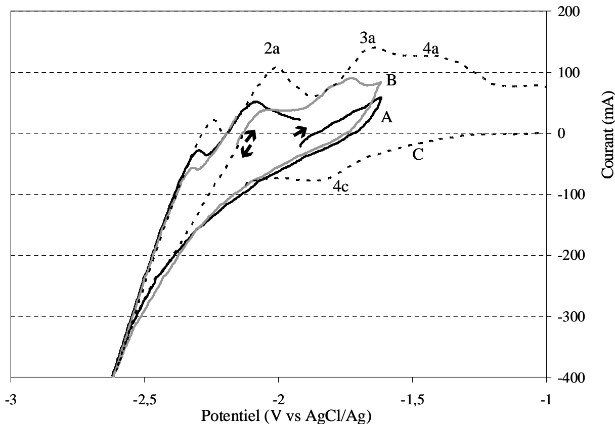
Figure 3-20 : Voltampérogrammes enregistrés dans CaCl 2 -KCl à 750°C sur fil de tungstène (0,8 cm 2 ) servant d'amenée de courant à une pastille de cériine poreuse (24 %vol) après des chronoampérométries à : A\ -2,1 V (30 Coulombs) ; B\ -2,2 V (50 C) ; C\ -2,3 V (15 C)
