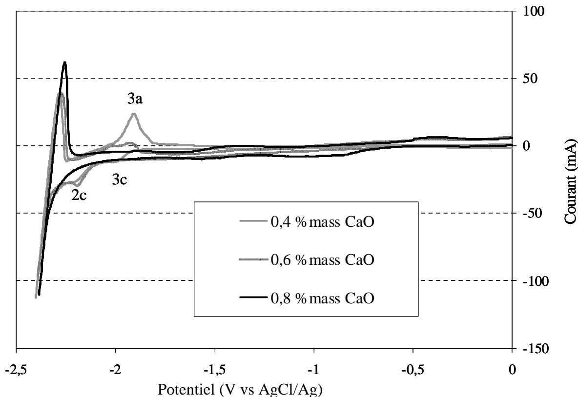
Figure 3-12 : Voltampérogrammes cycliques dans CaCl 2 -KCl (4 %mas CeCl 3 ) à 750°C et 0,1 V/s sur électrode de tungstène (0,2 cm 2 ) lors d'ajouts de CaO (0,4 à 0,8 %mass)
