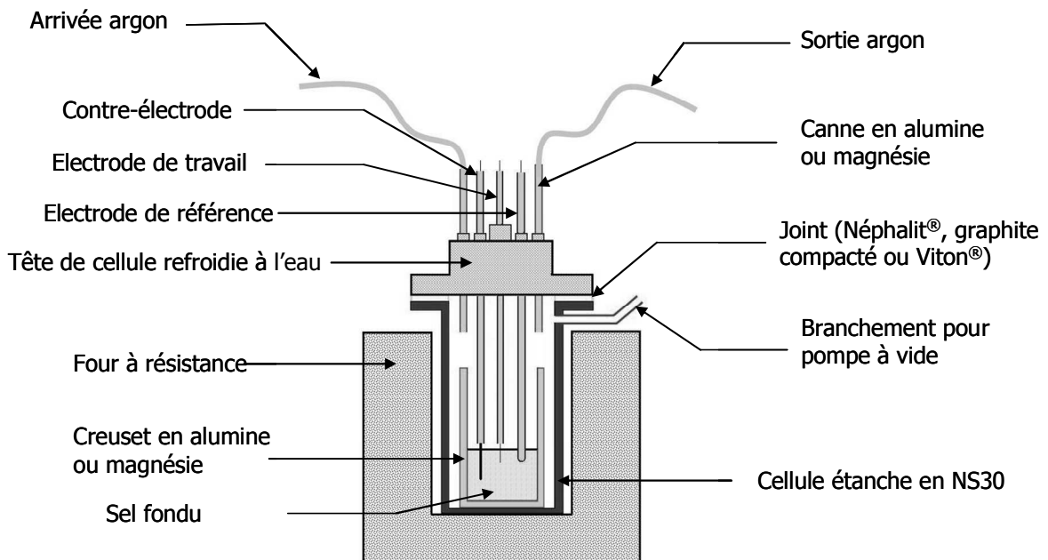
Figure 2-1: Schéma du montage expérimental avec la première cellule utilisée (cf. Figure 2-2)
