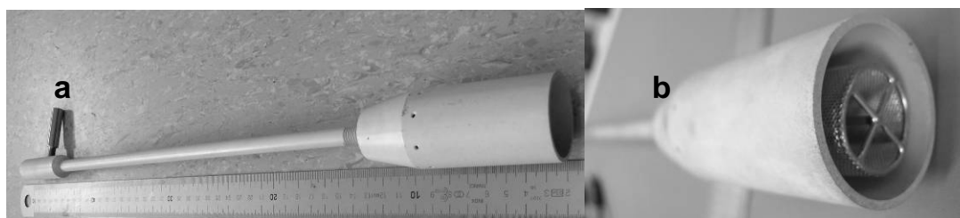
Figure 5-3 : a) Photo de la cloche en nitrure de bore, de la canne d'évacuation des gaz et de l'adaptateur pour la sortie des gaz; b) Photo d'une anode en platine à l'intérieur de la cloche
