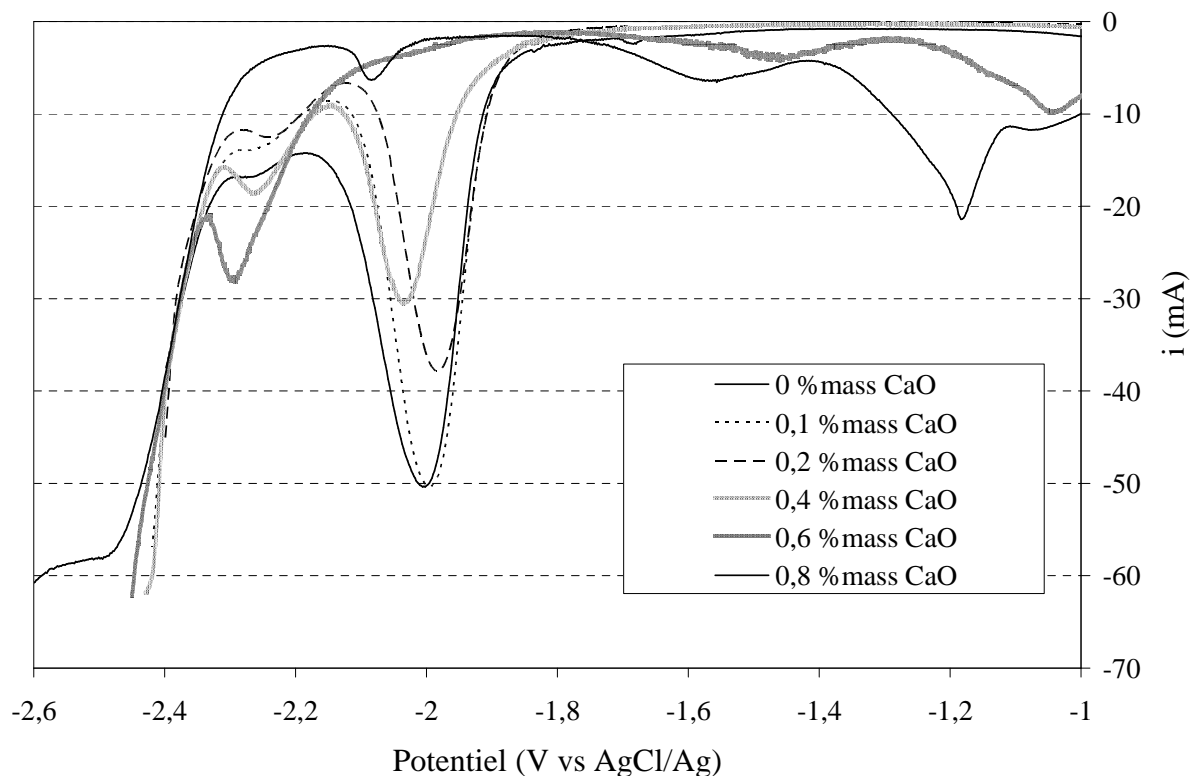
Figure 3-14 : Voltampéromogrammes à vague carrée enregistrés dans \text{CaCl}_2\text{-KCl} (4 %mas \text{CeCl}_3 ) à 750^\circ\text{C} et 0,1 \text{ V/s} sur électrode de tungstène ( 0,2 \text{ cm}^2 ) lors d'ajouts de \text{CaO} (0,1 à 0,8 %mass)
