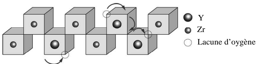
Figure 1-6 : Schéma de diffusion des ions oxyde dans une membrane de type YSZ
