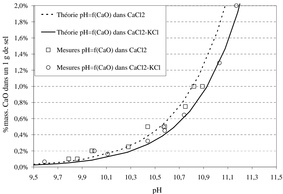
Figure 2-13 : Variation de la concentration en CaO (en %mass.) dans les sels CaCl 2 et CaCl 2 -KCl en fonction du pH
