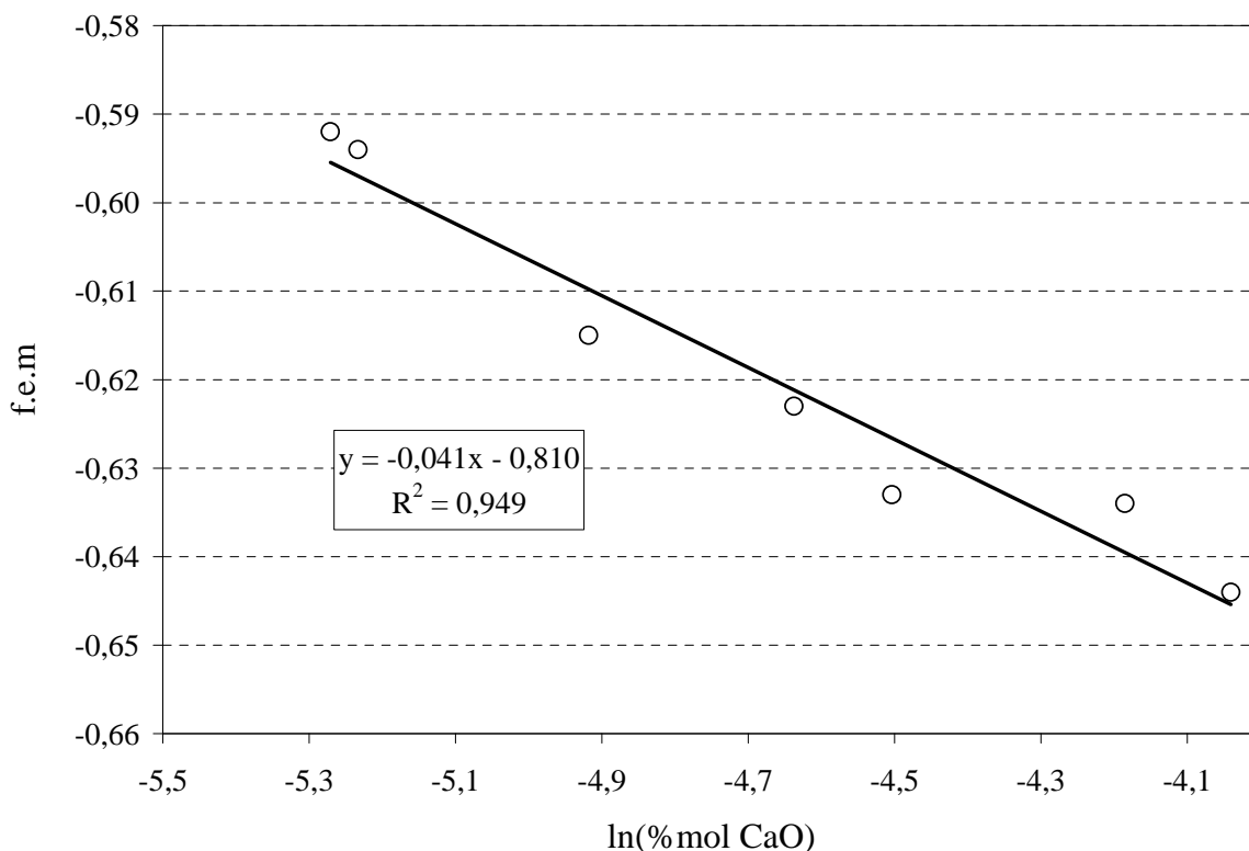
Figure 2-17 : Etalonnage du capteur à ions oxyde dans CaCl 2 -CaO à 890°C
