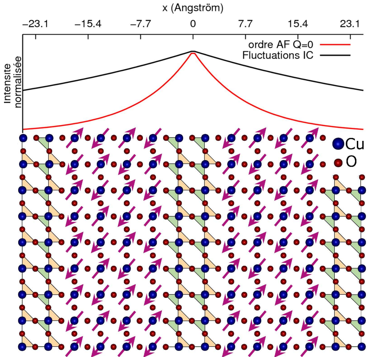
FIGURE 6.15 – Schéma de 13x8 mailles élémentaires dans La_{1.915}Sr_{0.085}CuO_4 . On remarque les deux zones AF en antiphase sur 4 mailles de long séparées par des zones riches en trous où se développe l'ordre AF à Q = 0 symbolisé par les triangles jaunes et verts. Les longueurs de corrélations mesurées expérimentalement coïncident avec cette image puisqu'elles sont de 2 mailles suivant l'axe (1, 0, 0) et de 3 mailles suivant la diagonale. Dans ce cas il n'y a pas de corrélation entre les boucles d'une échelle à deux montants à une autre. En haut sont représentées les transformées de Fourier des Lorentziennes, indiquant les longueurs de corrélations dans l'espace direct.
