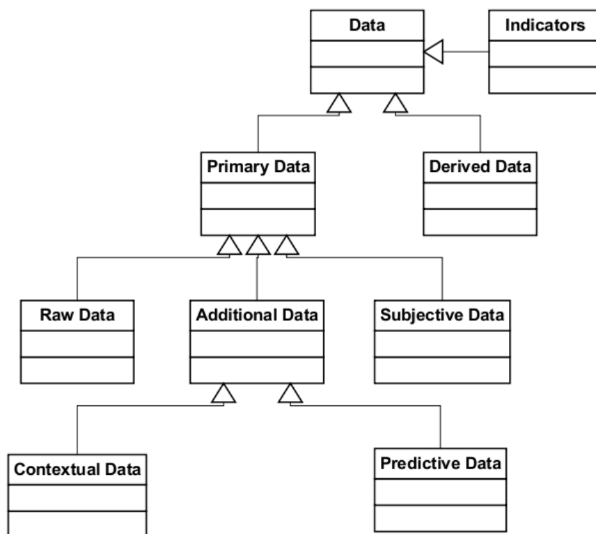
Figure 2-8 Typologie des données d'observation proposée par DPULS
