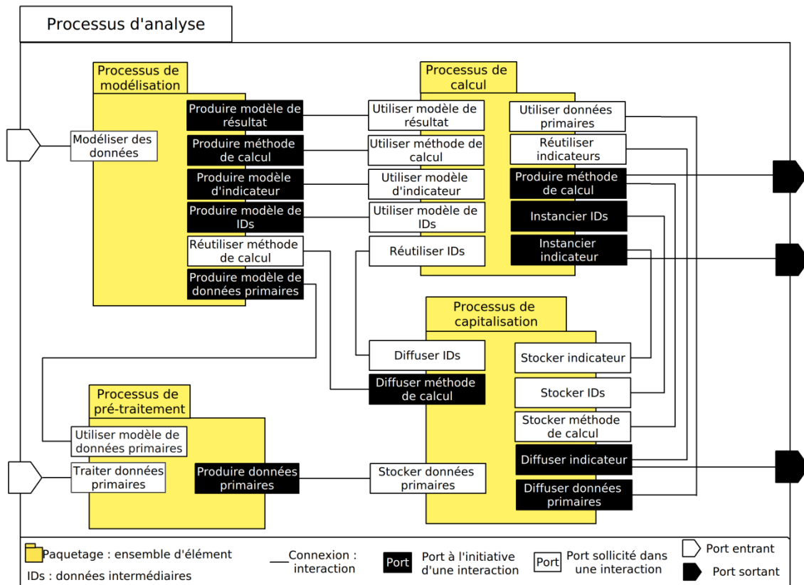
Figure 4-2 Les quatre processus du processus d'analyse des traces
