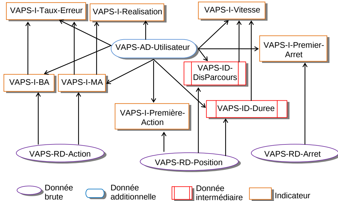
Figure 6-14 La cartographie des données du VAPS
