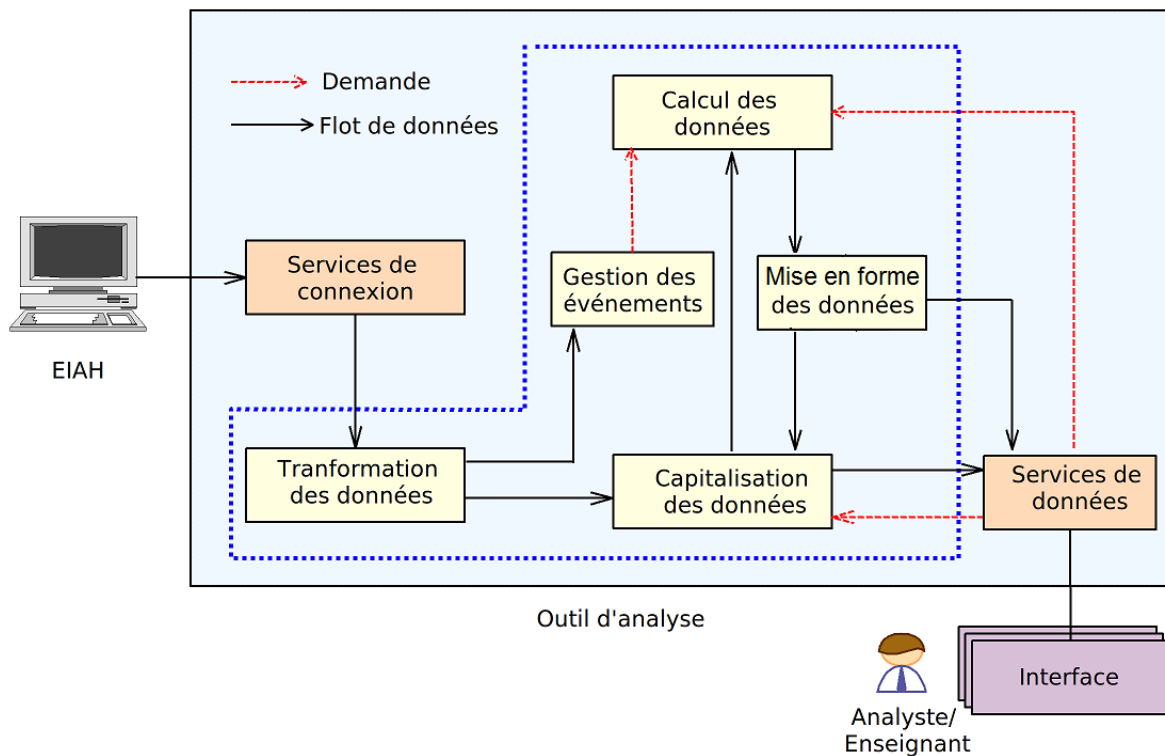
Figure 6-1 L'architecture générale de l'outil d'analyse des traces
