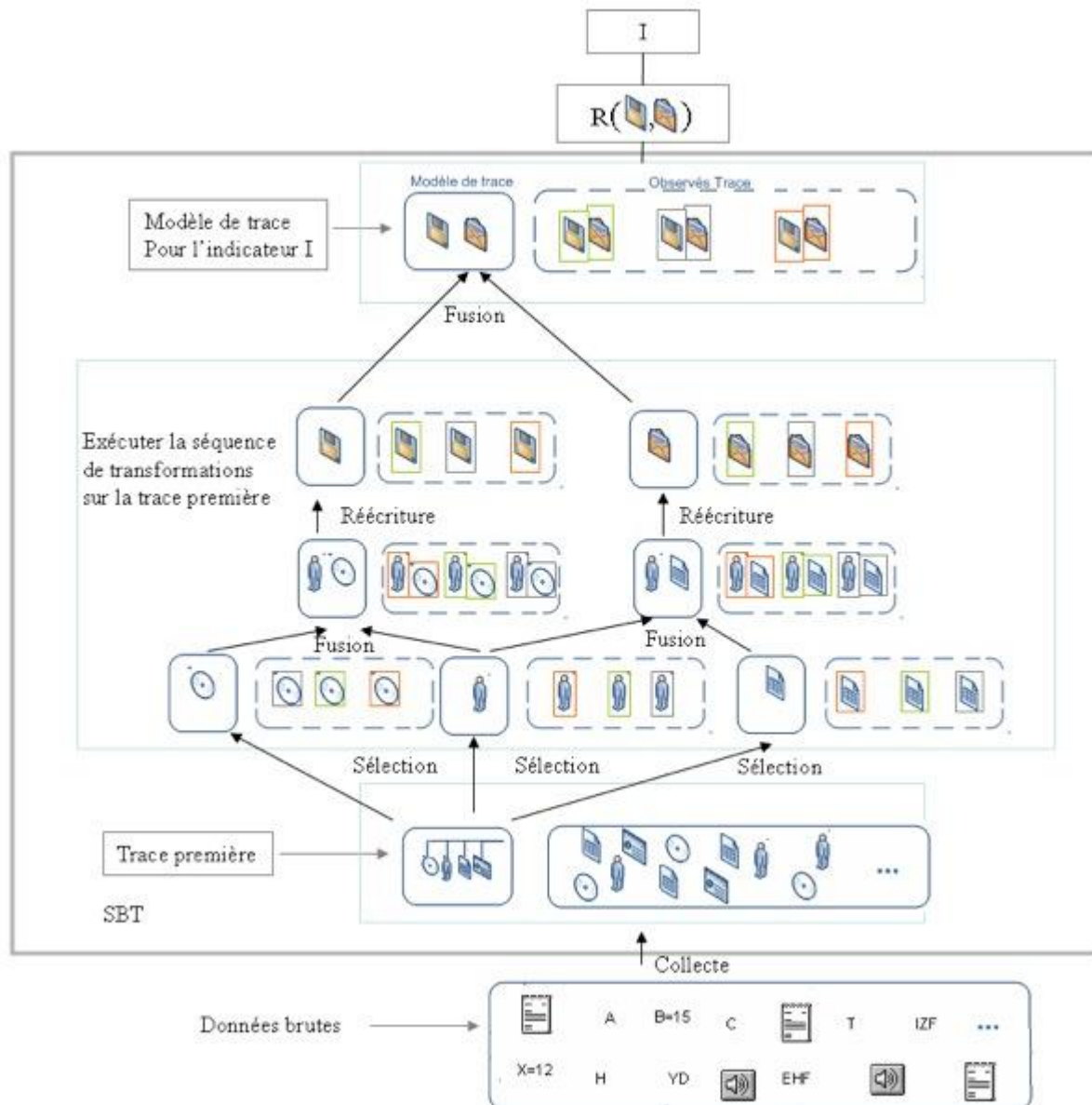
Figure 2-19 La séquence de transformations sur la trace première [Djouad et al. (2009)]
