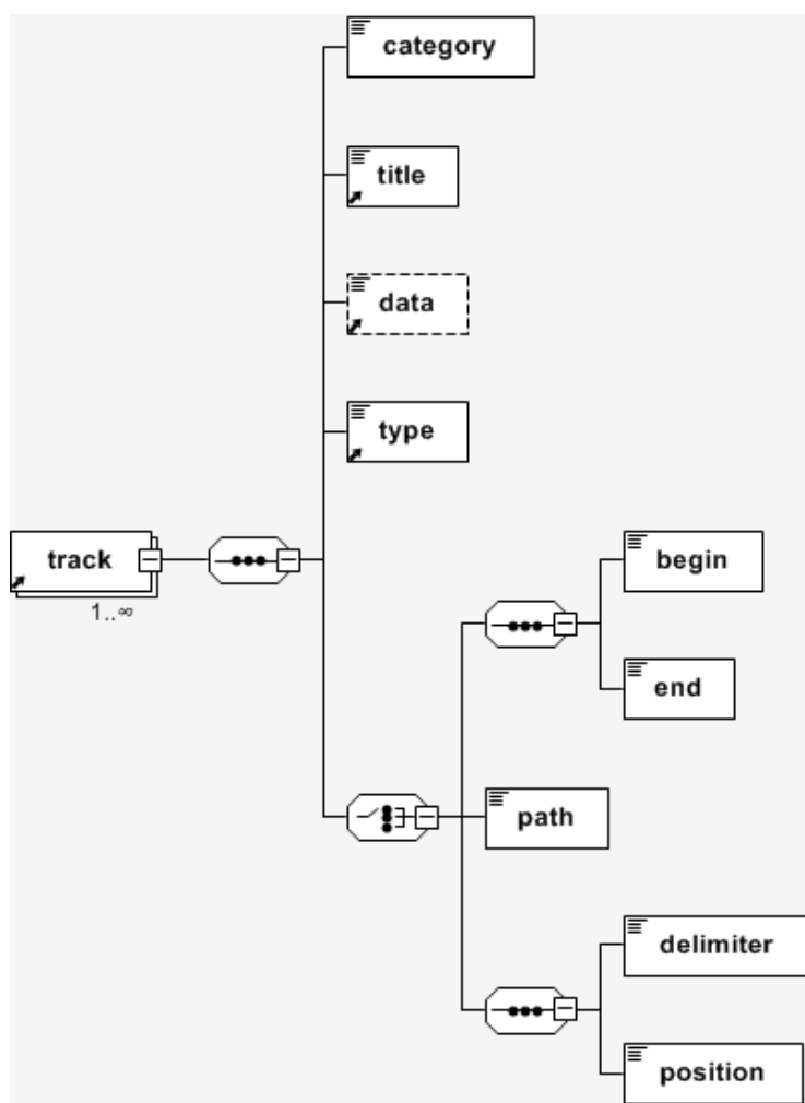
Figure D-3 Le modèle d'information d'une trace
