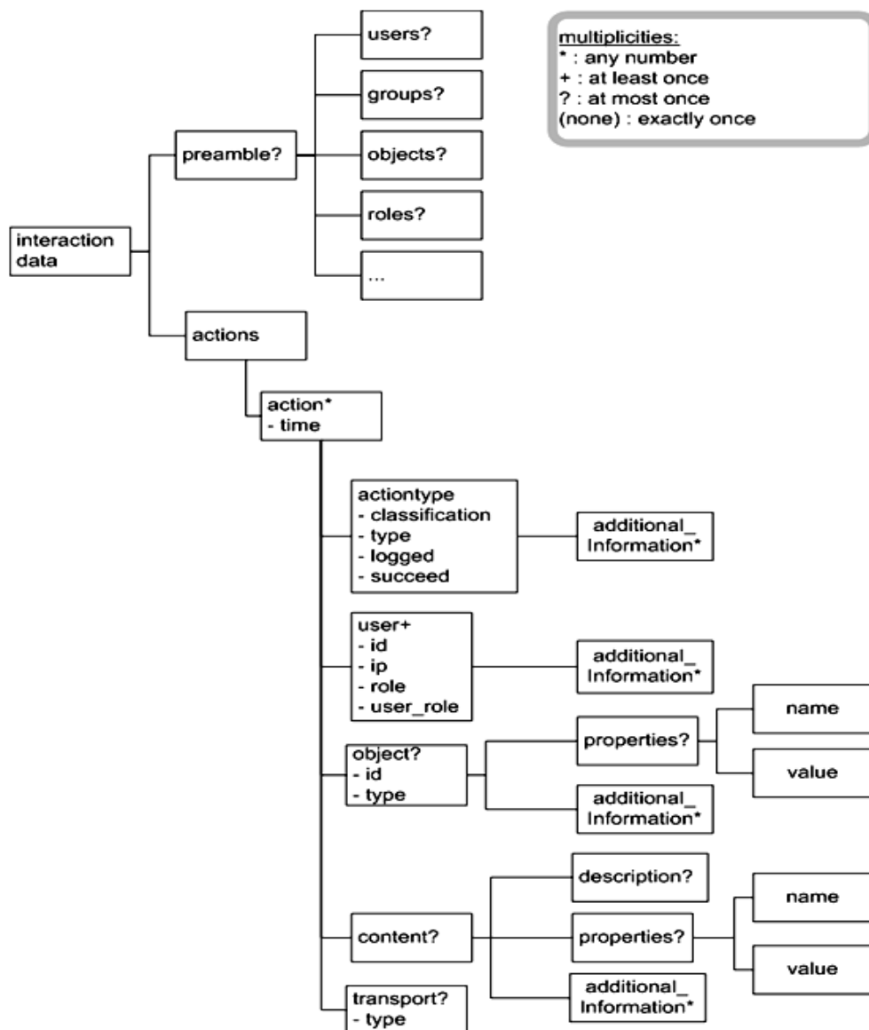
Figure 2-6 Structure simplifiée du format commun de traces proposé par CAViCoLA
