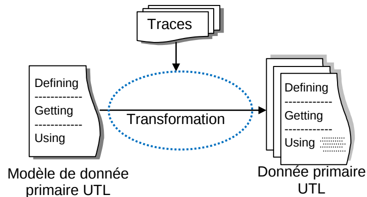
Figure 4-3 Le processus de prétraitement de données
