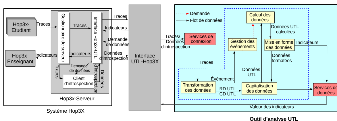
Figure 7-10 L'architecture de l'outil d'analyse en interaction avec Hop3x
