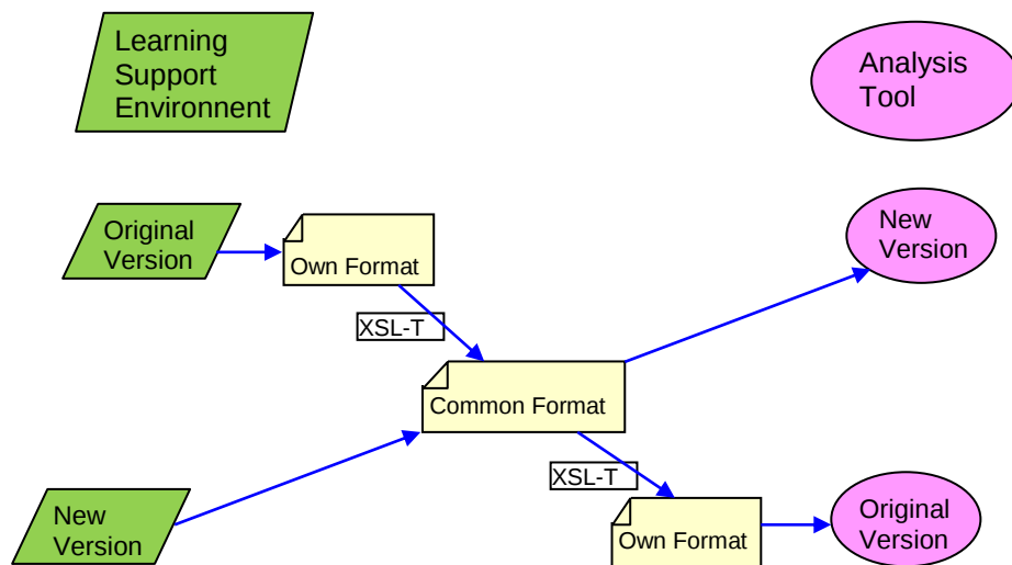
Figure 2-7 Communication entre un EIAH et un outil d'analyse via un format commun DTD
