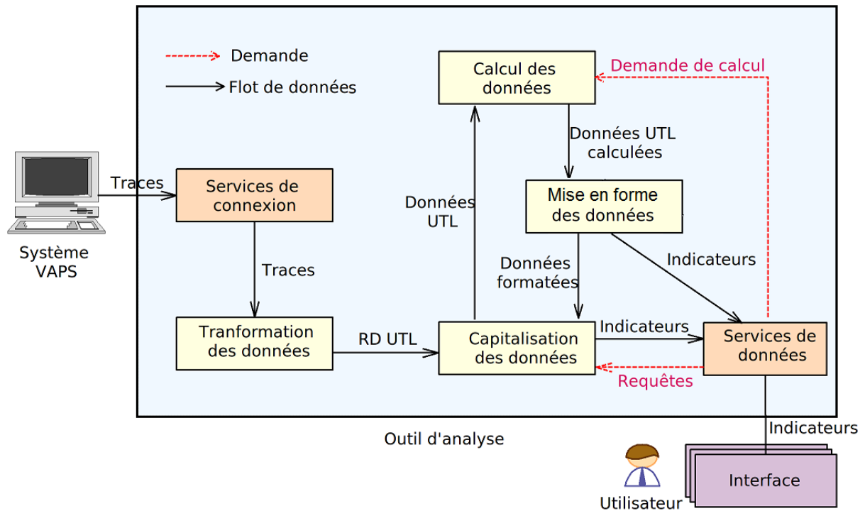
Figure 6-8 Le modèle d'application pour le calcul d'indicateurs après la session
