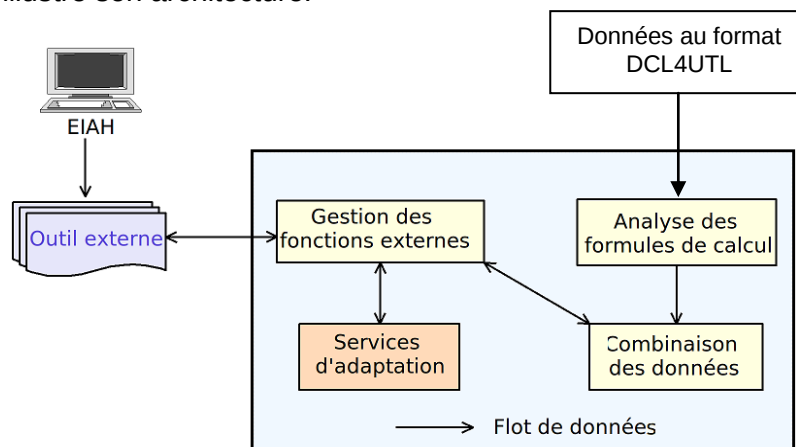
Figure 6-2 L'architecture de composant “Calcul des données”
