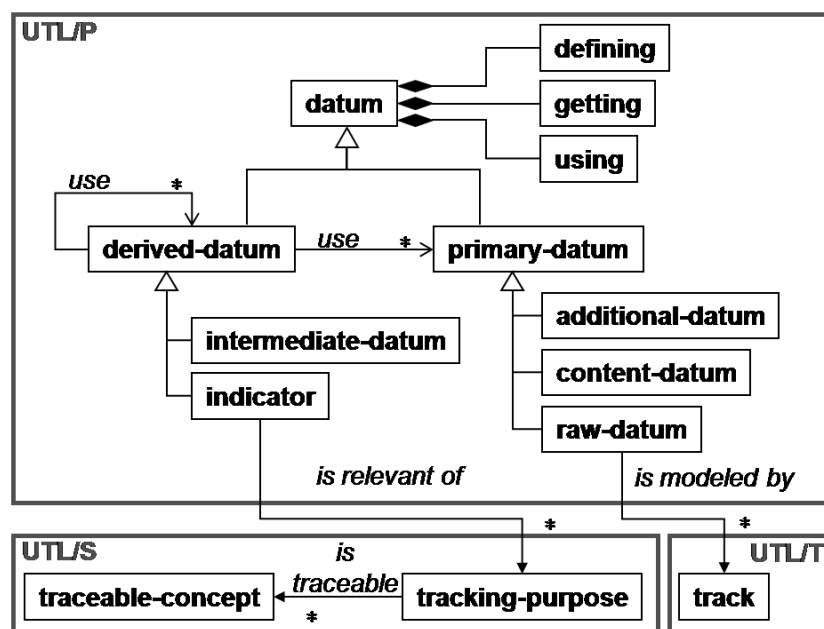
Figure 2-10 Le modèle conceptuel d'UTL
