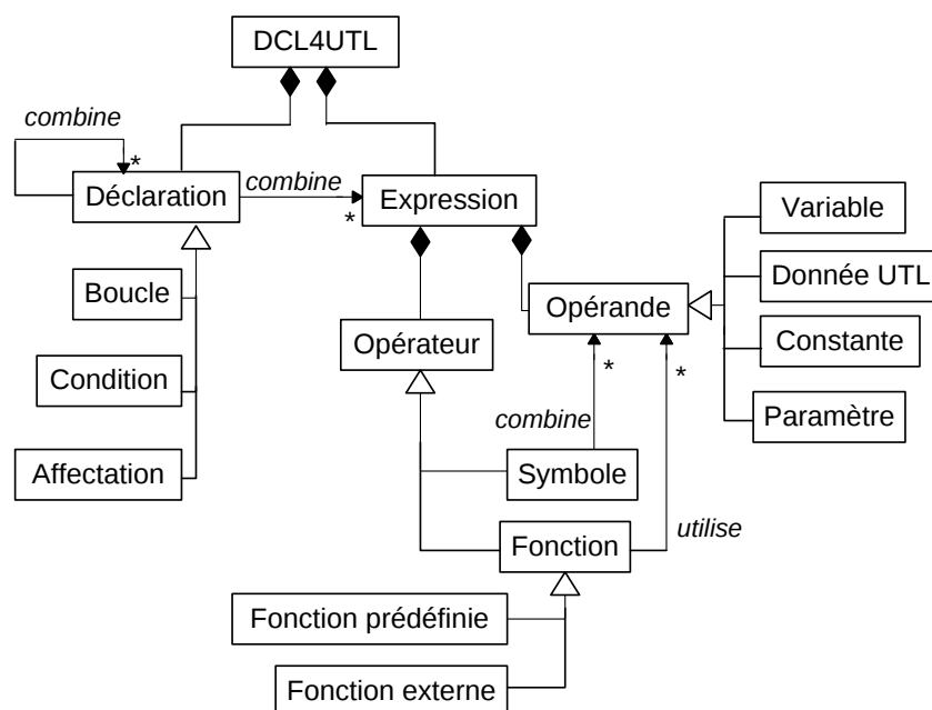
Figure 5-3 La structure du langage DCL4UTL
