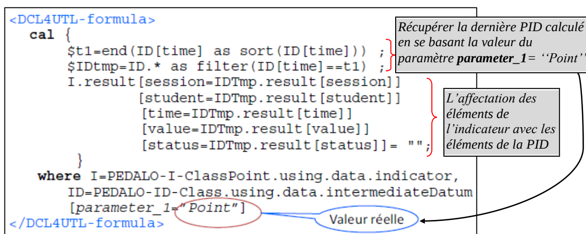
Figure 7-8 La méthode de calcul de l'indicateur PEDALO-I-ClassPointExist
