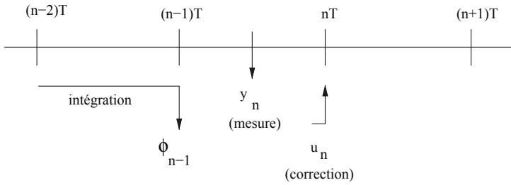
FIGURE 2.6 – Chronologie de la boucle d'asservissement.
