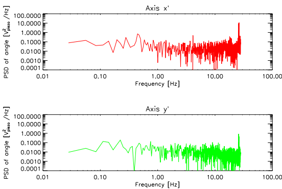
(a) DSP de tip et de tilt.
