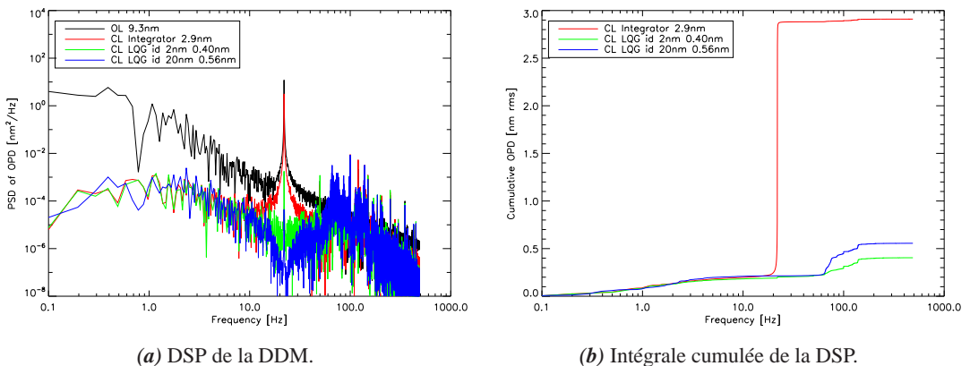
FIGURE 4.45 – Correction d'une vibration de 10 nm d'amplitude, avec une identification réalisée sur une vibration de 2 nm et 20 nm d'amplitude.
