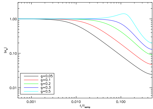
(b) Fonction de transfert de bruit.
