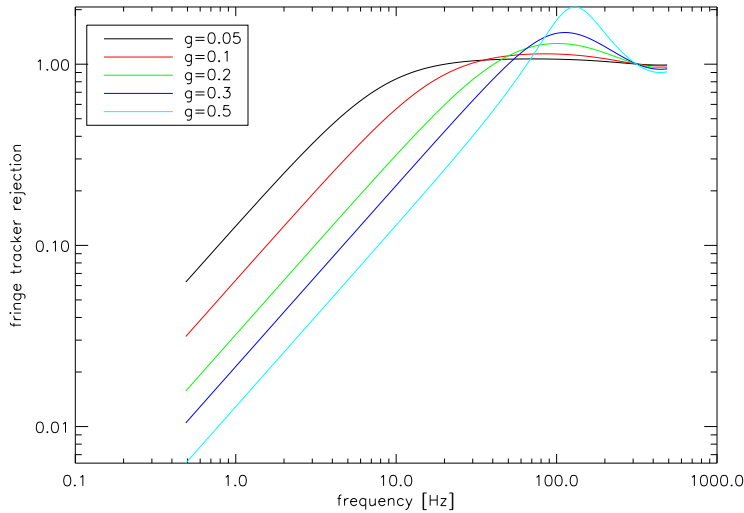
FIGURE 4.30 – Fonction de transfert de réjection du suiveur de franges, en fonction du gain de l'intégrateur.
