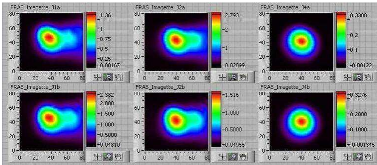
(a) Alignement non optimal.
