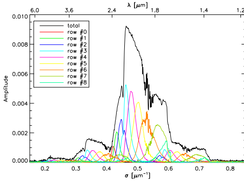
(e) Bande \mathcal{H-K} , spectre non corrigé.
