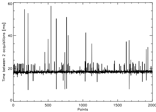
(a) Écart temporel entre deux mesures consécutives du CLOWFS.
