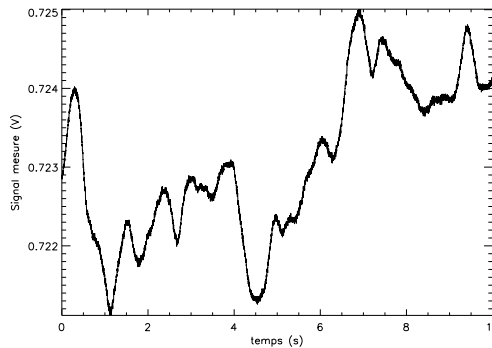
(c) Signal de frange brillante.
