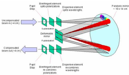
(a) Principe de l'adaptive nuller.
