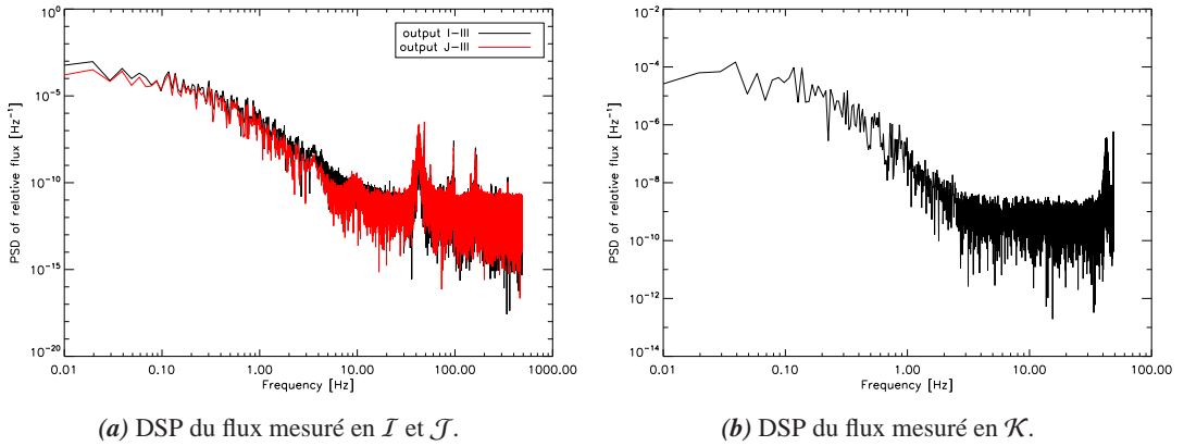
FIGURE 3.21 – DSP du flux mesuré en I , J et K lorsque le flux moyen injecté est maximal.
