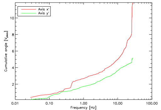
(b) Intégrale cumulée de la DSP.
