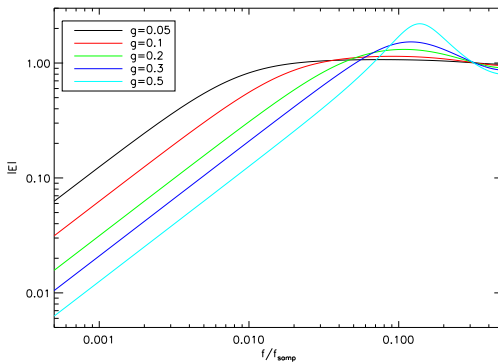
(a) Fonction de transfert de réjection.
