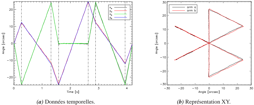
FIGURE 4.8 – Données temporelles des photocentres du FRAS lors de son étalonnage et représentation en XY de ces mêmes données.
