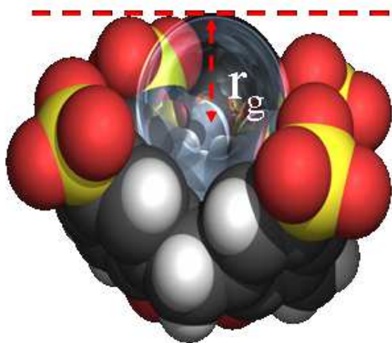
FIG. 2.3 – Visualisation de la cavité sphérique et du rayon de giration du calixarène.
