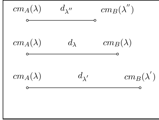
FIG. 5.2 – Cas où un seul centre de masse est déplacé. La légende est la même que celle utilisée sur la figure 5.1.
