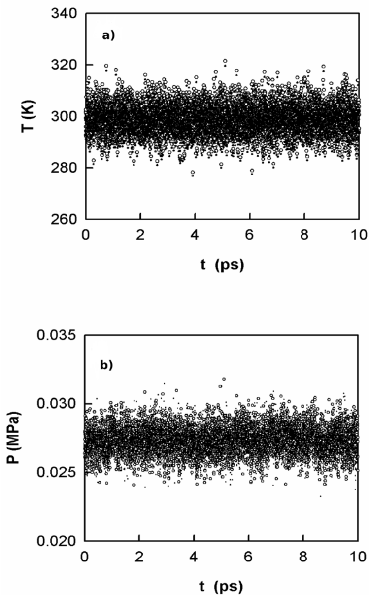
FIG. 4.5 – a) Température en fonction du temps pour les états \lambda' et \lambda . (○) représente la température instantanée dans l'état de référence. (●) représente la température instantanée dans l'état perturbé. b) Pression en fonction du temps pour les états \lambda' et \lambda . (○) représente la pression instantanée dans l'état de référence. (●) représente la pression instantanée dans l'état perturbé.
