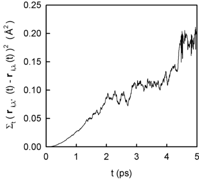
FIG. 4.3 – Trajectoire de la somme du carré de la différence des positions pour l'atome perturbé entre l'état perturbé (\mathbf{r}_{\lambda'}^i, \mathbf{p}_{\lambda'}^i) et l'état de référence (\mathbf{r}_{\lambda}^i, \mathbf{p}_{\lambda}^i) .
