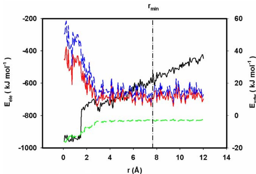
FIG. 5.10 – Interactions électrostatiques (—), dispersives (—), répulsives (—) et de dispersion-répulsion (—) entre le calixarène et l'ion \text{La}^{3+} en fonction de la distance séparant leurs centres de masse.
