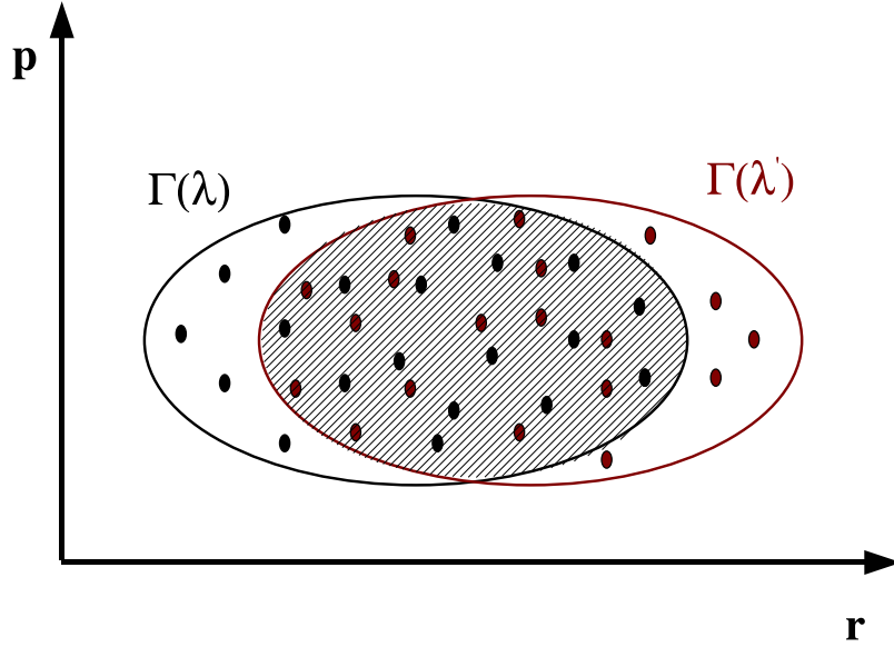
FIG. 4.2 – Recouvrement des espaces des phases entre l'état de référence et l'état perturbé. \Gamma(\lambda) est l'espace des phases de l'état de référence et \Gamma(\lambda') représente l'espace des phases parcourus de l'état perturbé. Les cercles indiquent les points d'intégration relatifs aux positions atomiques.
