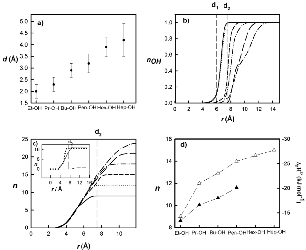
FIG. 3.4 – a) Moyenne de la distance entre le centre de masse du macrocycle et le centre de masse de d'alcool (de Et-OH à Hep-OH). b) Intégration de la distribution de distance entre le point cdm_{OH} (cf figure (3.3)) et le groupement OH de la molécule d'alcool (de Et-OH à Hep-OH). (—) Et-OH, (···) Pr-OH, (- - -) Bu-OH, (- · - ·) Pen-OH, (— — —) Hex-OH, (- · - ·) Hep-OH. c) Intégration de la distribution de distance entre chaque atome de la chaîne alkyle de la molécule d'alcool (de Et-OH à Hep-OH) et le point cdm_{OH} . On utilisera la même légende que la figure (3.4.b). La deuxième figure correspond à l'intégration de la distribution de distance (définie précédemment dans (a) et (b)) relative aux ions \text{La}^{3+} (— — —), \text{Me}_4\text{N}^+ (....) et à la molécule d'heptanol (- - -). d) ( \blacktriangle ) Variation d'enthalpie de complexation obtenue par microcalorimétrie représentée sur l'axe de droite. ( \Delta ) Nombre d'atomes insérés dans la cavité représenté sur l'axe de gauche.
