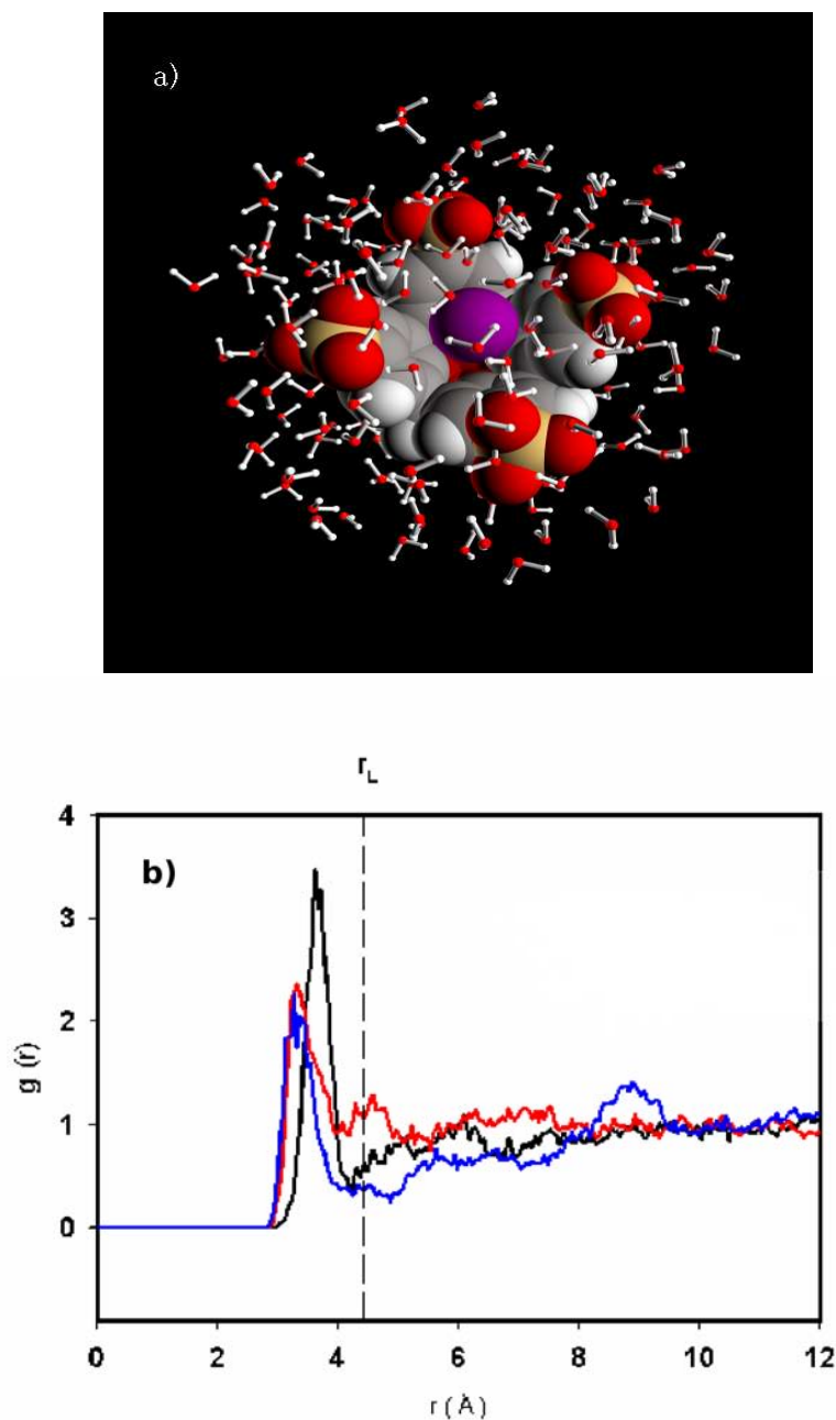
FIG. 6.1 – a) Visualisation du complexe dans le cluster d'eau. b) (—) Distribution radiale entre le centre de masse des groupements sulfonate et les atomes d'oxygène de l'eau. (—) Distribution radiale entre l'ion césium et les atomes d'oxygène de l'eau en présence du macrocycle et seul en solution (—). Ces distributions radiales correspondent au cas où la distance entre le calixarène et l'ion \text{Cs}^+ est de 2.0 Å. r_L indique la borne supérieure que l'on utilise dans notre critère de sélection.
