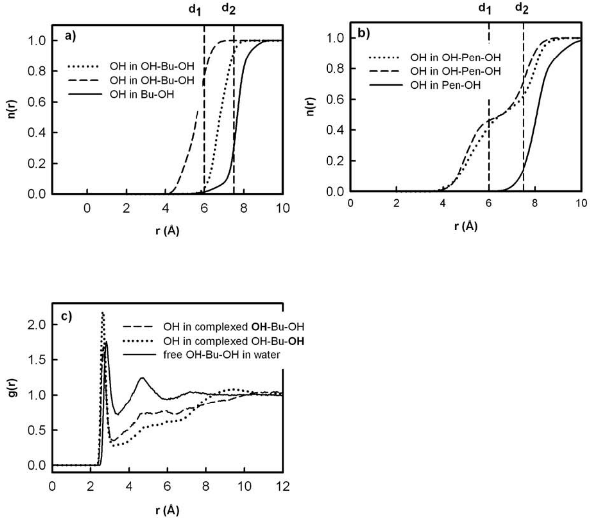
FIG. 3.9 – Intégration de la distribution de distance ( In_d : Abréviation utilisée pour représenter les intégration de distribution de distances) entre l'atome d'oxygène du groupement hydroxyde des diols et le centre de masse cdm_{OH} [ In_d ] (défini sur la figure (3.2)). In_d a été calculée pour les complexes impliquant le diol OH-Bu-OH (a) et le diol OH-Pen-OH (b). a) (—) In_d pour l'un des groupements OH dans le cas de la molécule OH-Bu-OH, (---) In_d pour le second groupement OH dans le cas de la molécule OH-Bu-OH, (...) In_d dans le cas de la molécule Bu-OH. b) (—) In_d pour l'un des groupements OH dans le cas de la molécule OH-Pen-OH, (---) In_d pour le second groupement OH dans le cas de la molécule OH-Pen-OH, (...) In_d dans le cas de la molécule Pen-OH. c) Distribution radiale entre l'atome d'hydrogène du groupement hydroxyde de la molécule OH-Bu-OH et les atomes d'oxygène des molécules d'eau (—) pour le premier groupement OH dans le cas du substrat en présence du complexe, pour le deuxième groupement OH dans le cas du substrat en présence du complexe (...) et dans le cas du substrat seul en solution (—).
