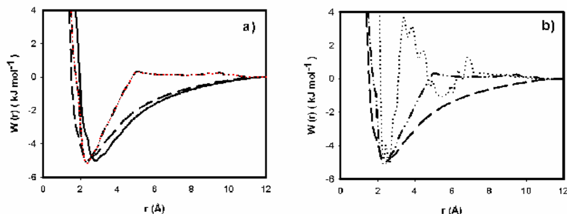
FIG. 5.4 – Profils de potentiel de force moyenne pour la paire d'ions [\text{Ca}^{2+} \cdots \text{SO}_4^{2-}] en phase gazeuse. a) FCS (— — —), FCFS (—), FEP (· · ·) et \text{FEP}^m (— · · —). b) FCS (— — —), \text{FEP}^m (— · · —) ainsi que la méthode PMFK (· · ·). La signification de ces acronymes est donnée dans le tableau (5.1).
