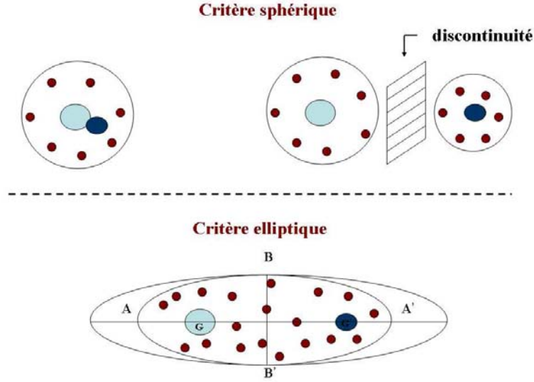
FIG. 6.2 – Visualisation des deux critères choisis pour déterminer l'ensemble qui sera traité en mécanique quantique. (●) et (●) représentent les centres de masse du calixarène et de l'ion \text{Cs}^+ . (●) représente les molécules d'eau. AA' = r^c + r^{\text{Cal}^{4-}} + r^{\text{Cs}^+} représente le grand axe de l'ellipse; BB' = r^{\text{Cal}^{4-}} + r^{\text{Cs}^+} représente le petit axe; r est la distance focale; G et G' sont les deux foyers de l'ellipse correspondant aux centres de masse du calixarène et de l'ion \text{Cs}^+ .
