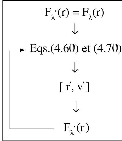
FIG. 4.4 – Schéma représentant le processus itératif pour le calcul de la force \mathbf{F}_{\lambda'}(\mathbf{r}_{\lambda'}^N) .
