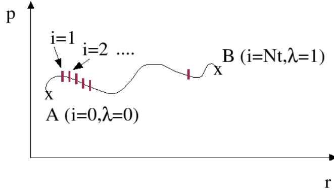
FIG. 4.1 – Schéma permettant de visualiser la décomposition du chemin thermodynamique entre les états A et B dans l'espace des phases. \lambda est le paramètre de couplage, i permet d'identifier chaque micro-état. Nt est le nombre total de subdivisions.
