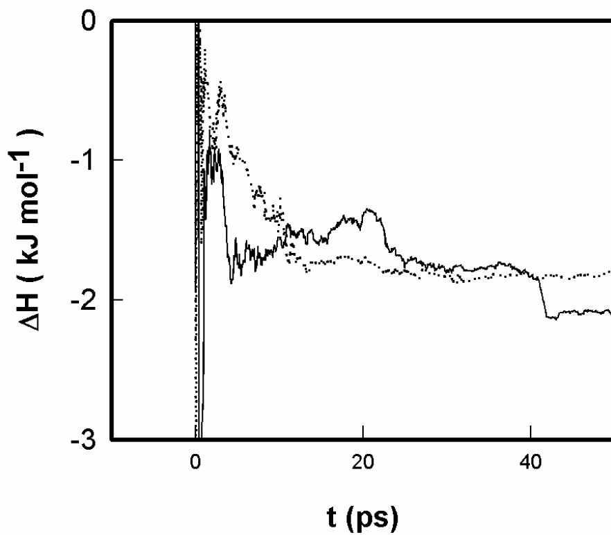
FIG. 4.10 – Variation d'enthalpie instantanée calculée pour la perturbation de \text{Ca}^{2+} en \text{Mg}^{2+} seul en solution ( \lambda=0.3 ). (—) est obtenue par les méthodes \mathcal{M}_I et FEP. ( \cdot \cdot \cdot ) est obtenue par les méthodes \mathcal{M}_{IV} et FEP.
