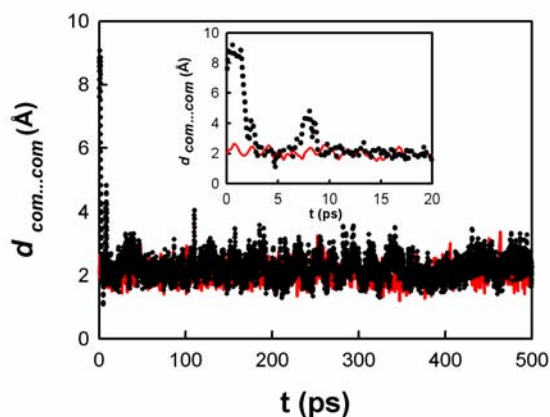
FIG. 3.2 – Distance entre le centre de masse du calixarène et celui du propanol en fonction du temps pour deux configurations initiales différentes. (···) correspond à la situation où les deux molécules sont éloignées de 10 Å. (—) représente la situation où les deux molécules sont proches l'une de l'autre.
