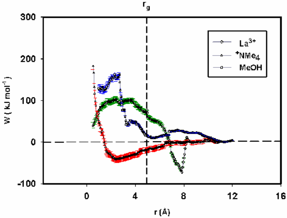
FIG. 5.8 – Profils de potentiel de force moyenne pour les paires d'ions : [\text{Ca}^{4-} \cdots \text{La}^{3+}] (—), [\text{Ca}^{4-} \cdots \text{Me}_4\text{N}^+] (—) et [\text{Ca}^{4-} \cdots \text{Me-OH}] (—). r_g représente la valeur du rayon de giration du macrocycle, que nous avons défini dans la section (2.6).
