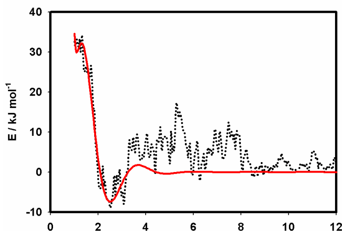
FIG. 6.3 – Ajustement de la différence d'énergie entre l'énergie moléculaire et l'énergie quantique. La différence a été ajustée par l'intermédiaire d'une fonction sinusoïdale amortie. (—) représente le résultat de l'ajustement et (···) représente la courbe à ajuster.
