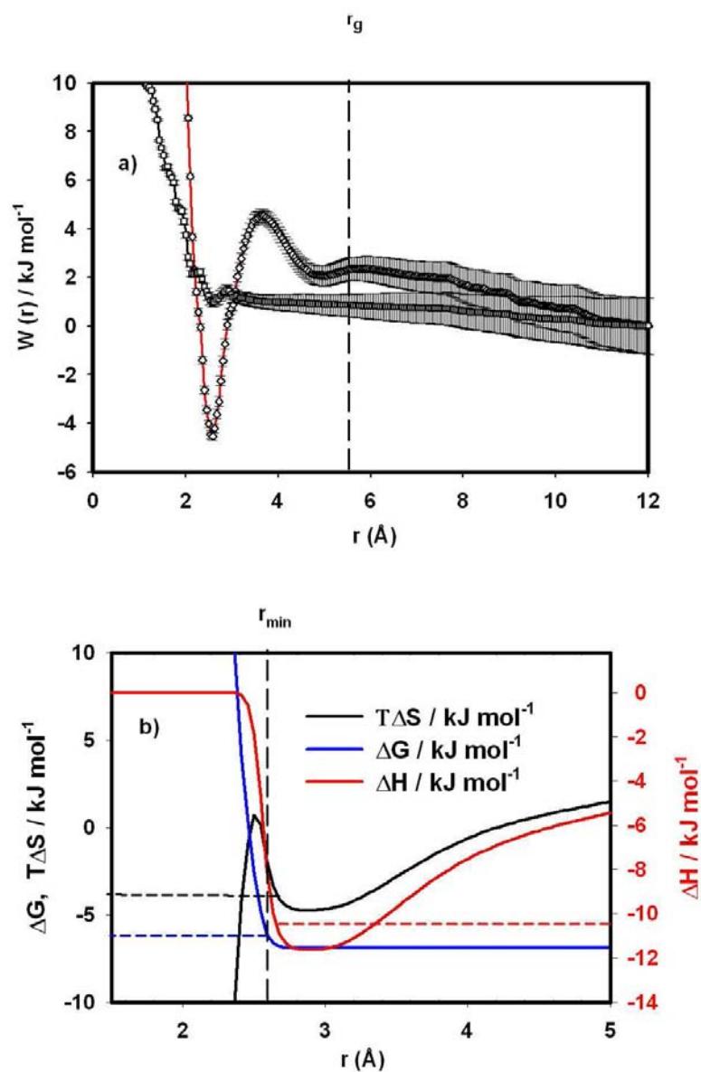
FIG. 6.4 – a) Potentiel de force moyenne corrigé ( \text{---}, \diamond ) et non corrigé ( \text{---}, \square ). b) Intégration des potentiels de force moyenne permettant de déterminer les grandeurs d'association en fonction de la valeur de la borne d'intégration. Les traits en pointillés représentent les valeurs obtenues par microcalorimétrie.
