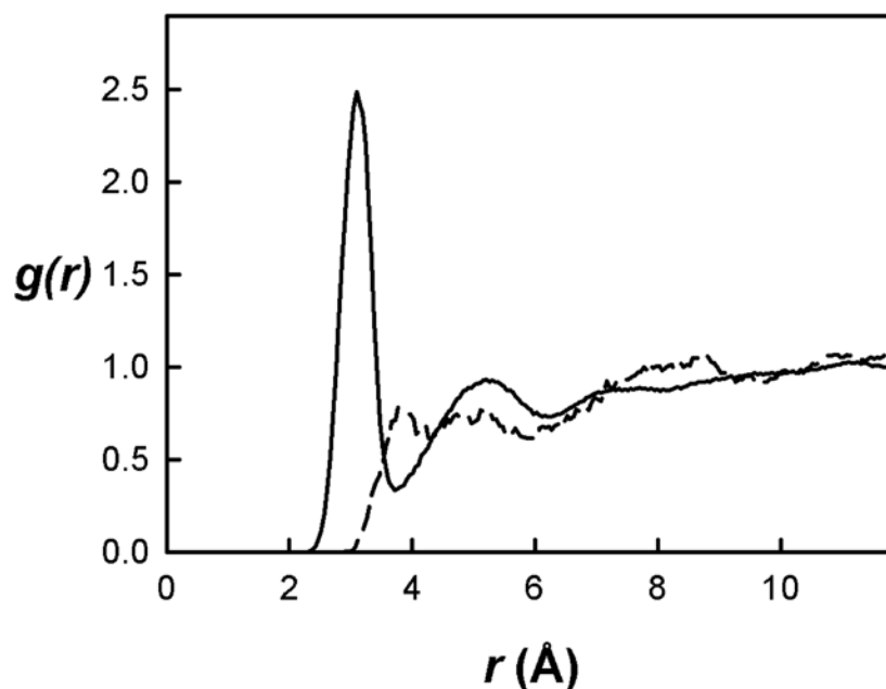
FIG. 3.8 – Distributions radiales entre le groupement OH du méthanol et les atomes d'oxygène de l'eau pour le méthanol seul (—) en solution et en présence du complexe (---).
