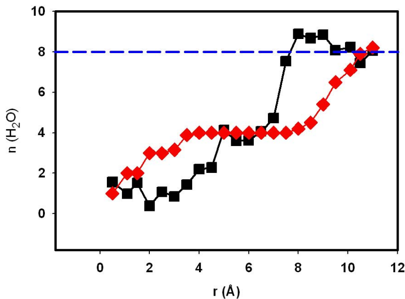
FIG. 5.12 – Nombre de molécules d'eau dans la première couche de solvation de l'ion \text{La}^{3+} (■) et dans la cavité (♦). La courbe (---) représente le nombre de molécules d'eau dans la première couche d'hydratation de l'ion lanthane pour l'ion seul en solution (8) et le nombre de molécules d'eau dans la cavité pour la calixarène seul en solution (8).
