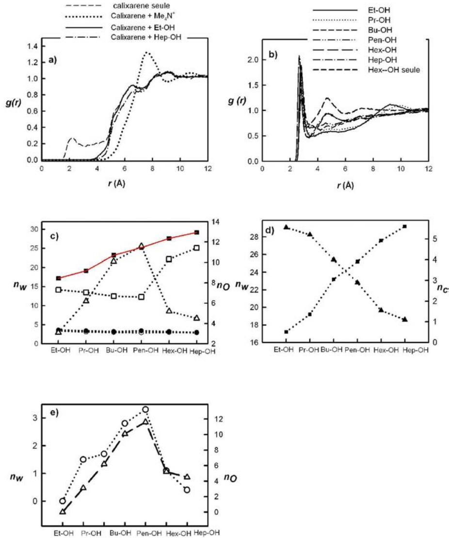
FIG. 3.5 – a) Distribution radiale entre le centre de masse du calixarène et les atomes d'oxygène des molécules ( g_{[\text{cdm}_{\text{Cal}4-}-\text{O}(\text{H}_2\text{O})]} ) d'eau (de Et-OH à Hep-OH) b) g_{[\text{OH}_{\text{Al}}-\text{O}(\text{H}_2\text{O})]} de Et-OH à Hep-OH. \text{OH}_{\text{Al}} représente le groupement hydroxyde de l'alcool. c) Nombre de molécules d'eau présentes dans la première couche de solvation du groupement OH de l'alcool seul en solution ( \bullet ) et de l'alcool en présence du complexe ( \circ ). ( \blacksquare ) Nombre de molécules d'eau présentes dans la seconde sphère d'hydratation pour l'alcool seul en solution, et en présence du calixarène ( \square ). ( \Delta ) Nombre d'atomes d'oxygène appartenant aux groupements sulfonate dans la deuxième couche de solvation du groupement OH de l'alcool représenté sur l'axe de droite. (—) Nombre total d'atomes d'oxygène (eau + sulfonate) dans la seconde sphère de solvation du groupement OH de l'alcool. d) ( \blacksquare ) Nombre de molécules d'eau présentes dans la seconde couche de solvation du groupe OH dans le cas des alcools seuls en solution, représenté sur l'axe de gauche. ( \blacktriangle ) Nombre d'atomes de carbone de la chaîne alkyle dans la seconde sphère de solvation du groupement OH, représenté sur l'axe de droite. e) ( \Delta ) Nombre d'atomes d'oxygène des groupements sulfonate dans la seconde sphère de solvation du groupe OH, représenté sur l'axe de droite ( \circ ) Nombre de ponts de liaisons hydrogène entre le groupe \text{SO}_3^- et l'alcool, représenté sur l'axe de gauche.
