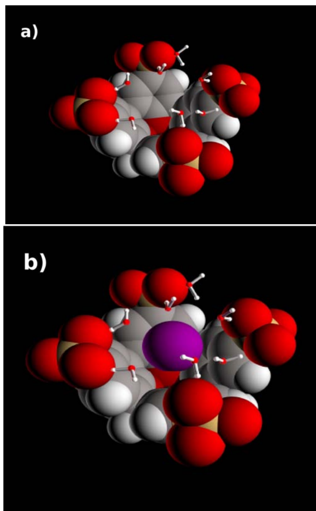
FIG. 6.6 – a) Visualisation de la désolvatation de la cavité. b) Visualisation de la solvatation de l'ion césium.
