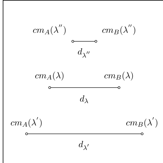
FIG. 5.1 – Schéma permettant de visualiser le déplacement des centres de masse de deux molécules dans le cas d'un élongation ( \lambda' ) de la distance intermoléculaire et dans le cas d'une diminution ( \lambda'' ) de cette distance. ( \lambda ) désigne le paramètre de couplage pour l'état de référence.
