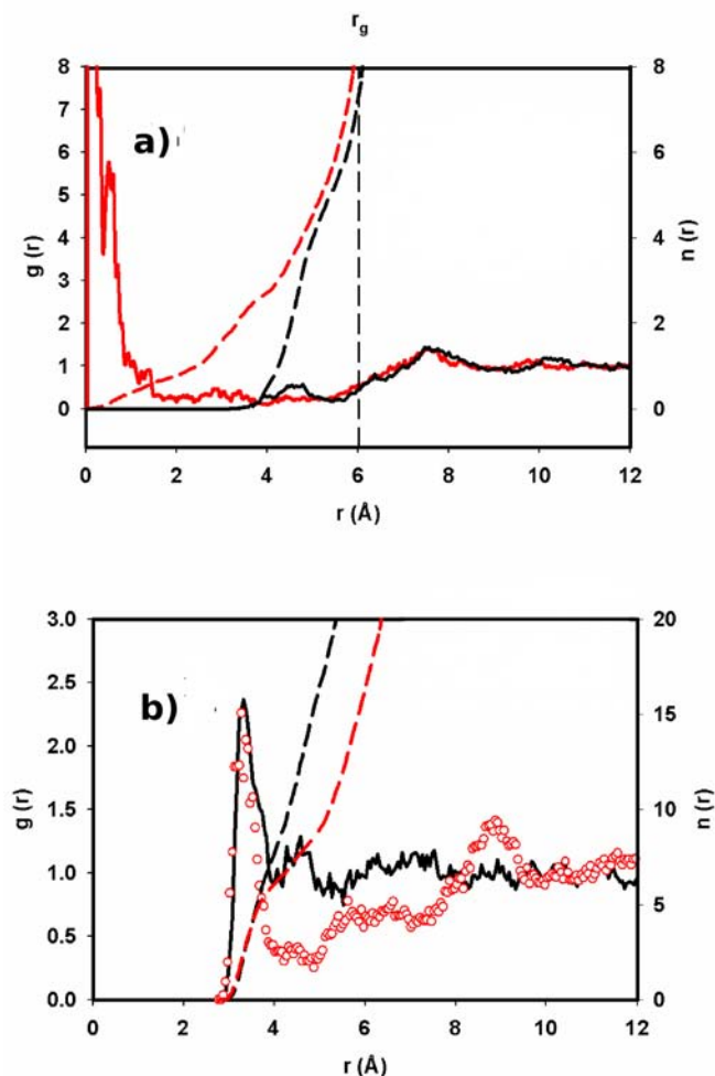
FIG. 6.5 – a) (—) Distribution radiale entre le centre de masse du macrocycle seul en solution et les atomes d'oxygène des molécules d'eau. (—) Distribution radiale entre le centre de masse du macrocycle en présence du complexe et les atomes d'oxygène de l'eau. r_g indique le rayon de giration du centre de masse du calixarène b) (—) Distribution radiale entre l'ion césium seul en solution les atomes d'oxygène des molécules d'eau. (—) Distribution radiale entre l'ion césium en présence du macrocycle les atomes d'oxygène des molécules d'eau. Sur les deux figures les courbes en pointillés représentent les courbes intégrales des distributions radiales (on utilise le même code de couleur que pour les distributions radiales).
