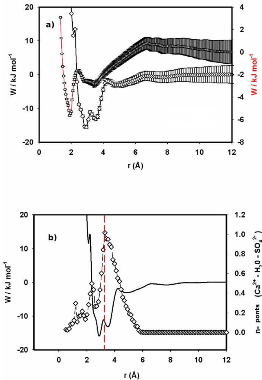
FIG. 5.5 – a) Profil de potentiel de force moyenne pour la paire d'ions [\text{Ca}^{2+} \cdots \text{SO}_4^{2-}] en phase gazeuse (—) représenté sur l'axe de droite. Profil de potentiel de force moyenne pour la paire d'ions [\text{Ca}^{2+} \cdots \text{SO}_4^{2-}] en phase aqueuse (—) représenté sur l'axe de gauche. b) (—) profil de potentiel de force moyenne en milieu aqueux représenté sur l'axe de gauche. ( \diamond ) nombre moyen de ponts de liaisons hydrogène pour le triplet [\text{Ca}^{2+}, \text{H}_2\text{O}, \text{SO}_4^{2-}] représenté sur l'axe de droite. La courbe (—) marque la valeur n_{\text{max}} défini comme le nombre maximal de ponts de liaisons hydrogène entre les ions \text{Ca}^{2+} et \text{SO}_4^{2-} et le puits de potentiel.
