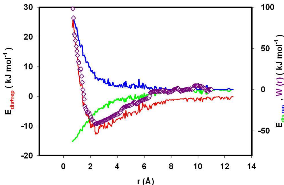
FIG. 5.13 – Interactions entre le calixarène et l'ion tétraméthylammonium en fonction de la distance séparant les centres de masse du macrocycle et du substrat. Les interactions dispersives (—) sont représentées sur l'axe de droite. Les interactions répulsives (—) sont représentées sur l'axe de droite. Les interactions de dispersion-répulsion (—) sont représentées sur l'axe de gauche. (◇) Potentiel de force moyenne entre le macrocycle et l'ion tétraméthylammonium représenté sur le premier axe de droite.
