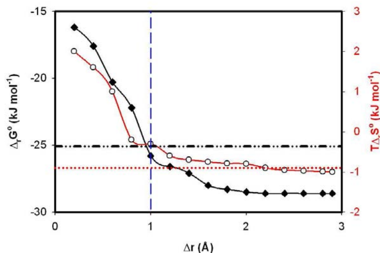
FIG. 5.9 – (—, ♦) évolution de \Delta_r G^\circ représentée sur l'axe de gauche en fonction de \Delta r tel que d_l = r_{min} + \Delta r . (—, ○) évolution de T\Delta_r S^\circ représentée sur l'axe de droite, en fonction de \Delta r . r_{min} est la position du puits de potentiel obtenue pour la paire [\text{Cal}^{4-} \cdots \text{Me}_4\text{N}^+] . La méthode utilisée pour calculer le potentiel de force moyenne est la méthode FEP m . (···) représente la valeur expérimentale de T\Delta_r S^\circ . (···) représente la valeur expérimentale de \Delta_r G^\circ . (---) indique la valeur de \Delta r utilisée pour le calcul des grandeurs d'association.
