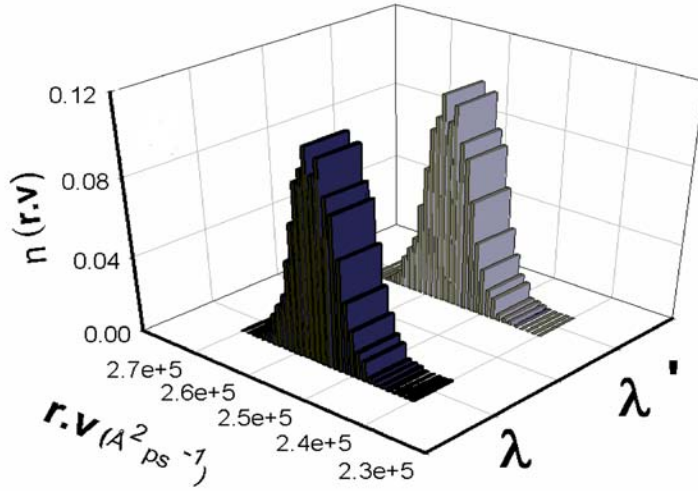
FIG. 4.7 – Distribution du produit \mathbf{r}_\lambda^N \mathbf{p}_\lambda^N pour les états \lambda et \lambda' .
