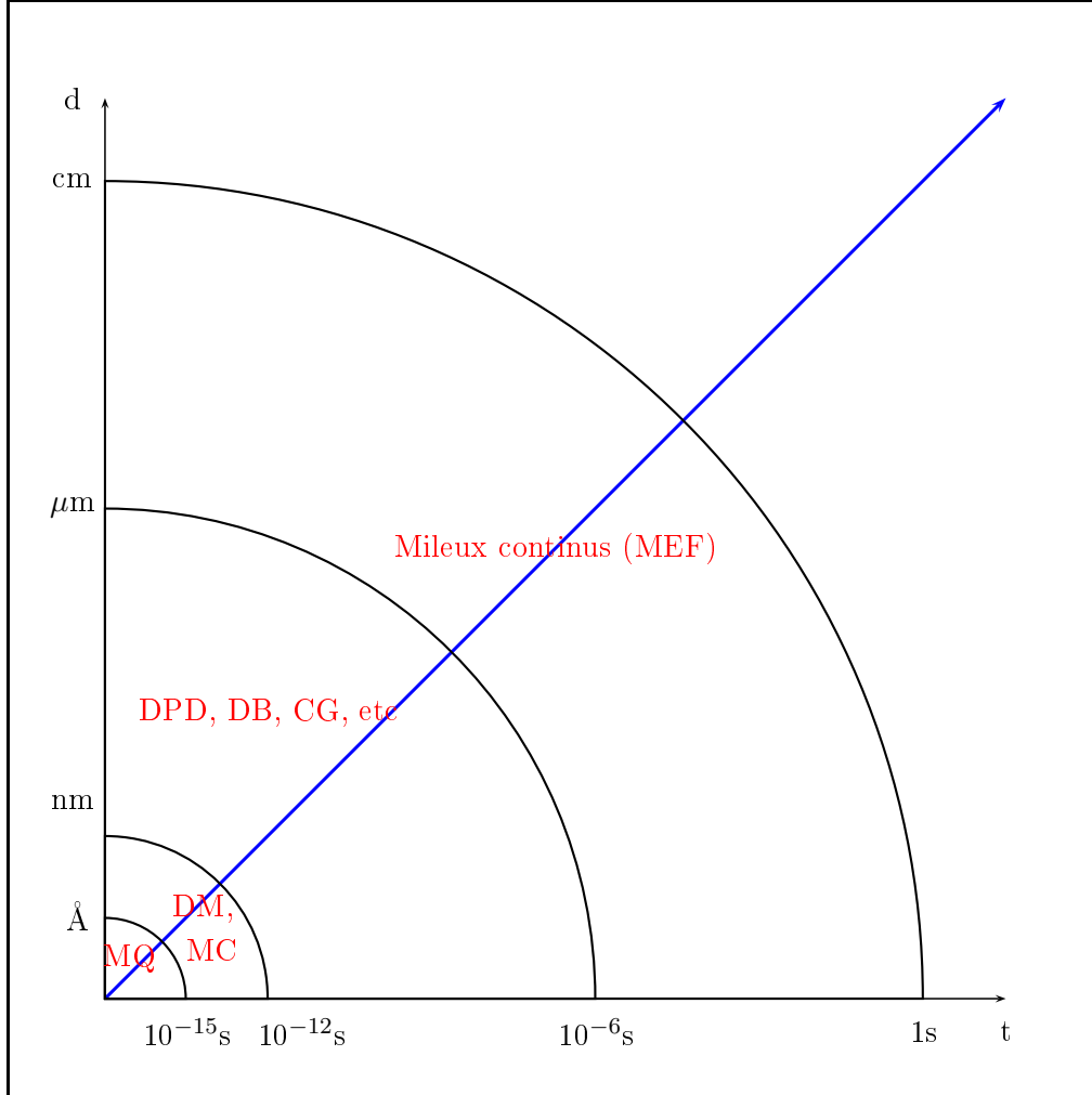
FIG. 2.1 – Méthodes de simulation utilisées en fonction de l'échelle spatiale ( d ) et temporelle ( t ). (MQ)=Mécanique quantique, (DM)=Dynamique moléculaire, (MC)=Monte Carlo, (DPD)=Dynamique des particules dissipatives, (DB)=Dynamique brownienne, (MEF)=Méthodes des éléments finis, (CG)= Coarse graining . ( \rightarrow ) indique le sens d'évolution dont il est question dans la discussion.
