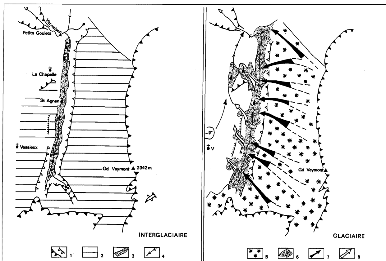
Figure II.67 - La "capture" par les écoulements superficiels des eaux météoriques appartenant à l'impluvium karstique, via les glaciers pléistocènes : exemple des Hauts-Plateaux et de la Vernaion
