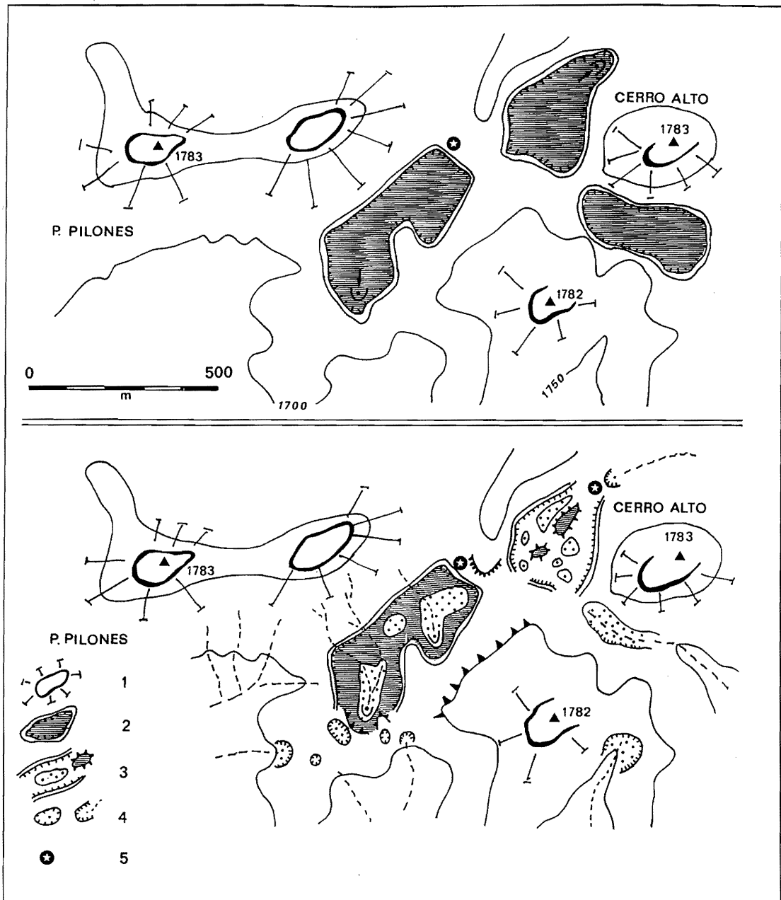
Figure III.102 - Évolution morpho-karstique des Hoyos de los Pilonos-Pilar
