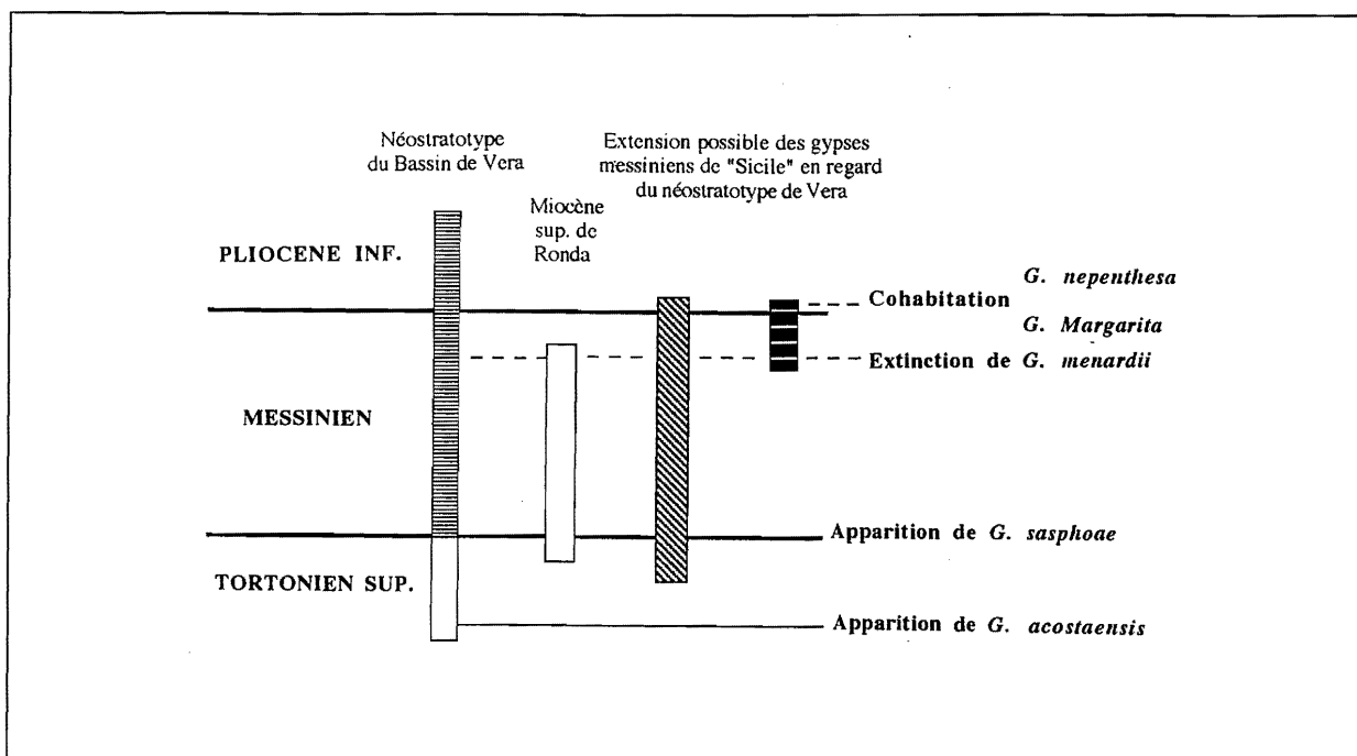
Figure III.14 - Les dépôts miocènes de Ronda au regard du Néostratotype de Cuevas de Almanzora (bassin de Vera, Levant espagnol)
