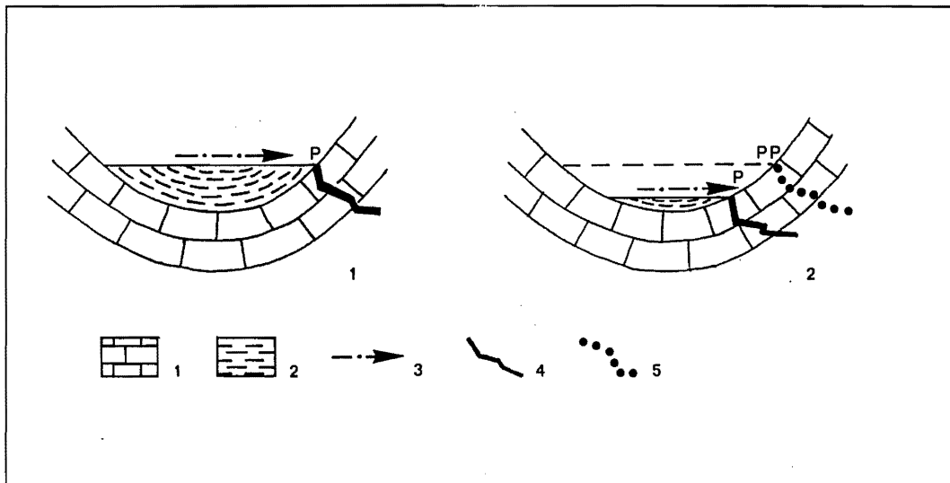
Figure I.5 - Exemples de l'incidence du dégagement d'une couverture lithologique partielle dans l'agencement d'un système karstique binaire s.l.
