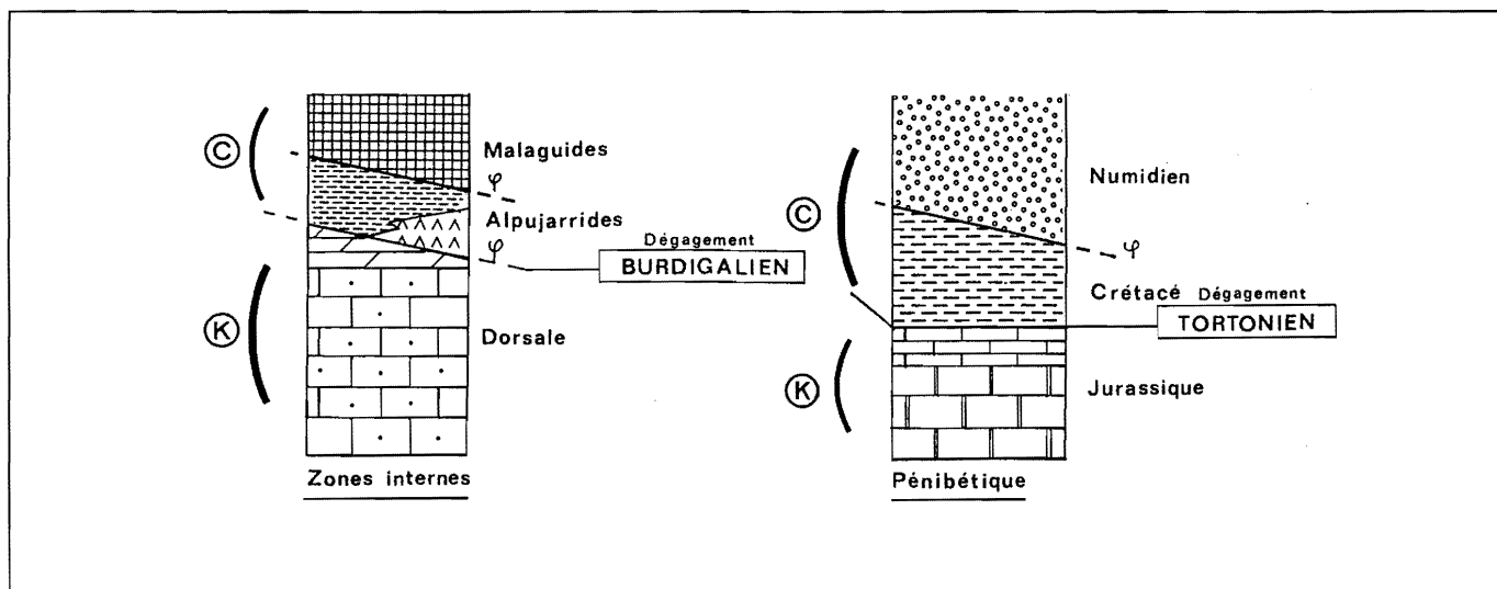
Figure III.27 - Les assises karstifiables des Serranías de Ronda et de Grazalema et leurs couvertures imperméables c : couverture; K : assises karstifiables.
