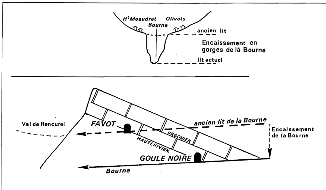
Figure II.81 - Étagement de la grotte Favot et de l'émergence de Goule Noire lié à l'encastement des gorges de la Bourne
