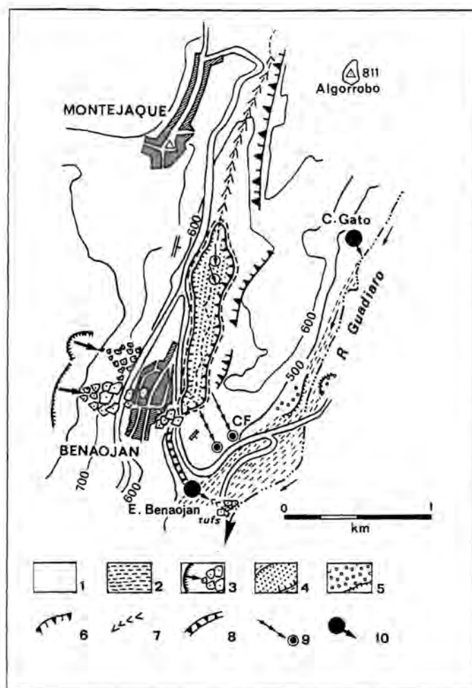
Figure III.89 - Carton morphologique du poljé de Benaoján
