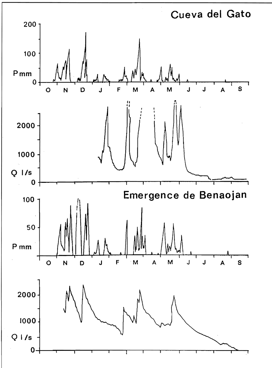
Figure III.44 - Relation précipitation-débit pour les émergences del Gato et de Benaojan. D'après A. Battle Gargallo et al. , 1986.
