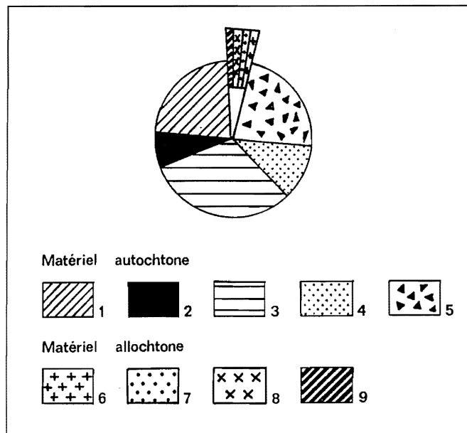
Figure II.16 - Comptage pétrographique des conglomérats sommitaux du synclinal de Pommiers-Romeyère.
