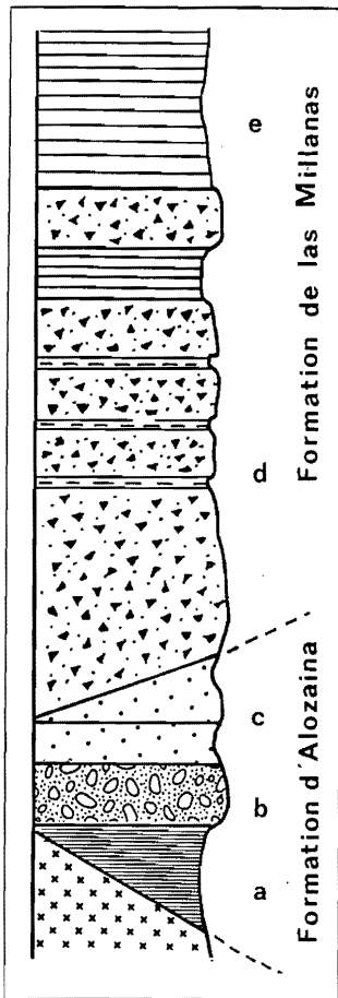
Figure III.5 - Échelle litho-stratigraphique des formations d'Alosaina et de las Millanas
