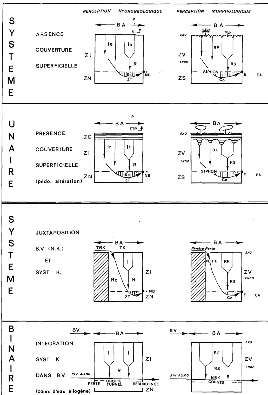
Figure I.1 - Les représentations hydrogéologiques et karstologiques d'une même entité : le système karstique. Expression schématique des systèmes unaires et binaires
