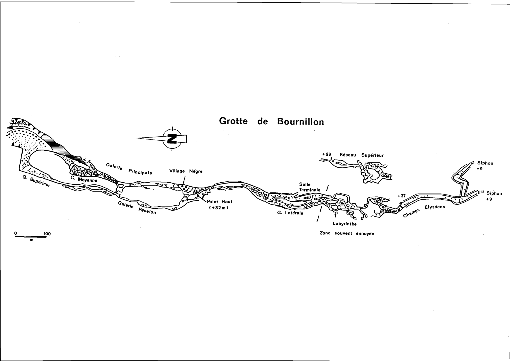
Figure II.110 - Plan morpho-spéologique de la grotte de Bournillon
