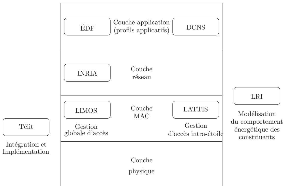
Figure 3.2 – Domaine d'intervention des différents acteurs sur la pile OCARI.
