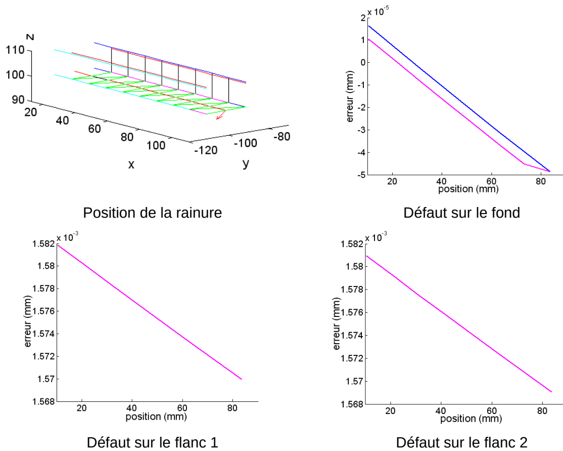
Figure 2-18 : Défauts lors d'une opération de rainurage sur la Verne
