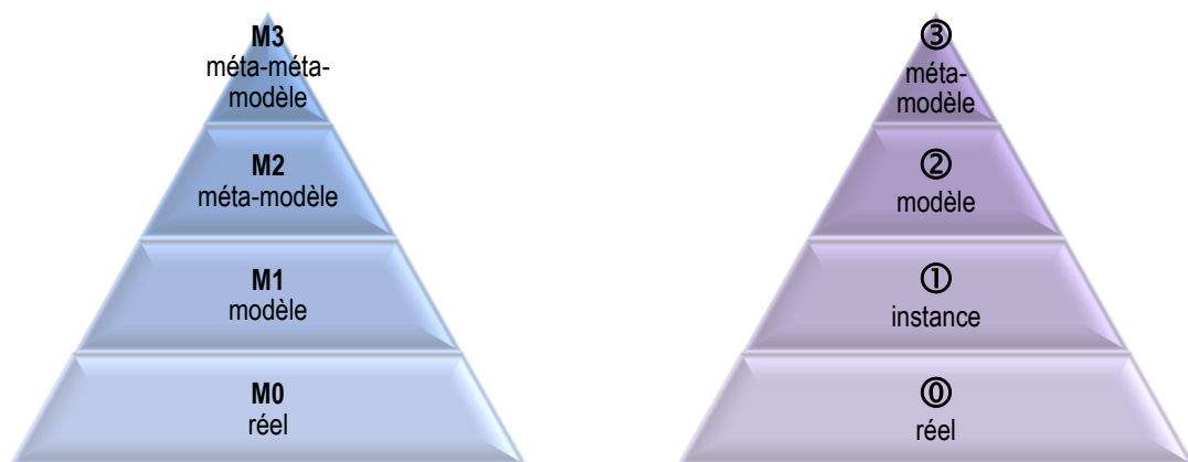
Figure 87 : Les quatre niveaux de modélisation de l'IDM. Figure 88 : Nos quatre niveaux de modélisation.
