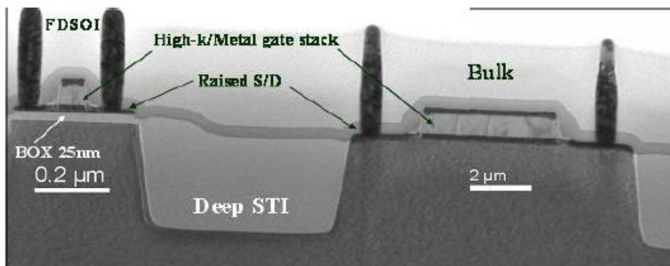
Figure 3.12. : Vue en coupe TEM de transistors MOS fabriqués sur la même puce en technologie planaire FDSOI BOX mince et sur silicium massif [Fenuillet'09].
