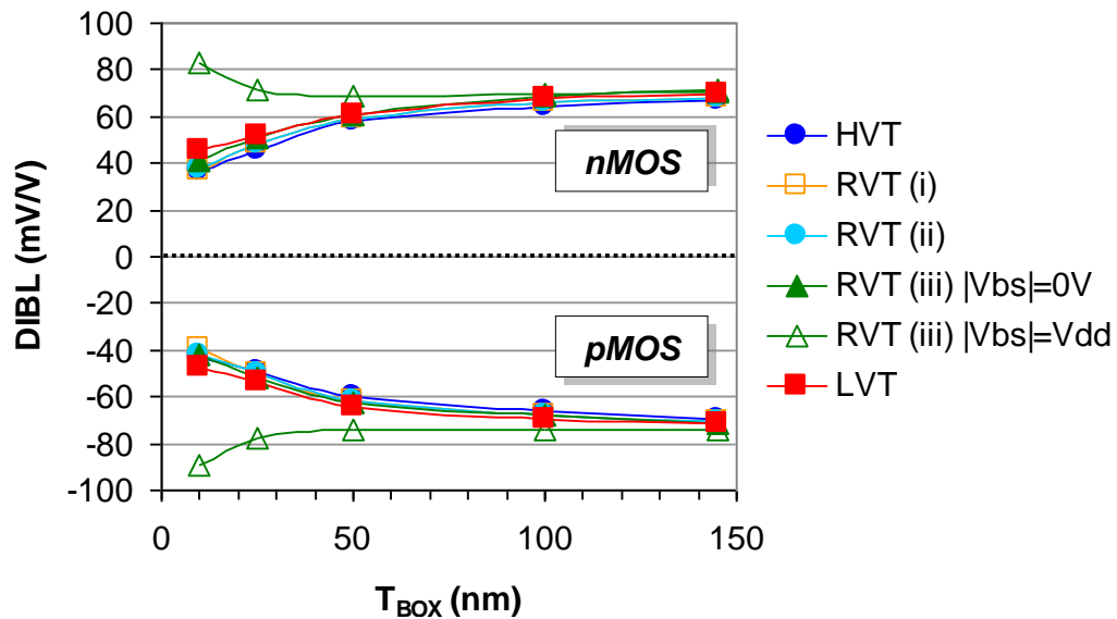
Figure 4.12. : Evolution du DIBL ( (V_{T\_in\_court} - V_{Tsat\_court}) / (V_{DD} - 50 \text{ mV}) ) en fonction de T_{BOX} pour plusieurs options de V_T d'un transistor nMOS et d'un transistor pMOS FDSOI à canal court ( L_G=30 nm) et ayant un film mince de silicium non dopé d'une épaisseur T_{Si}=6 nm, un oxyde de grille avant d'une épaisseur T_{OX}=1,2 nm et une tension d'alimentation V_{DD}=0,9 V.
