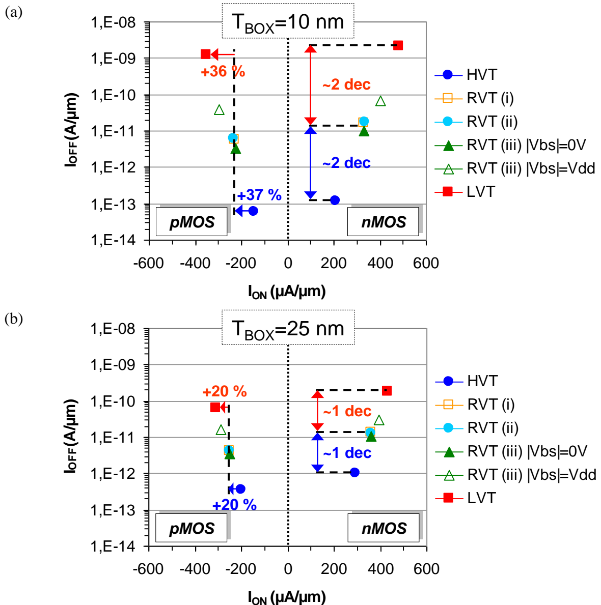
Figure 4.25. : Evolution du courant I_{OFF} en fonction du courant I_{ON} pour différentes options de V_T d'un transistor nMOS et d'un transistor pMOS FDSOI à canal court ( L_G=30 nm) et ayant un film mince de silicium non dopé d'une épaisseur T_{Si}=6 nm, une épaisseur d'oxyde de grille avant T_{OX}=1,2 nm et une tension d'alimentation V_{DD}=0,9 V avec une épaisseur de BOX (a) T_{BOX}=10 nm et (b) T_{BOX}=25 nm.
