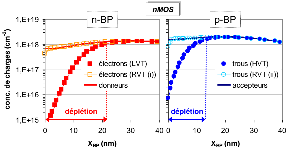
Figure 4.19. : Evolution de la concentration de charges en fonction de la profondeur du BP ( X_{BP} ) lorsque V_{GS}=V_T pour plusieurs options de V_T d'un transistor nMOS FDSOI à canal long ( L_G=1 \mu m ) et ayant un film mince de silicium non dopé d'une épaisseur T_{Si}=6 \text{ nm} , un oxyde de grille avant d'une épaisseur T_{OX}=1,2 \text{ nm} , un BOX d'une épaisseur T_{BOX}=10 \text{ nm} et une tension d'alimentation V_{DD}=0,9 \text{ V} .
