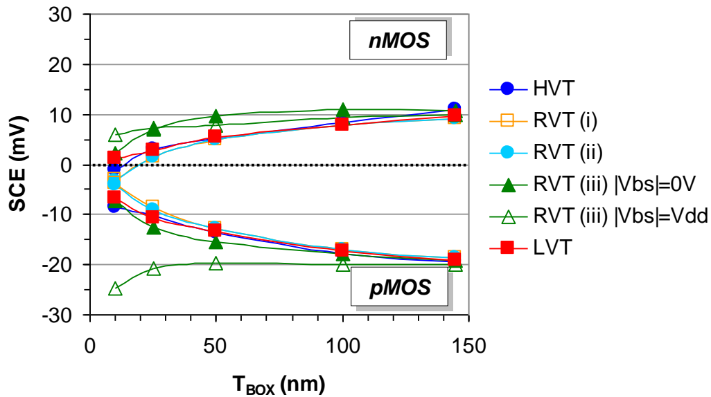
Figure 4.11. : Evolution des effets canaux courts ( SCE = V_{T\_long} - V_{T\_in\_court} ) en fonction de T_{BOX} pour plusieurs options de V_T d'un transistor nMOS et d'un transistor pMOS FDSOI ayant un film mince de silicium non dopé d'une épaisseur T_{Si}=6 nm, un oxyde de grille avant d'une épaisseur T_{OX}=1,2 nm et une tension d'alimentation V_{DD}=0,9 V.
