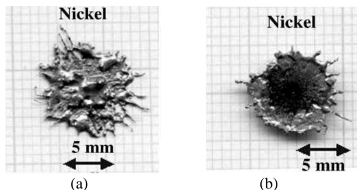
Figure 1.11. Morphologie de lamelles de nickel projetées sur un substrat en acier inoxydable : (a) T = 300\text{ K} , (b) T = 673\text{ K} [42]
