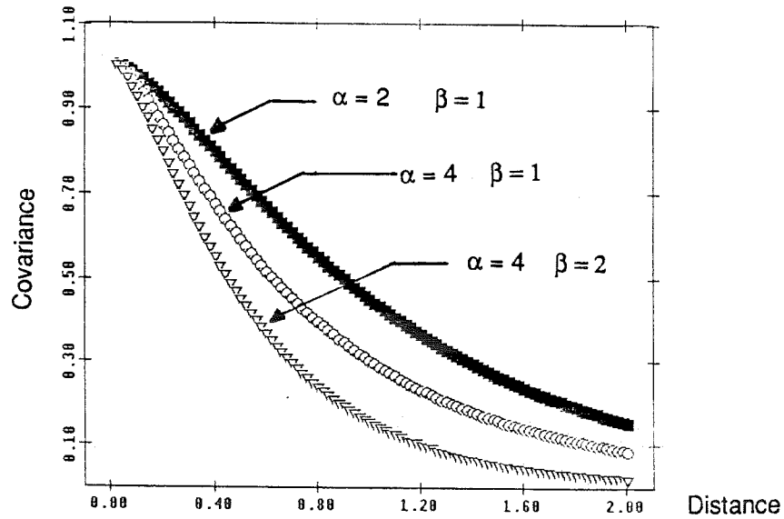
Fig 2-1: Modèle de covariance proposé par Fortus (1975):
