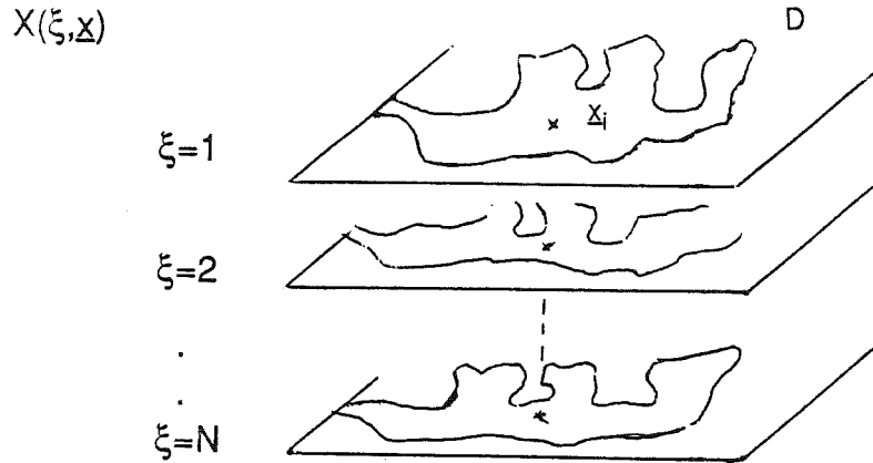
Fig. 1-2: Echantillonnage spatial du processus X(\xi, x) sur un domaine borné D , dans un contexte de multiréalisations.
