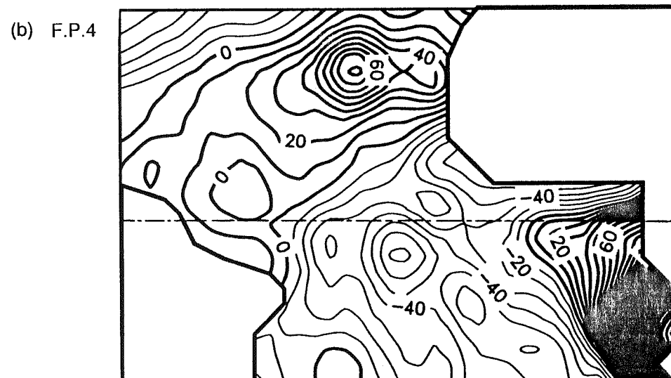
Fig. 4-24: F.P. calculées sur le réseau aléatoire, à gauche par ACP classique, à droite par ACPP. (a) F.P. 3 (b) F.P. 4.
