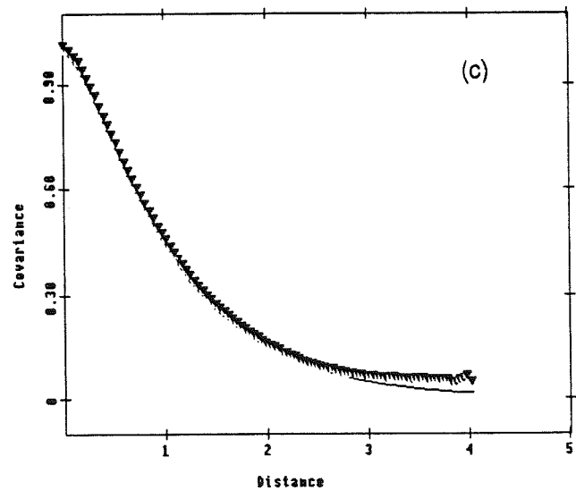
Fig. 2-13: Covariances théoriques ----- et expérimentales ▼ d'un jeu de N réalisations simulées par Bandes tournantes. (a) N=100 , (b) N=300 , (c) N=1000 .
