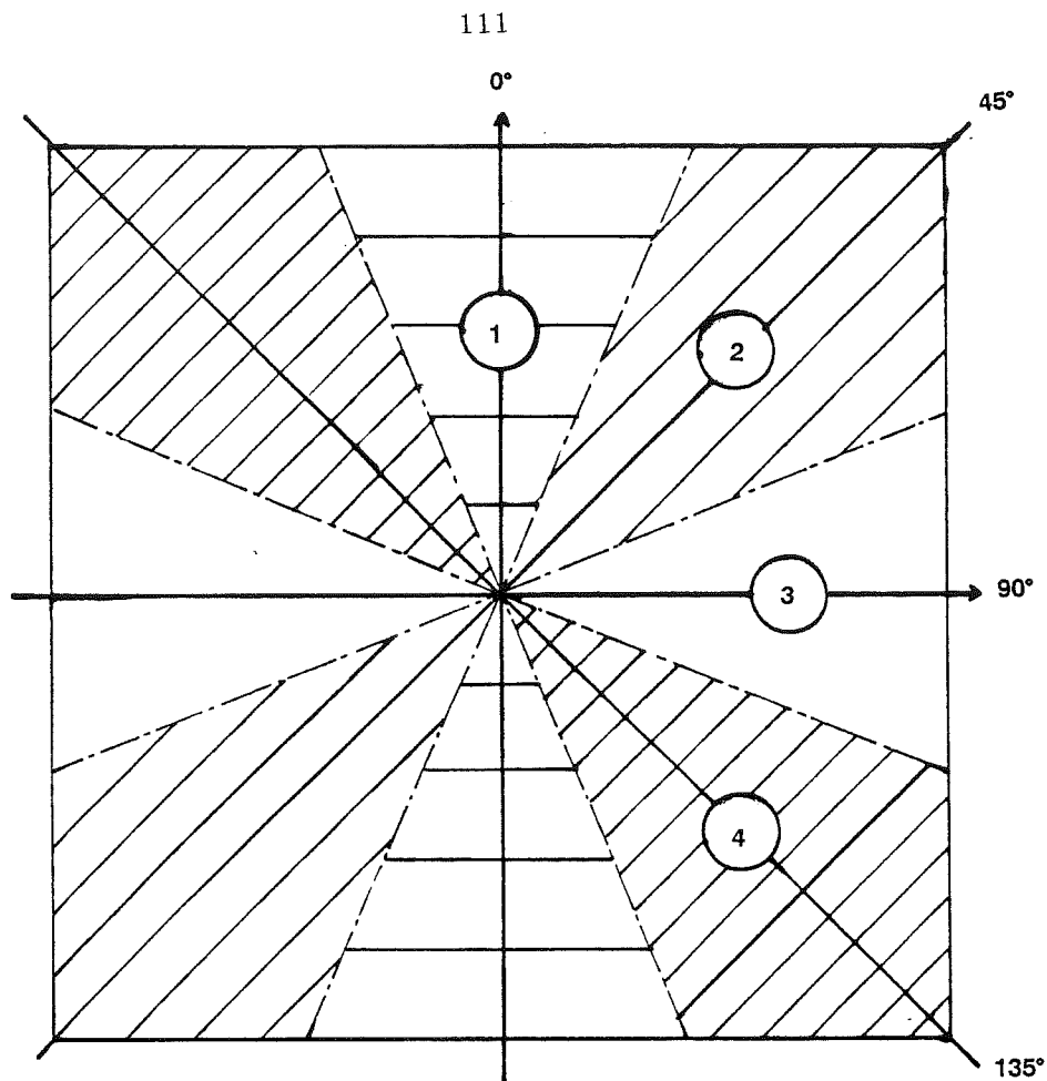
Fig. 3-17: Les différentes directions retenues pour le calcul des variogrammes par azimut.
