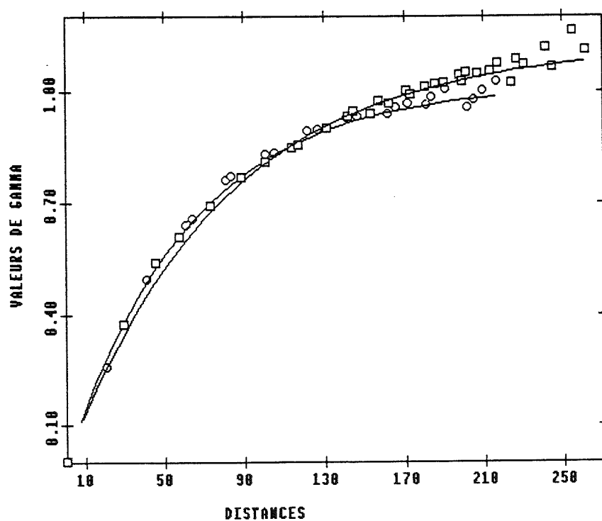
Fig. 3-18: Variogrammes climatologiques globaux bruts et modélisés, les données étant simulées par ACP.
