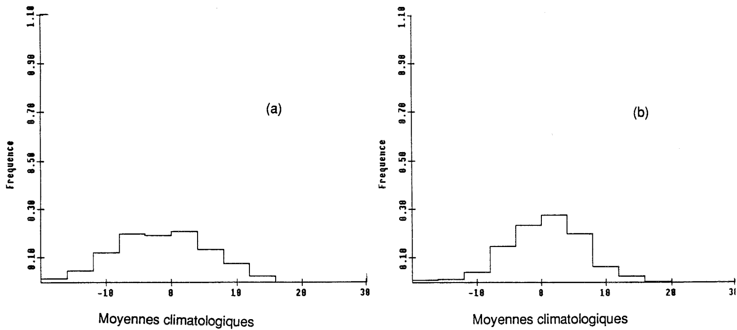
Fig. 3-12: Histogramme des moyennes climatologiques avec des distributions des Z_k(\xi)
