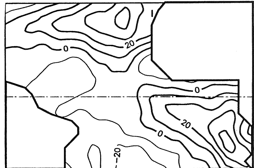
Fig. 4-24: F.P. calculées sur le réseau aléatoire, à gauche par ACP classique, à droite par ACPP. (a) F.P. 3 (b) F.P. 4.
