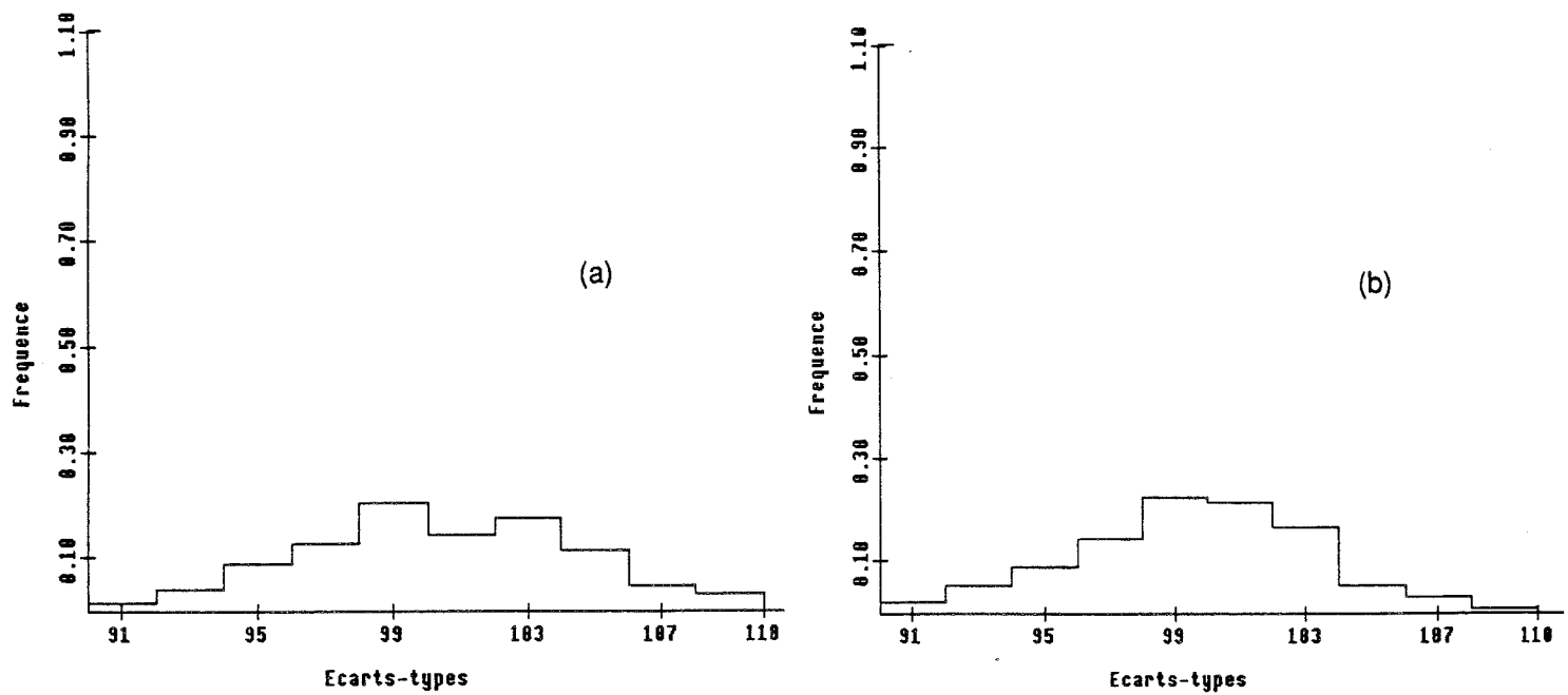
Fig. 3-13: Histogramme des écart-types climatologiques avec des distributions des Z_k(\xi)
