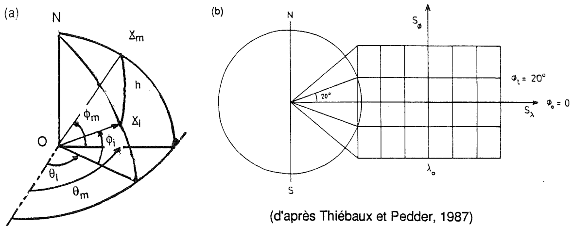
Fig. 4-7: (a) Définition de la longitude et de la latitude (θ, φ) ainsi que de la distance sur la sphère
