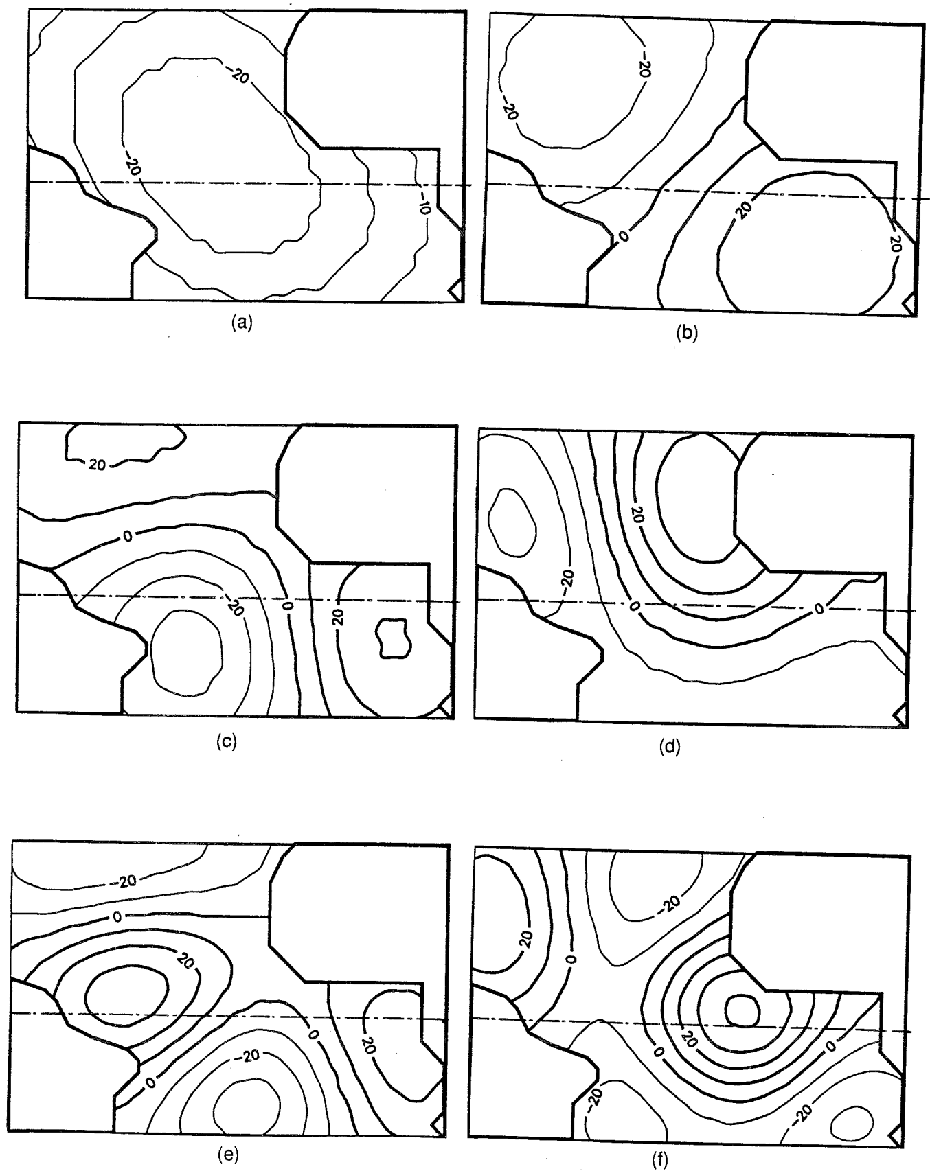
Fig. 4-26: Fonctions propres calculées par ACPP (LPF) de la SST désaisonnalisée en remplissant la matrice de covariance C à l'aide du modèle:
