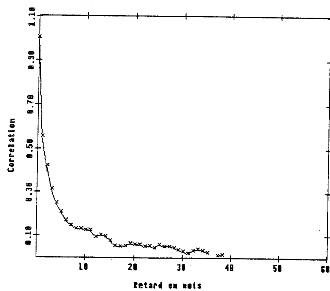
Fig. 4-6: Corrélogramme de l'ensemble du fichier des SST désaisonnalisées.
