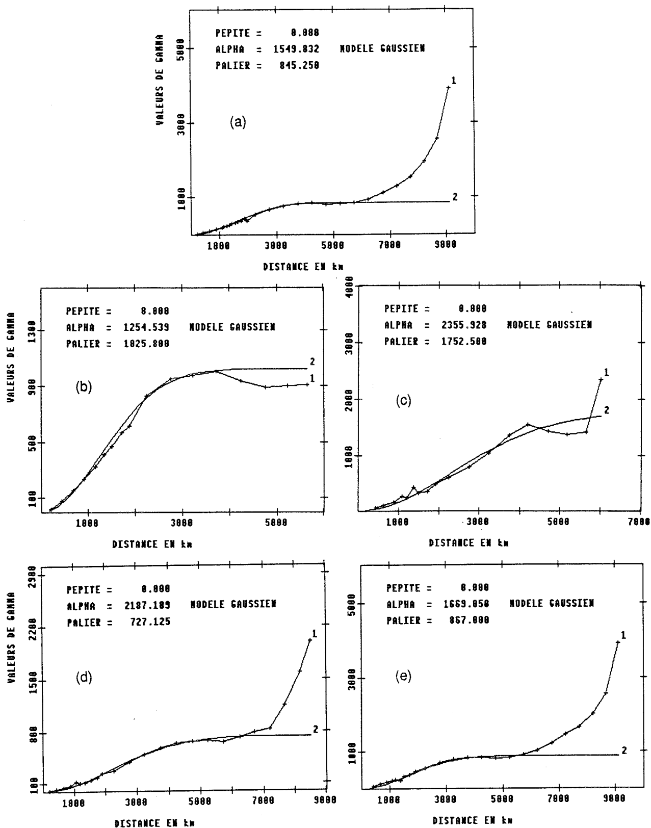
Fig. 4-9: Variogrammes climatologiques de la SST brute calculés sur l'ensemble du domaine.
