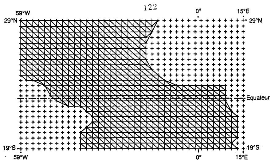
Fig. 4-1: Discretisation du domaine d'étude (grille de 2° par 2° entre 19°S et 29°N et 59°W et 15°E)
