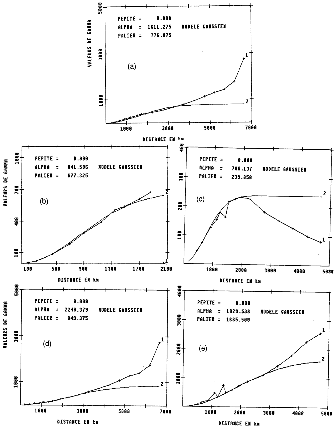
Fig. 4-11: Variogrammes climatologiques de la SST brute calculés sur l'hémisphère Sud.
