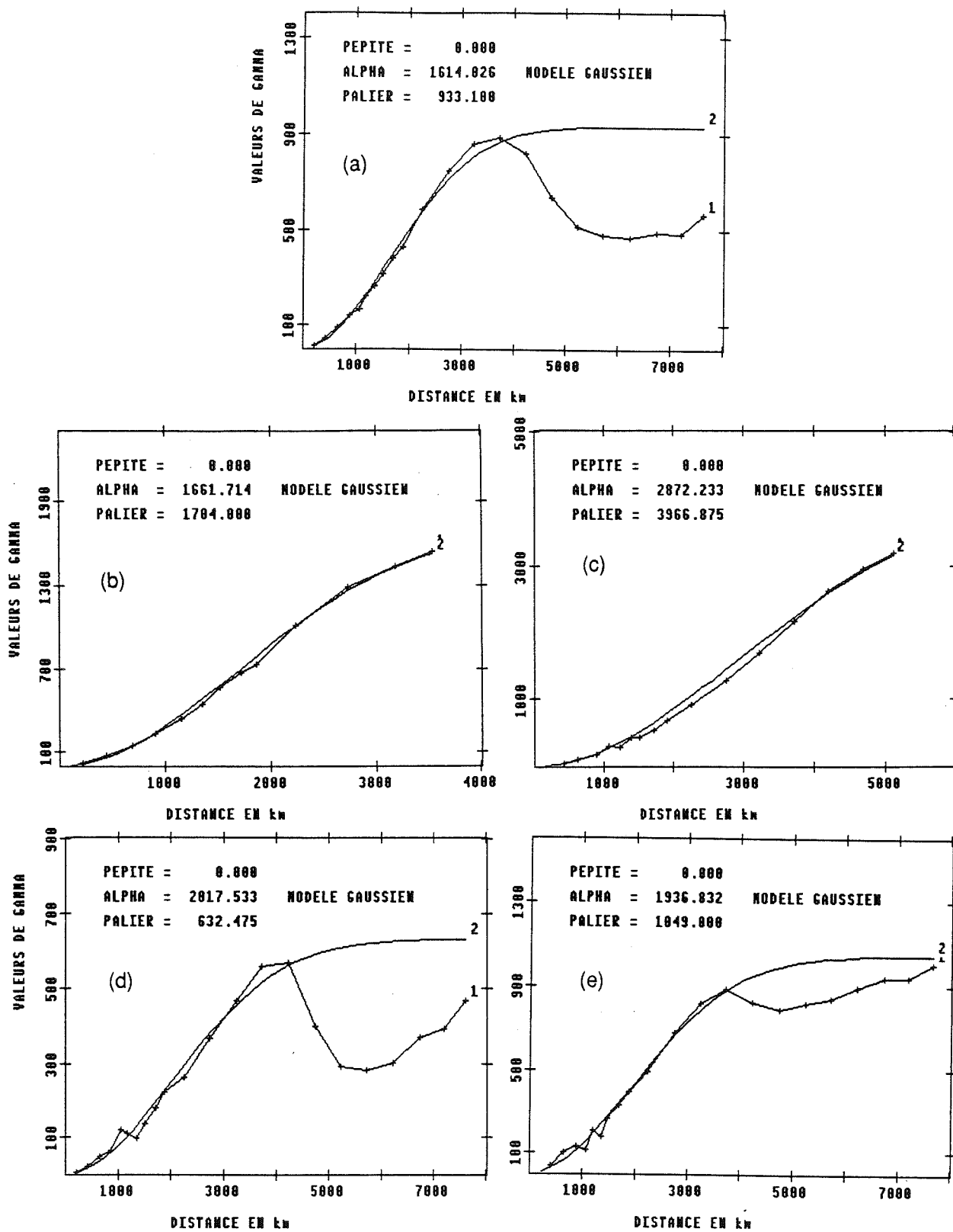
Fig. 4-10: Variogrammes climatologiques de la SST brute calculés sur l'hémisphère Nord.
