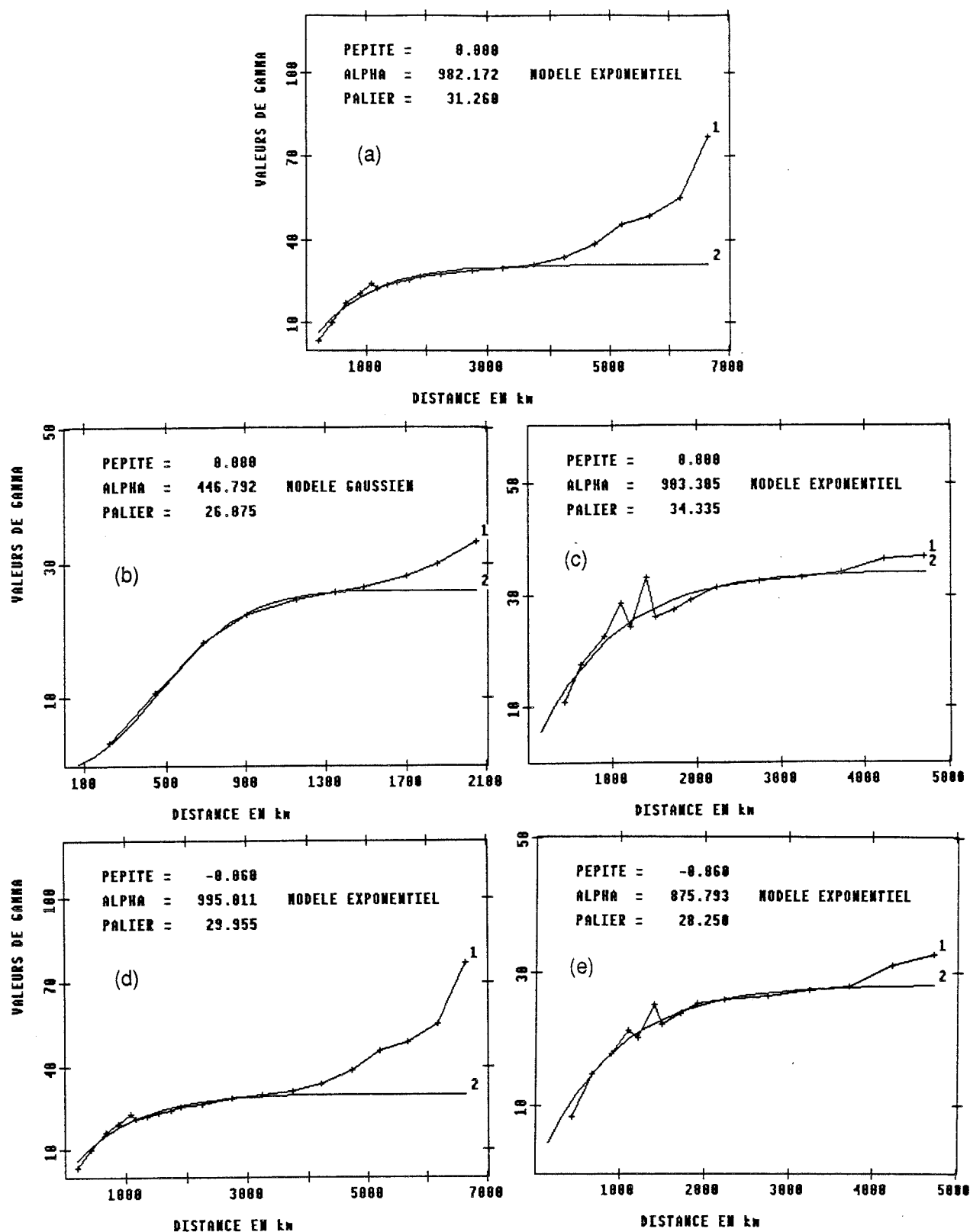
Fig. 4-14: Variogrammes climatologiques de la SST désaisonnalisée calculés sur l'hémisphère Sud.
