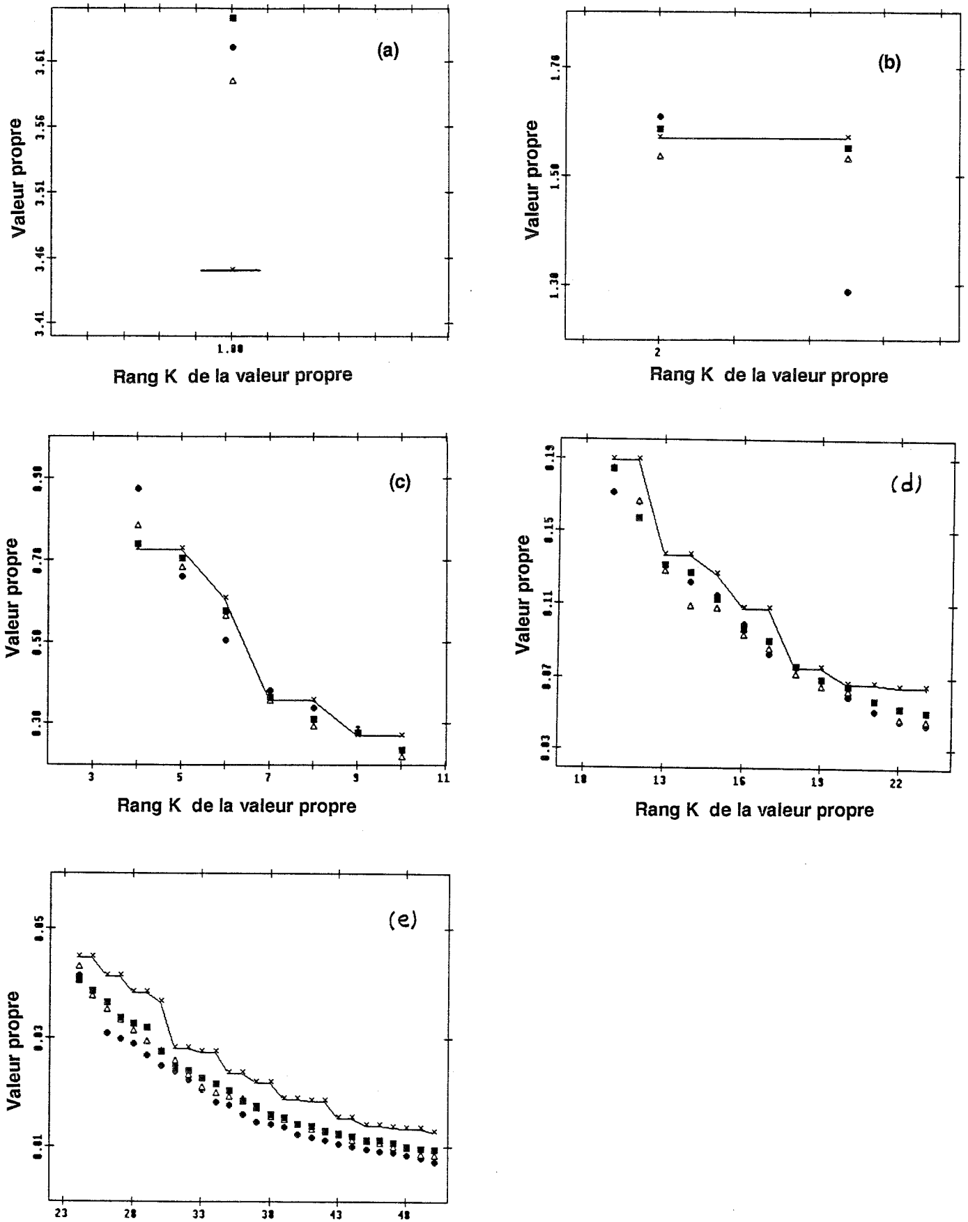
Fig. 2-10: Valeurs propres en fonction de leur rang K ( R=2 , \alpha=2 , \beta=1 ) selon la taille N de l'échantillon. (Attention : les échelles des diverses figures sont différentes).
