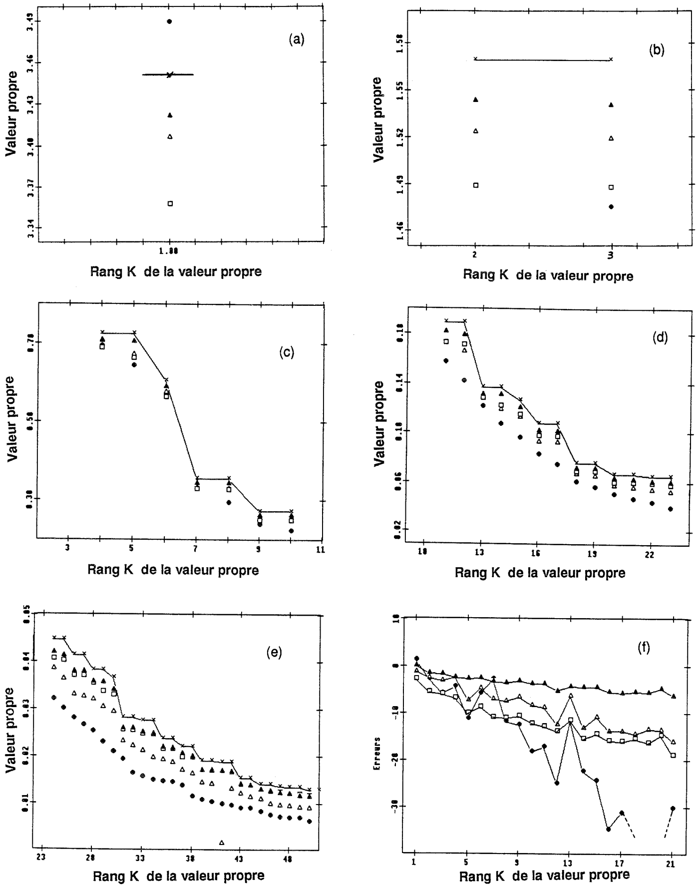
Fig. 2-4: Valeurs propres en fonction de leur rang K ( R=2 , \alpha=2 , \beta=1 ) selon la densité P du réseau. (Attention : les échelles des diverses figures sont différentes).
