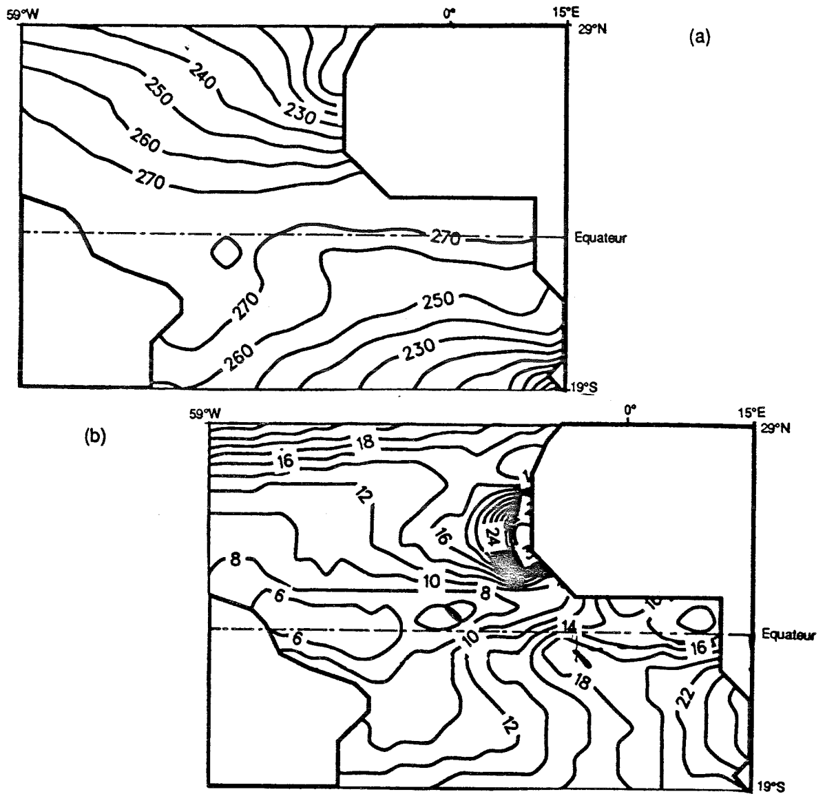
Fig. 4-3: Moyenne (a) et écart-type (b) climatologiques (tous mois et toutes années confondus) de la SST brute sur la période 1964-1985. (SST en 1/10^{\circ}\text{C} )
