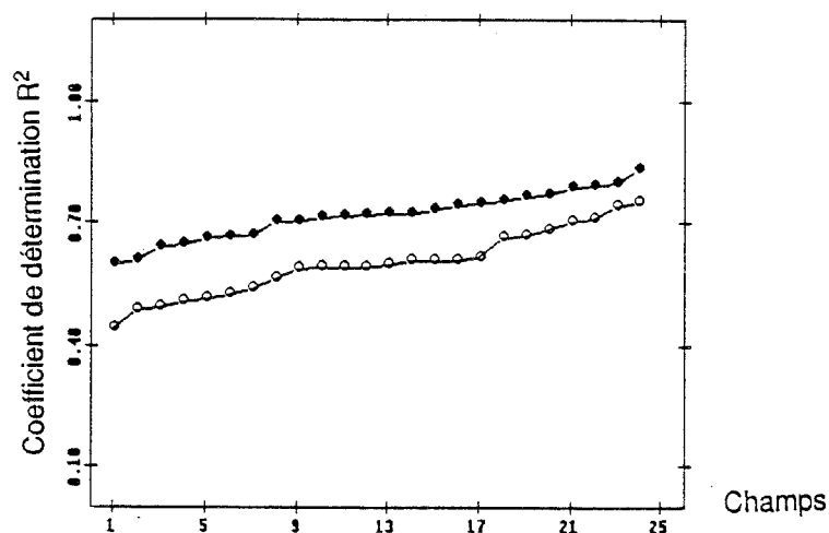
Fig. 4-27: Courbe d'efficacité (coefficient de détermination R^2(t_i, \xi_i) classés) des 24 champs reconstitués par ACPP des données de 1964 à 1985 en LPF.
