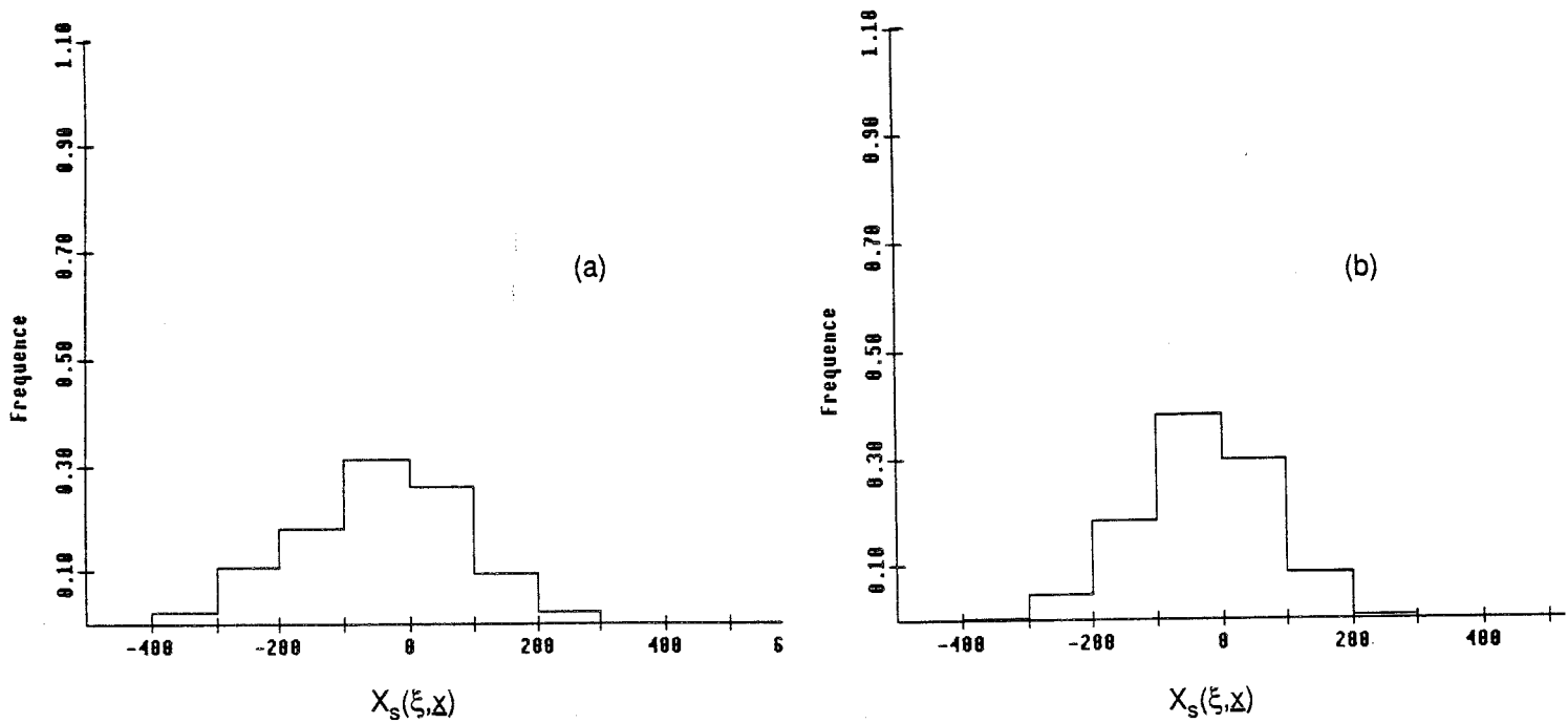
Fig. 3-11: Histogramme de X_s(\xi, \Delta) pour le champ 114 avec des distributions des Z_k(\xi) (a) gaussiennes, (b) uniformes
