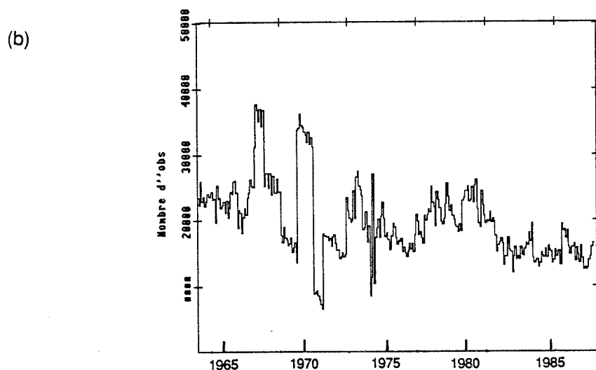
Fig 4-2: (a) Nombre moyen d'observations mensuelles par boîte de 5° par 2°. (b) Nombre total d'observations par mois.
