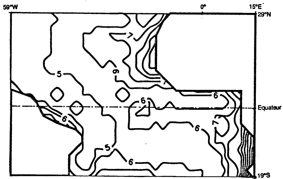
Fig. 4-4: Ecart-type climatologique (tous mois et toutes années confondus) des SST désaisonnalisées sur la période 1964-1987. (SST en 1/10^{\circ}\text{C} )
