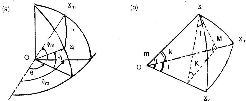
Fig. C-2: (a) Définition de la longitude et de la latitude ( \theta_i, \phi_i ) d'un point x_i (b) Représentation des côtés ( i, m, k ) et des angles ( I, M, K ) d'un triangle sphérique qui sont respectivement les faces et les dièdres d'un trièdre.
