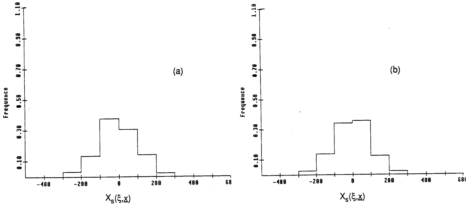
Fig. 3-10: Histogramme de X_s(\xi, \Delta) pour la station 42 avec des distributions des Z_k(\xi) (a) gaussiennes, (b) uniformes
