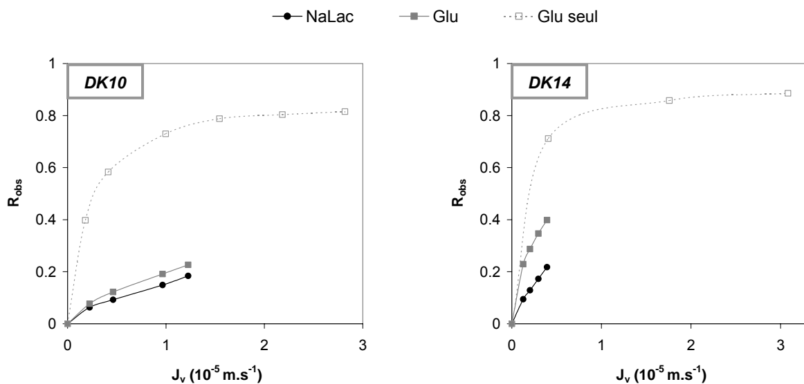
Figure IV-18 . Mélange glucose / lactate de sodium - Rétentions observées - v_t = 1.3 m \cdot s^{-1} - [Glu] = 0.1 M - [NaLac] = 1 M - Membranes DK10 et DK14
