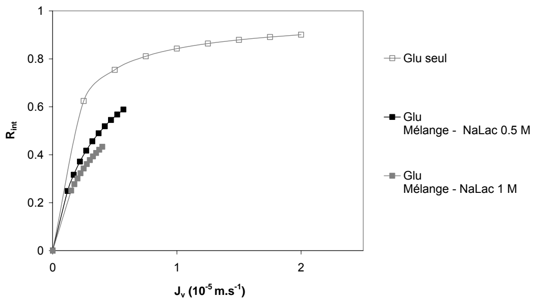
Figure IV-11 . Mélange glucose / lactate de sodium - Rétention intrinsèque du glucose - Influence de la concentration initiale en lactate de sodium - Membranes DK14 - [Glu] = 0.1\text{ M}
