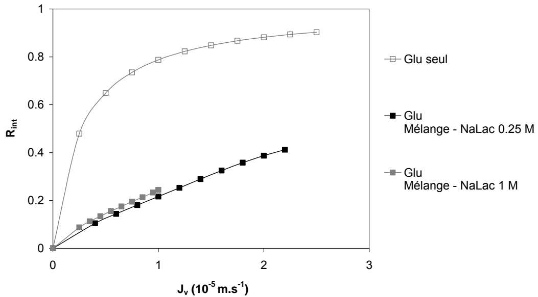
Figure IV-10 . Mélange glucose / lactate de sodium - Rétention intrinsèque du glucose - Influence de la concentration initiale en lactate de sodium - Membranes DK10 - [Glu] = 0.1\text{ M}
