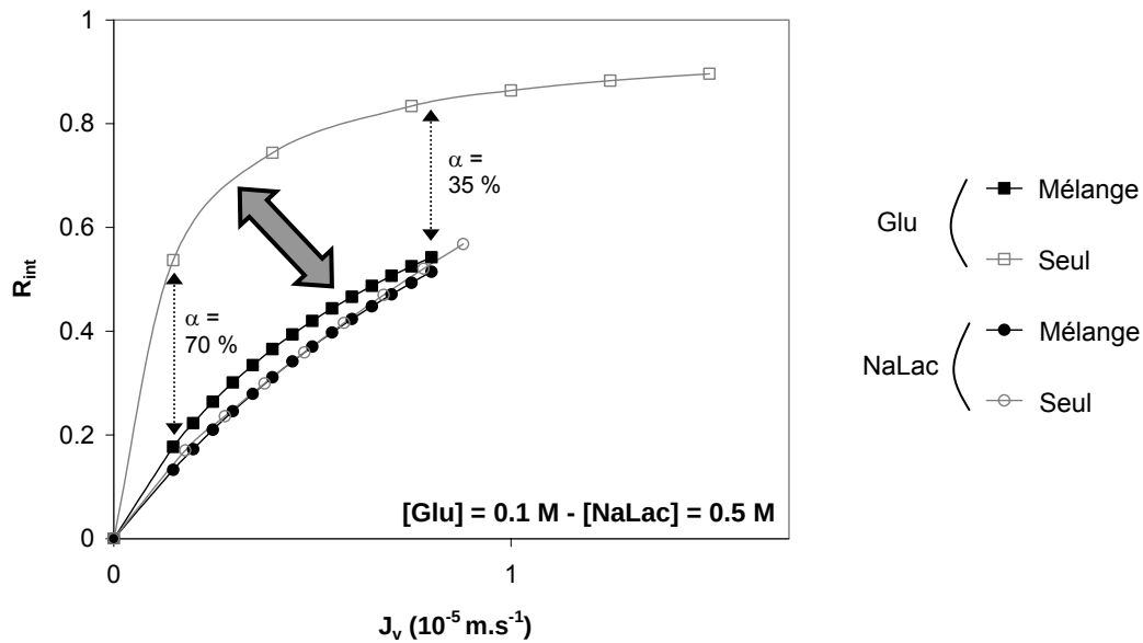
Figure IV-6 . Mélange glucose / lactate de sodium - Rétention intrinsèque - Comparaison avec les rétentions des solutés seuls en solution - Membrane DK15 - [Glu] = 0.1 \text{ M} - [NaLac] = 0.5 \text{ M}
