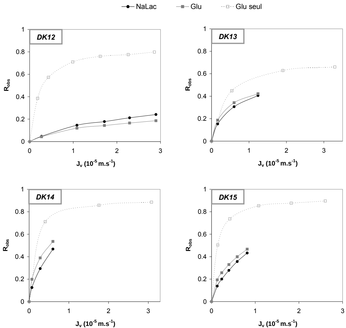
Figure IV-16 . Mélange glucose / lactate de sodium - Rétentions observées - v_t = 1.3 \text{ m.s}^{-1} - [\text{Glu}] = 0.1 \text{ M} - [\text{NaLac}] = 0.5 \text{ M} - Membranes DK12, DK13, DK14 et DK15
