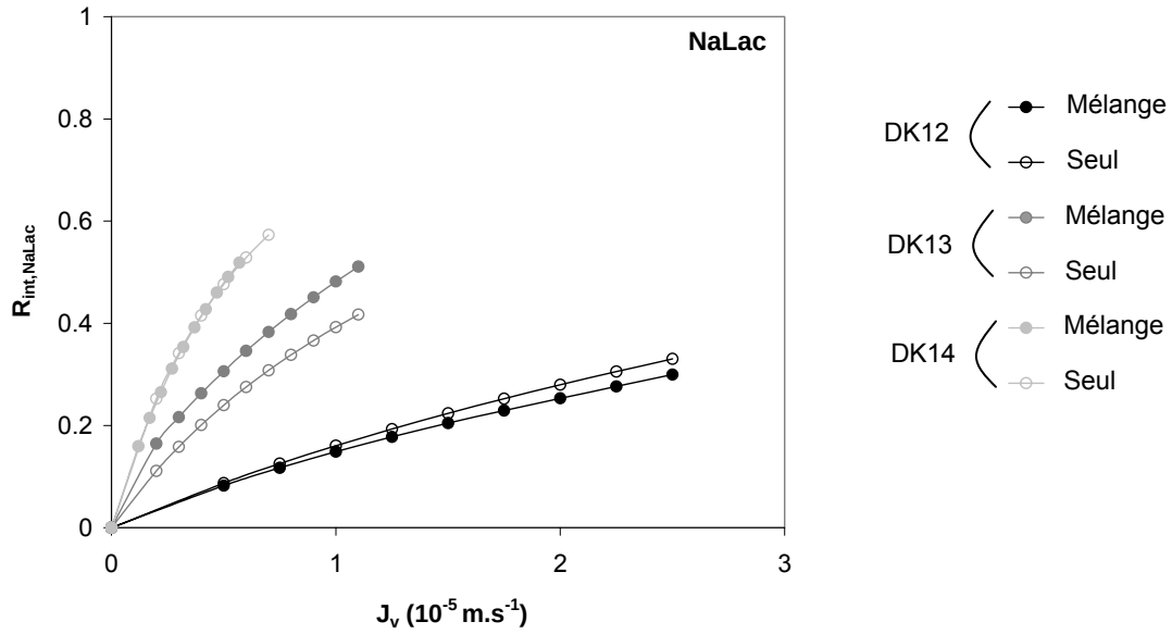
Figure IV-7 . Mélange glucose / lactate de sodium - Rétention intrinsèque du lactate de sodium - Comparaison avec les rétentions du soluté seul en solution - Membranes DK12, DK13, DK14 - [Glu] = 0.1 \text{ M} - [NaLac] = 0.5 \text{ M}
