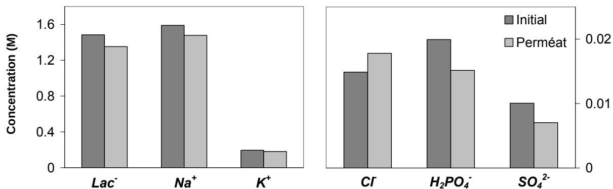
Figure V-8 . Jus n°2 - Composition initiale et après filtration - \Delta P = 20 bar
