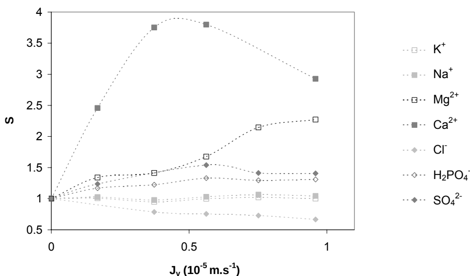
Figure V-10 . Jus n°1 - Facteur de séparation \text{Lac}^- / impurétés
