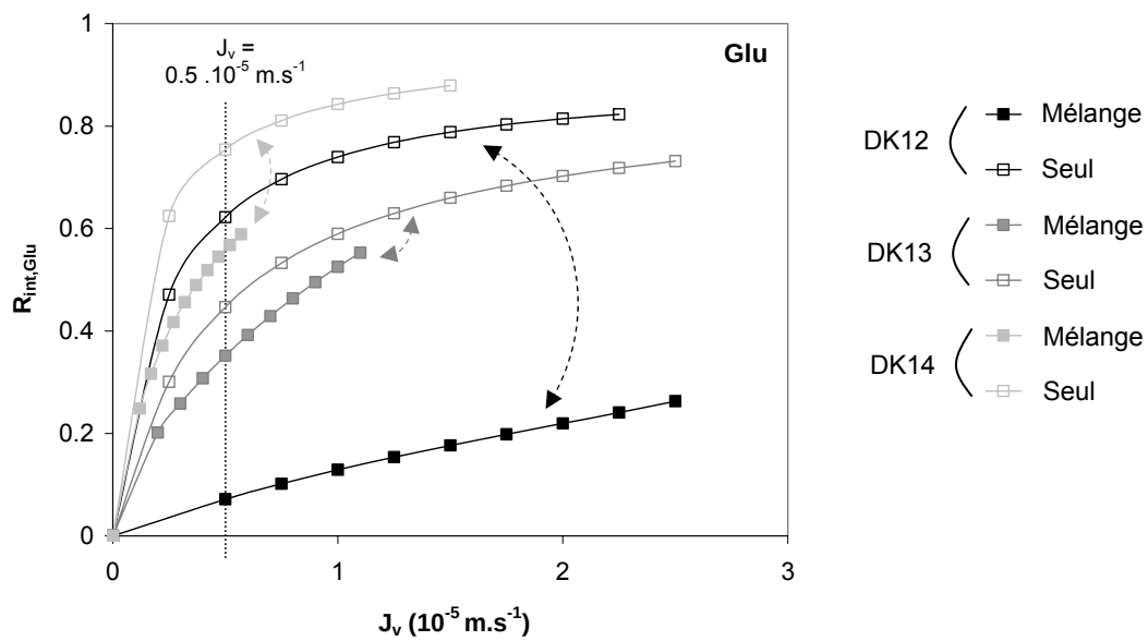
Figure IV-8 . Mélange glucose / lactate de sodium - Rétention intrinsèque du glucose - Comparaison avec les rétentions du soluté seul en solution - Membranes DK12, DK13, DK14 - [Glu] = 0.1 \text{ M} - [NaLac] = 0.5 \text{ M}
