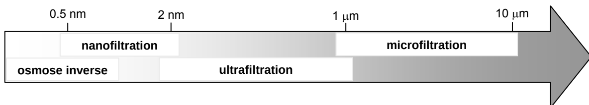
Figure II-1 . Opérations membranaires mettant en oeuvre un gradient de pression - Classement selon la taille moyenne de pores (rayon) des membranes mises en jeu
