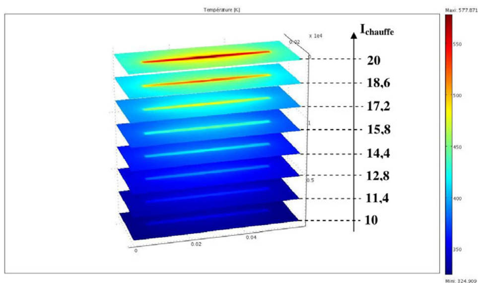
FIGURE 5.7 – Distribution de la température au cours du temps dans un substrat z = 0,2 mm pour une intensité de courant de chauffage comprise entre 10A et 20A et un coefficient d'échange thermique égal à 8W.m^{-2}.K^{-1}
