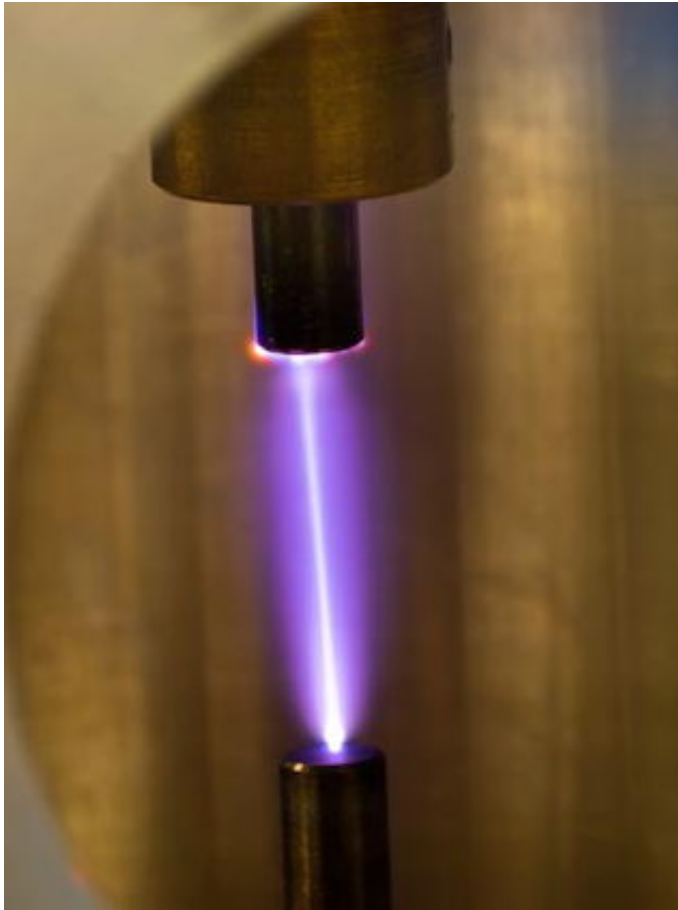
FIGURE 5.17 – Photographie en pause longue d'une transition glow-arc
