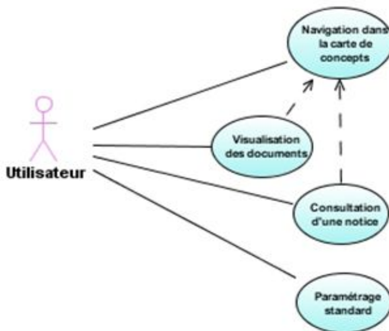
FIGURE 8.5 – Diagramme général des cas d'utilisations
