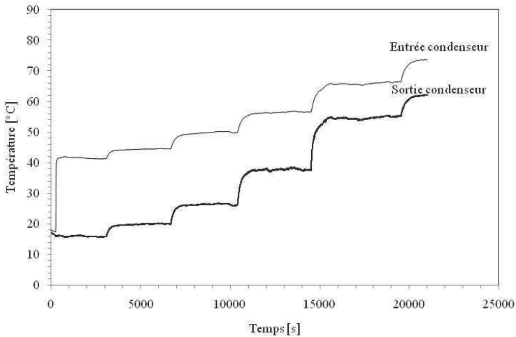
Figure V.14. Evolutions temporelles des températures du n-pentane :(a) évaporateur, (b) condenseur.
