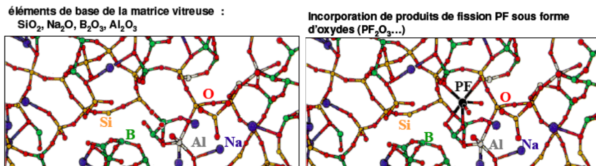
Figure 4 : Principe du confinement de produits de fission dans le verre nucléaire (d'après Godon et al., 04)
