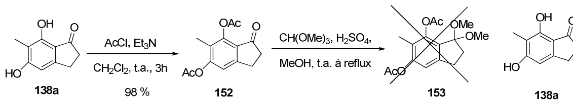
Schéma 124 : essai de protection de la fonction cétone avec les phénols protégés sous forme d'acétate
