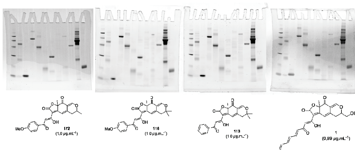
Figure 34 : Comparaison des gels révélés par des analogues de deuxième génération et l'épigallocatechine (excitation à 532 nm).
