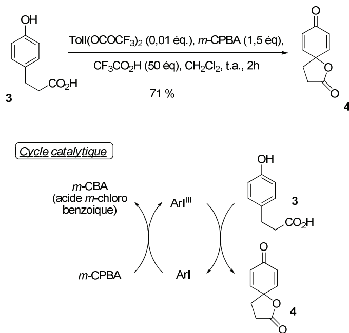
Schéma 8 : Formation de spirocyclohexadiènone en version catalytique
