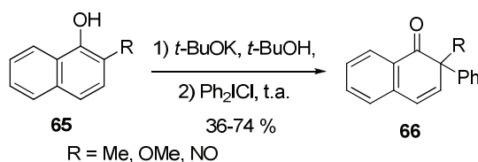
Schéma 27 : désaromatisation oxydante de naphthol par le sel de diphényliodonium
