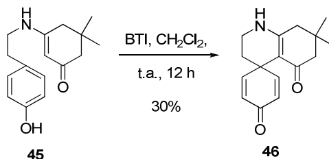
Schéma 18 : synthèse de spirocyclohexadiénone à partir d'un dérivé énamine
