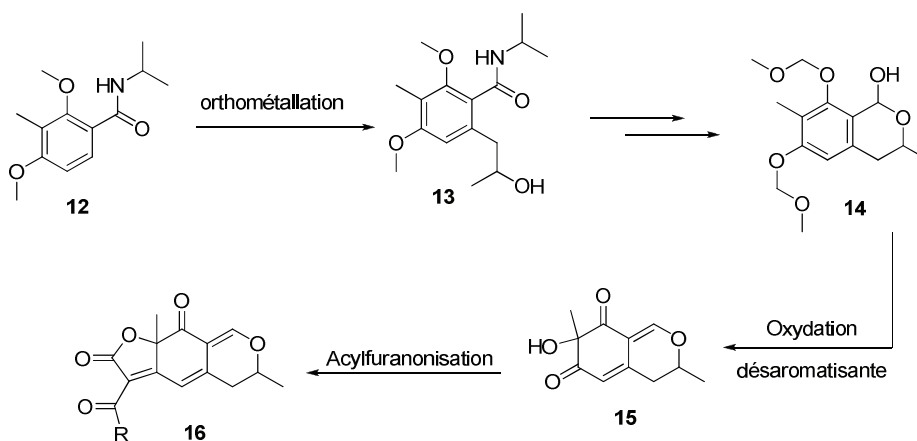
Schéma 52 : voie de synthèse d'analogues de l'épicocconone mise au point au laboratoire
