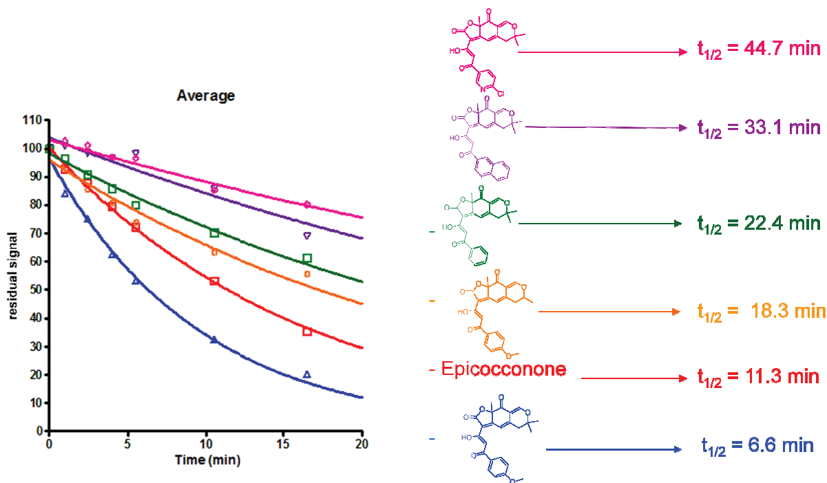
Figure 36 : Evaluation du photoblanchiment des analogues de seconde génération comparés à l'épicocconone
