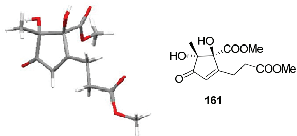
Figure 17 : structure par analyse aux rayons X du composé 161 issu de l'oxydation désaromatisante dans le méthanol
