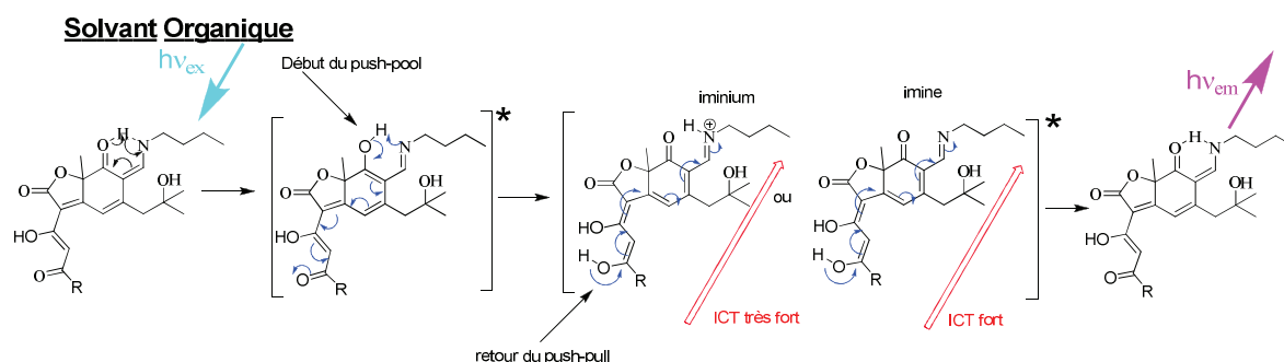
Schéma 143 : Push-pull constant entre les deux équilibres cétoénolique et cétoénaminique dans le \text{CH}_3\text{CN}
