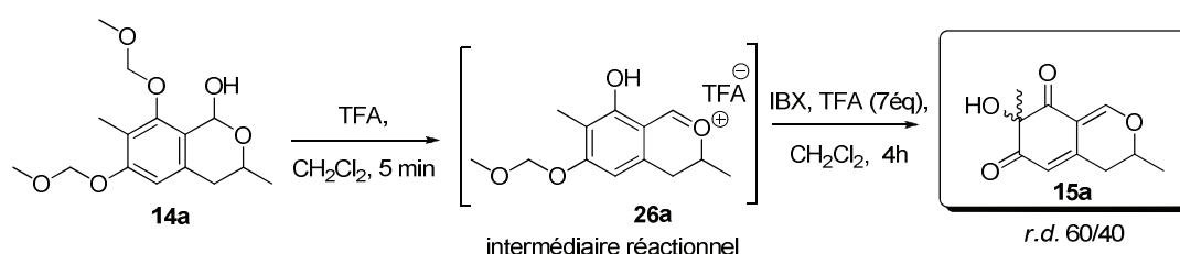
Schéma 65 : Obtention d'un mélange de diastéréoisomères lors de la réaction d'oxydation désaromatisante
