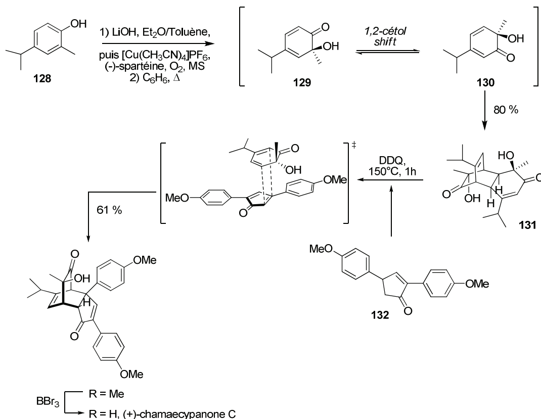
Schéma 48 : Synthèse du (+)-chamaecypanone C de Porco
