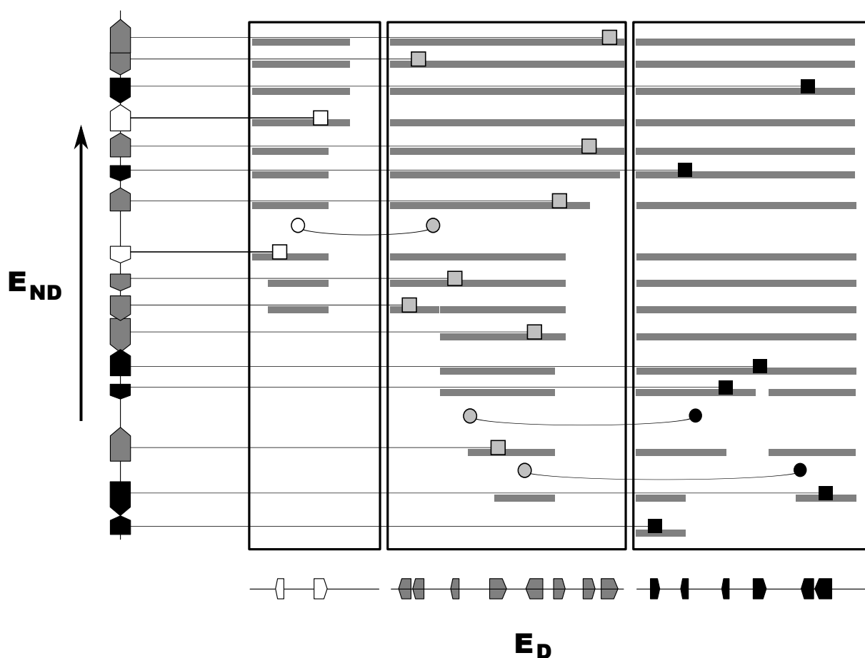
Figure 8.1. Extraction d'un bloc de synténie double-conservée. Le chromosome du génome non dupliqué est représenté verticalement à gauche, et les chromosomes du génome dupliqué sont disposés horizontalement. Un carré représente des gènes orthologues, les cercles représentent des gènes ohnologues. On parcourt les gènes du génome non dupliqué de bas en haut : à chaque nouveau gène, on étend le bloc si le ou les orthologues du gène se trouvent (i) sur le même chromosome que celui du gène précédent, (ii) dans le voisinage d'un gène déjà inclus (régions autorisées : zones grises), (iii) dans le voisinage d'un ohnologue d'un gène dans une région autorisée. Dans cet exemple, le 2 ème gène est ajouté au bloc car son orthologue est sur le même chromosome que celui du 1 er gène. Le 3 ème gène est rajouté car son orthologue est dans le voisinage de l'ohnologue d'un gène qui lui-même se trouve dans le voisinage du 2 ème gène. Figure tirée de (Muffato 2010).
