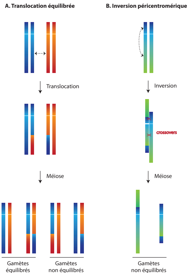
Figure 3.6. Conséquences de deux réarrangements équilibrés (A : translocation, B : inversion péricentrique) sur les gamètes produits à la méiose. Dans les deux cas, une partie des gamètes au moins est non équilibrée.
