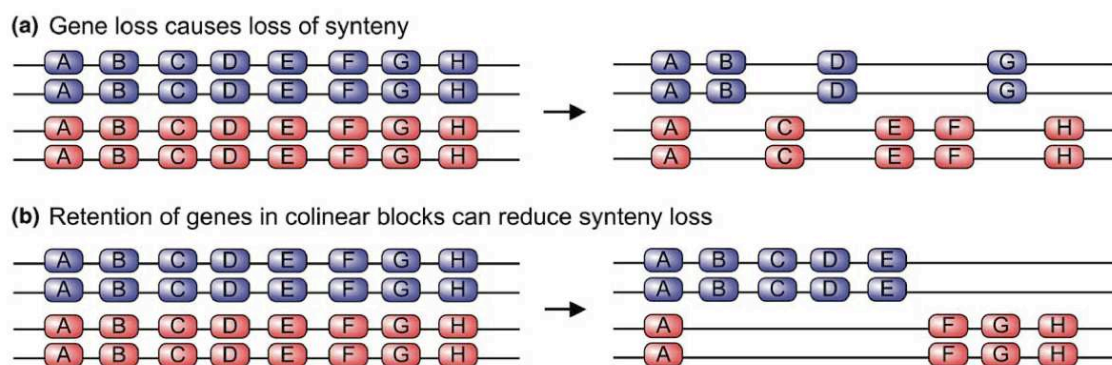
Figure 4.7. Perte de la synténie conservée au sens strict causée par la rediploidisation qui suit une duplication complète. La perte de gènes par délétions de larges blocs peut limiter la perte de synténie. Figure tirée de (Hufton and Panopoulou 2009).
