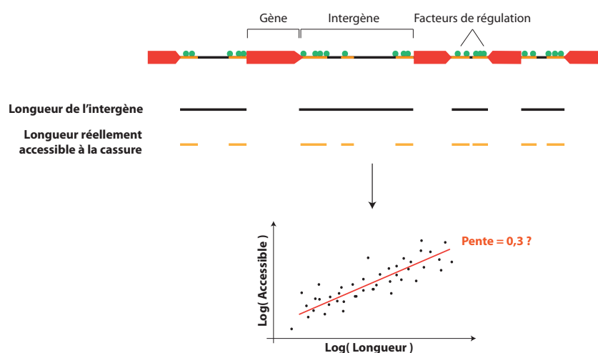
Figure 19.1. Proposition de modèle liant fixation de facteurs de régulation, ouverture de la chromatine et probabilité de cassure.
