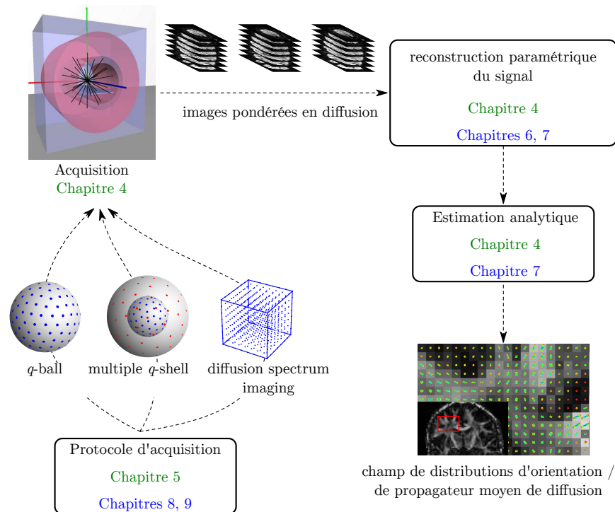
Figure 2.1: Schéma des différentes étapes en IRM de diffusion, depuis la préparation de la séquence d'acquisition à la reconstruction des informations locales de diffusion. Les chapitres qui traitent plus particulièrement chacune de ces étapes sont indiqués ; en vert, les chapitres d'état de l'art, et en bleu, les contributions.
