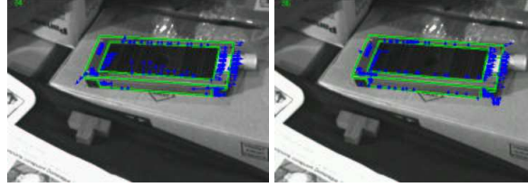
FIG. 5.4: Calcul des déplacements normaux aux contours pour deux images successives
