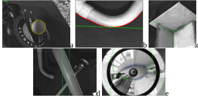
FIG. 5.3: Suivi de primitives 2D simples reposant sur la méthode des ECM dans des expérimentations utilisant l'asservissement visuel (a) reconstruction d'une sphère par vision dynamique active [31], (b) suivi de contour [126], (c) suivi d'un trièdre [4], (d) positionnement par rapport à un cylindre avec évitement des butées [32], (e) suivi de "droites" prenant la forme de cercles dans des images catadioptriques (projet ROBEA OMNIBOT [149])
