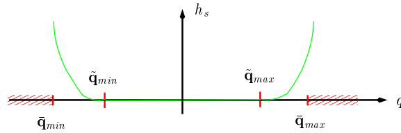
FIG. 3.5: Évitement des butées articulaires par une approche classique de projection de gradient : évolution de la fonction de coût h_s en fonction de la position articulaire.
