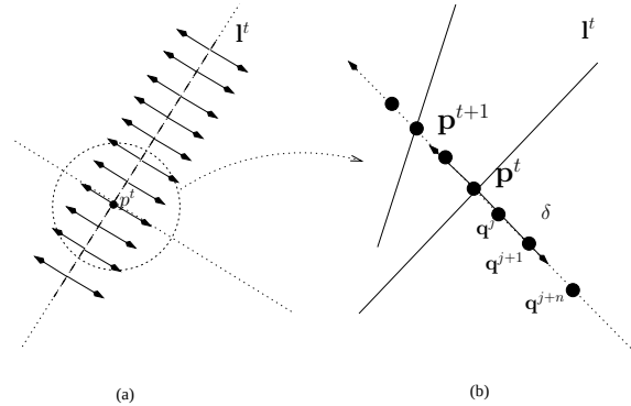
FIG. 5.2: Principe de l'algorithme des ECM pour la mise en correspondance de points de contour (a) calcul de la normale le long d'un contour, (b) recherche du correspondant le long de la normale.
