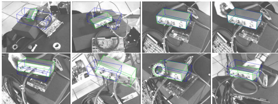
FIG. 5.10: Suivi d'un objet pendant une expérience d'asservissement visuel 2D 1/2. L'objet suivi est en vert et sa position désirée dans l'image est en bleu. Les images de la première ligne correspondent à l'étape initiale de positionnement. Dans la suivante, à la fois l'objet et le robot sont en mouvement.
