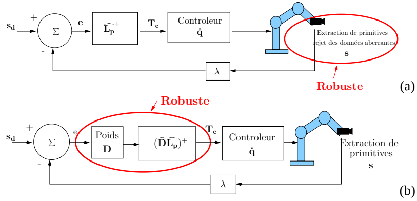
FIG. 3.12: (a) Asservissement visuel robuste "classique" : le rejet des données aberrantes se fait dans l'extraction des données, (b) Nouvelle loi de commande : le rejet des données aberrantes se fait dans la loi de commande.
