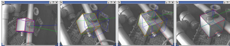
FIG. 5.9: Suivi d'un objet pendant une expérience d'asservissement visuel 2D 1/2. L'objet suivi est en vert et sa position désirée dans l'image est en bleu. Les points rouges correspondent aux points suivis par l'algorithme des ECM
