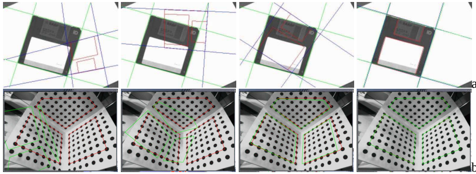
FIG. 5.6: Pose et calibration par asservissement visuel virtuel: principe. L'objectif est de modifier itérativement la position de la caméra en utilisant une loi de commande classique d'asservissement visuel afin de recaler les primitives visuelles extraites de l'image avec les primitives calculées par projection du modèle 3D. Sur la première ligne, des droites sont utilisées pour calculer la pose. Sur la seconde ligne des points sont utilisés pour calculer à la fois la pose et les paramètres intrinsèques de la caméra.
