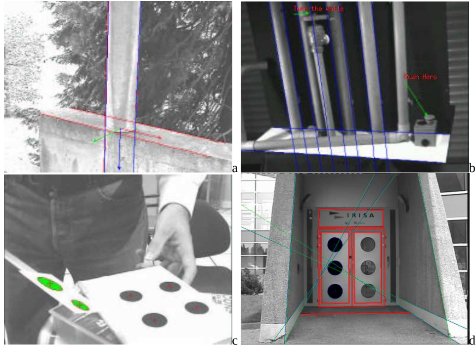
FIG. 5.7: Calcul de pose réalisé à partir de plusieurs primitives de nature différente (a-b) droite et cylindre (c) cercle et points (d) cercles et droites
