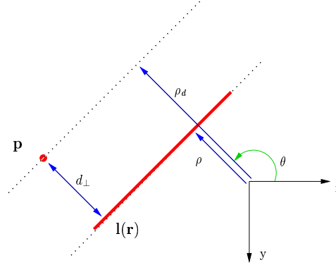
FIG. 5.8: Une des primitives visuelles utilisées dans le processus de suivi : distance d'un point à une droite
