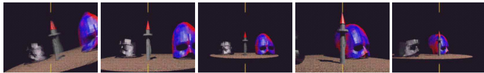
FIG. 4.2: Positionnement et suivi d'une trajectoire prédéfinie. L'animateur a spécifié une tâche de focalisation sur la tour (contraignant deux degrés de liberté). La caméra suit ensuite une trajectoire spécifiée par une spline 3D en utilisant une tâche secondaire (la distance entre le centre optique de la caméra et un point évoluant sur la courbe doit être minimale).
