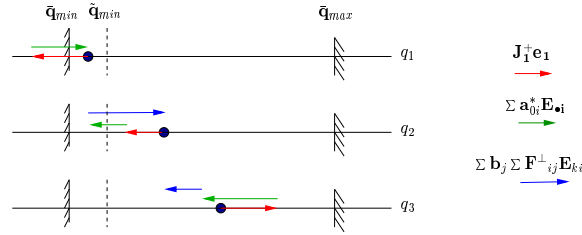
FIG. 3.8: Nouvel algorithme dans sa version itérative : aucun mouvement n’est autorisé pour les axes en zone critique et pour ceux susceptible d’y entrer. Si une solution existe au problème d’évitement de butée (i.e., si il y a des degrés de liberté disponibles), elle sera trouvée.
