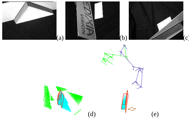
FIG. 3.3: Résultat d'un processus d'exploration globale par calcul de point de vue : (a) première image acquise par le système, (b) image de la même scène acquise pendant l'exploration (de nouvelles primitives apparaissent), (c) reconstruction et zones inconnues après la première reconstruction incrémentale, (d) zones connues et inconnues avant le début du processus d'exploration, (e) différents points de vue calculés pendant l'exploration (il ne reste plus de zones inconnues)
