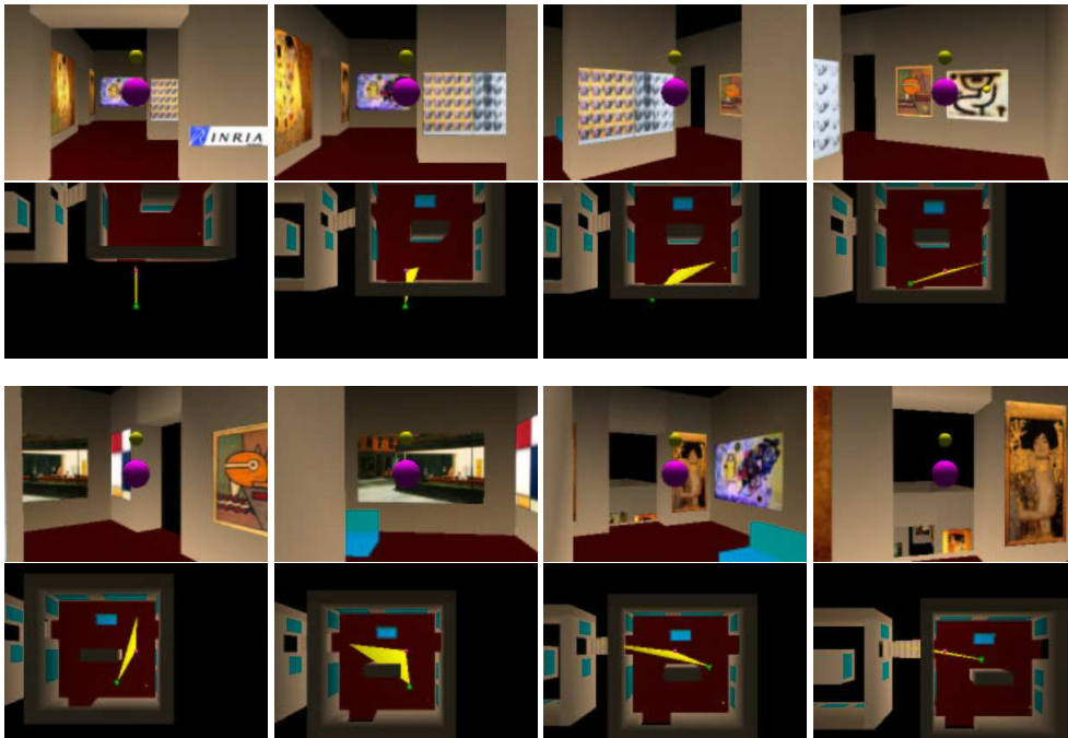
FIG. 4.3: Traversée d'un musée par une caméra poursuivant une cible. La tâche principale de la caméra est de rester focalisée sur sa cible (les deux sphères violette et jaune). Deux tâches secondaires sont par ailleurs considérées, spécifiant d'une part à la caméra de ne pas heurter un obstacle (ici les murs du musée) et d'autre part de toujours éviter l'occultation de la cible par des éléments du décor. Les première et troisième lignes montrent la vue de la caméra. Les secondes et quatrième lignes montrent une vue du dessus. Les volumes jaunes visibles sur ces vues du dessus sont utilisés pour prédire le risque d'occultation en extrapolant les positions futures de la cible. Les résultats de la même expérience dans le cas où aucune tâche secondaire n'est considérée sont présentées dans [138].
