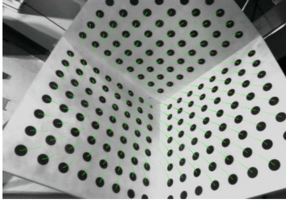
FIG. 5.11: Calibration d'un objectif de 6mm par asservissement visuel virtuel. La position des points en vert correspond à la reprojection des points du modèle 3D pour les paramètres de calibration estimés.
