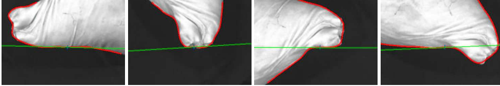
FIG. 2.3: Utilisation de la redondance pour une tâche de suivi de contour. La tâche principale impose que la tangente à la courbe extraite de l'image soit horizontale dans l'image (ce qui contraint 2 degrés de liberté), la tâche secondaire impose un mouvement dans la direction de l'axe des x du repère de la caméra.
