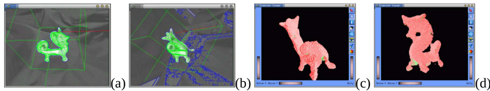
FIG. 3.4: Reconstruction d'un objet 3D par des techniques de coloration de voxels et exploration par asservissement visuel. (a-b) images acquises depuis positions différentes de la caméra avec projection du modèle reconstruit (c-d) deux vues du modèle final.
