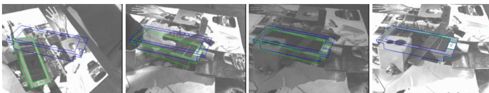
FIG. 2.1: Suivi d'un objet pendant une expérience d'asservissement visuel 2D. L'objet suivi est en vert et sa position désirée dans l'image est en bleu.
