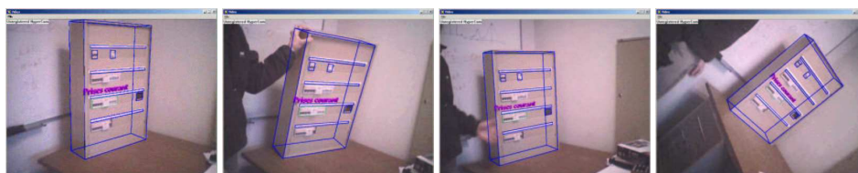
FIG. 5.17: Markerless : suivi d'une armoire électrique, occultations et mouvements importants
