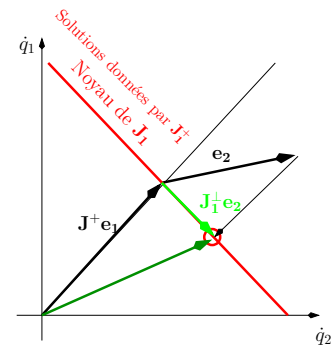
Fig 2.2-b : Dans le cas où une tâche secondaire e_2 est considérée, elle est projetée sur le noyau J_1^\perp de la tâche et n'a donc aucun effet sur la tâche principale.
