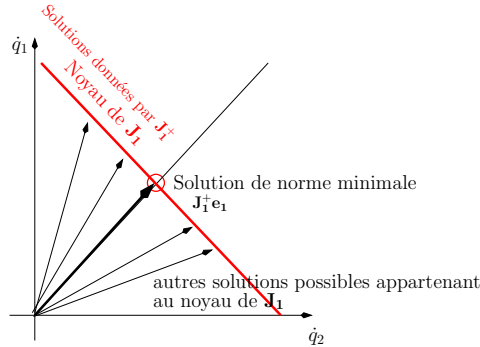
Fig 2.2-a : Il existe a priori une infinité de solutions aux problèmes, toutes situées sur le noyau J_1^\perp de J_1 . La pseudo-inverse J_1^+ de J_1 fournit la solution de norme minimale.
