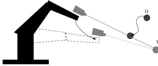
FIG. 3.10: Exemple d’une contrainte exprimée dans l’image : l’évitement d’occultations. La caméra doit rester focalisée sur l’objet T en évitant les occultations potentielles provoquées par O
