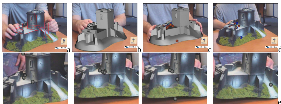
FIG. 5.18: Markerless : suivi d'un château fort, le mouvement des billes incrustées est géré par un moteur physique d'animation intégré dans le logiciel D'Fusion de Total-Immersion. Les images de la première ligne montrent (de droite à gauche) l'objet suivi avec les arêtes saillantes du modèle 3D superposées (a), le modèle 3D complet (b), l'ajout de billes soumises à la gravité et gérées par un moteur physique d'animation (c-d). La seconde ligne (e) correspond à quatre images extraites de la vidéo.
