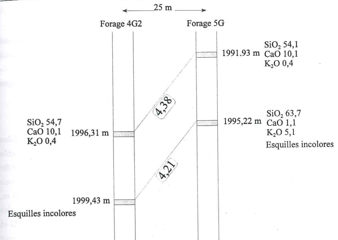
Figure 3-33 : Schématisation du décalage des profondeurs des couches de cendres (en grisé) entre les forages 4G2 et 5G (espacés de 25 m), entre 1990 et 2000 m. Les compositions des couches Si, Ca et K sont données en % poids d'oxyde. Le décalage entre les deux forages est de 4,38 m pour la couche supérieure et 4,21 m pour la couche inférieure.
