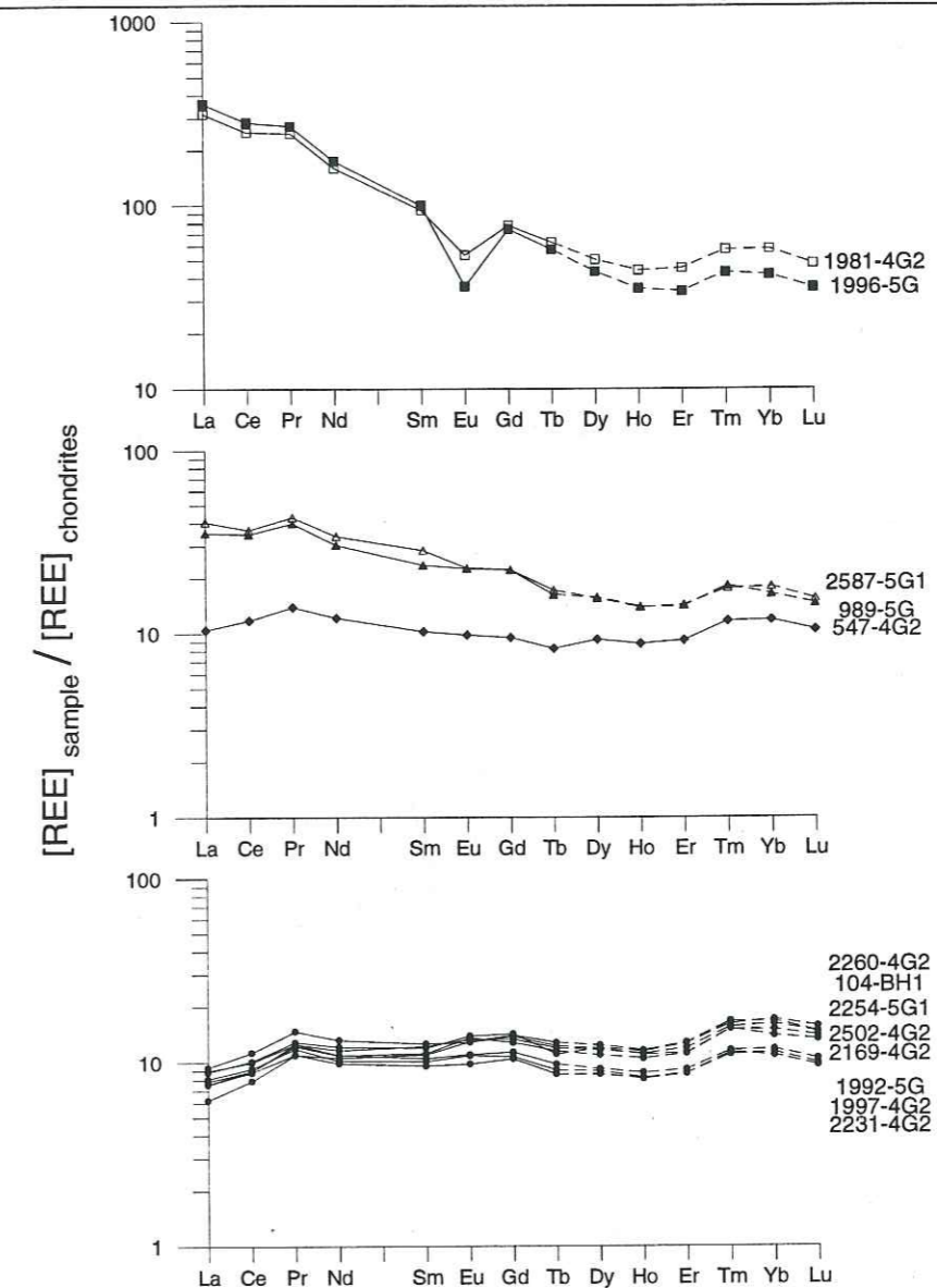
Figure 3-12 : Profil en REE normalisé aux chondrites : traits pleins : valeurs mesurées ; traits pointillés : valeurs corrigées pour les niveaux mesurés en février 1995.
