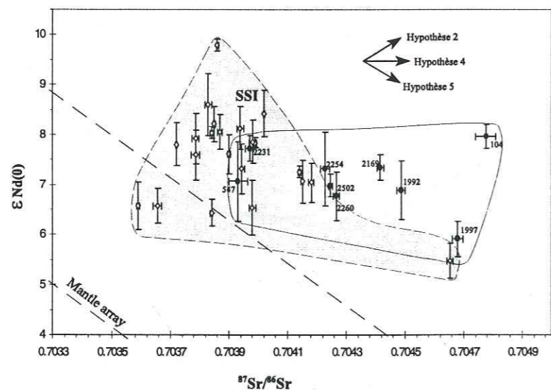
Figure 3-32 : comparaison des signature isotopique \epsilon \text{Nd} (0) versus ^{87}\text{Sr}/^{86}\text{Sr} entre les SSI (Pearce et al., 1995) et les cendres provenant des SSI. Les flèches indiquent la direction de la dérive entraînée (lorsqu'il peut être proposé à priori) selon les différentes hypothèses discutées dans le texte.
