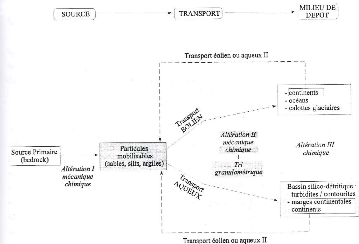
Figure 4-20 : Schéma du cycle formation / transport / sédimentation du matériel détritique issu de l'érosion des continents. Altération I : primaire ; II : secondaire ; III : tertiaire. Les étapes en grisé représentent les problématiques directes de notre étude.
