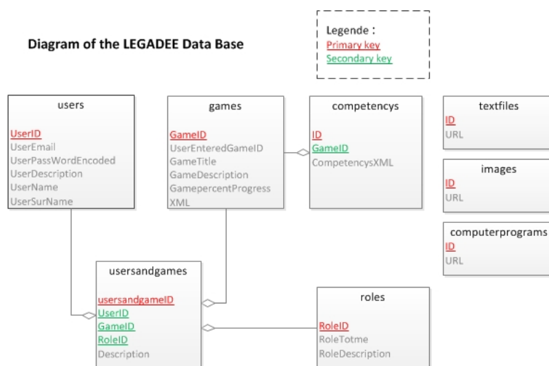
Fig 3 : Diagramme de la base de données
